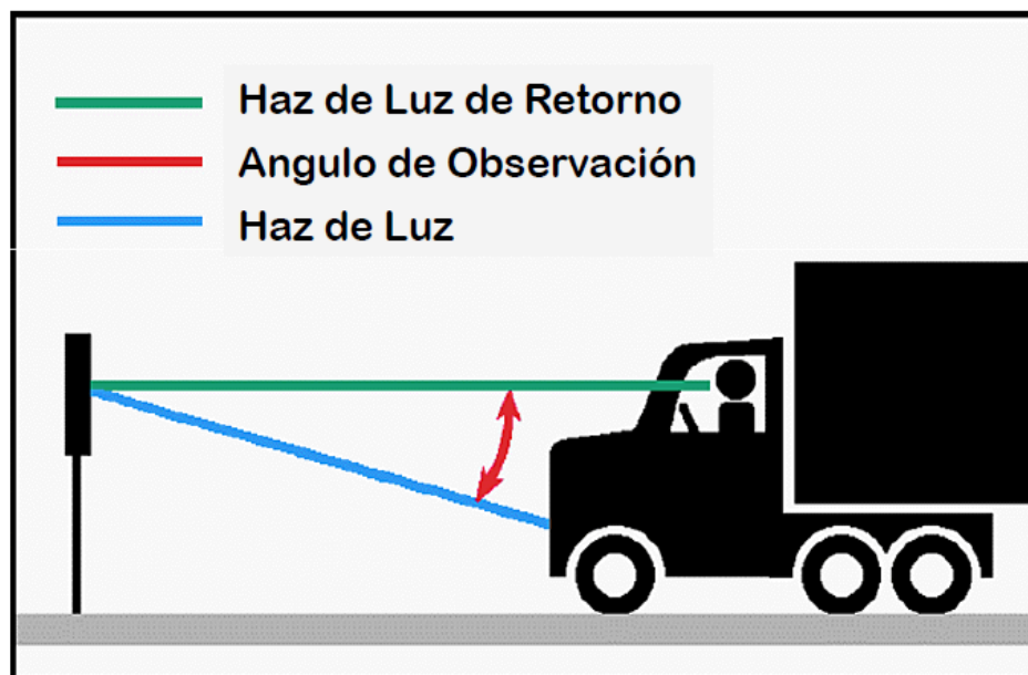
Figura 3.10. Ángulo de Observación. Fuente:(Barreno, 2014)
