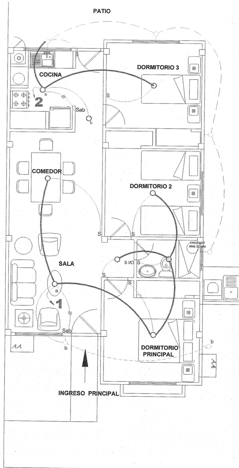
Figura 100. Circuito # 2, de Alumbrado.
