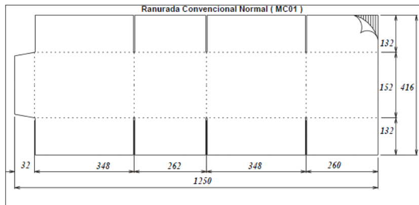
FIGURA 2. 9 MC01 CAJA RANURADA CONVENCIONAL NORMAL
