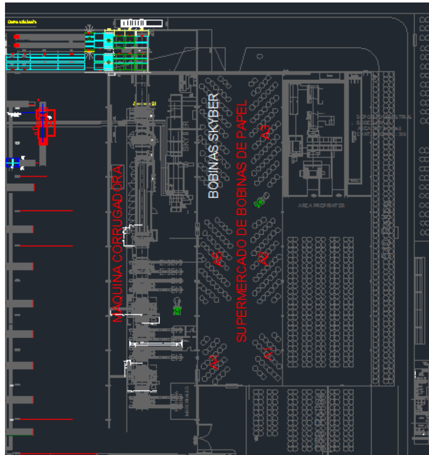
FIGURA 4. 9 SUPERMERCADO DE BOBINAS DE PAPEL
