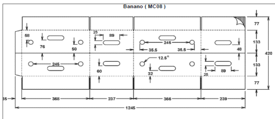
FIGURA 2. 16 MC08 TAPA DE BANANO
