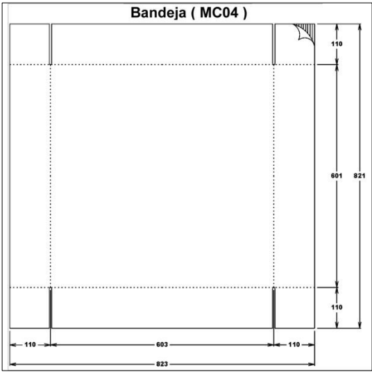
FIGURA 2. 12 MC04 CAJA TIPO BANDEJA
