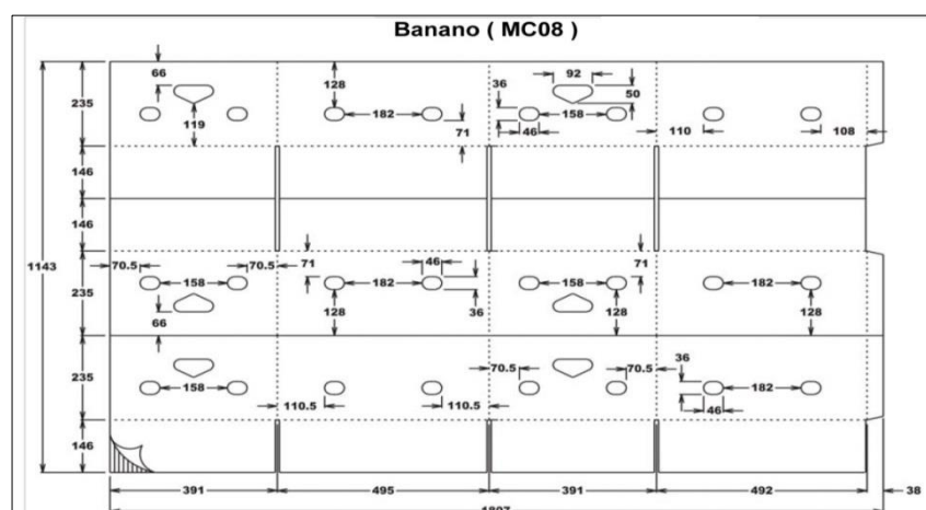
FIGURA 2. 17 MC08 FONDO DE BANANO
