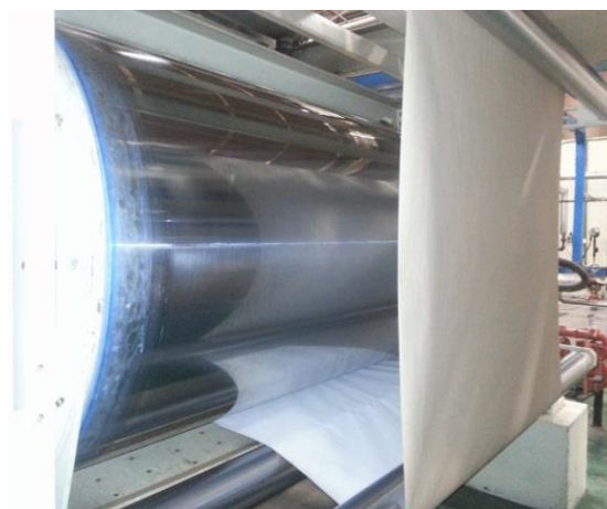
FIGURA 2. 42 PRE-CALENTADOR
