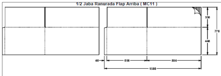
FIGURA 2. 18 MC11 ½ JABA RANURADA FLAP ARRIBA
