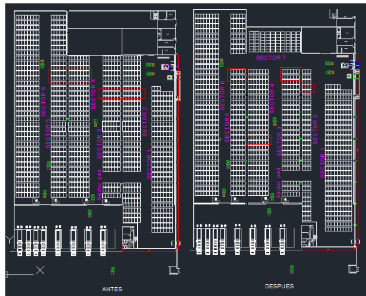
FIGURA 4. 29 MODIFICACIÓN DE LAYOUT ANTES Y DESPUÉS
