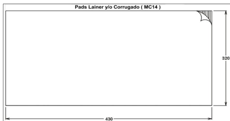
FIGURA 2. 21 MC14 PADS Y/O CORRUGADO
