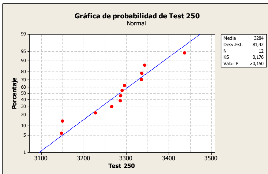
FIGURA 4.5 PRUEBA DE NORMALIDAD TEST 250
