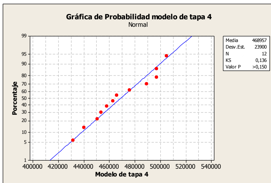
FIGURA 4. 22 PRUEBA DE NORMALIDAD MODELO DE TAPA 4
