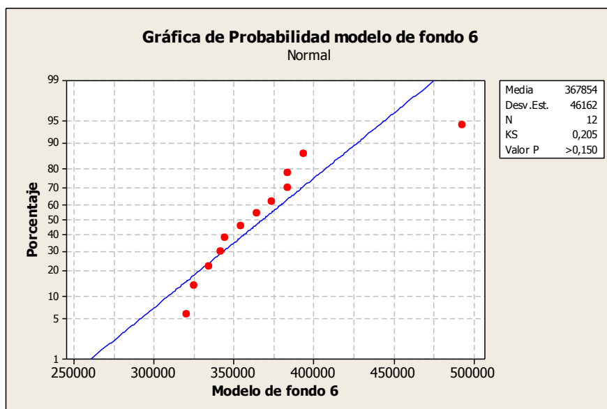
FIGURA 4. 25 PRUEBA DE NORMALIDAD MODELO DE FONDO 6
