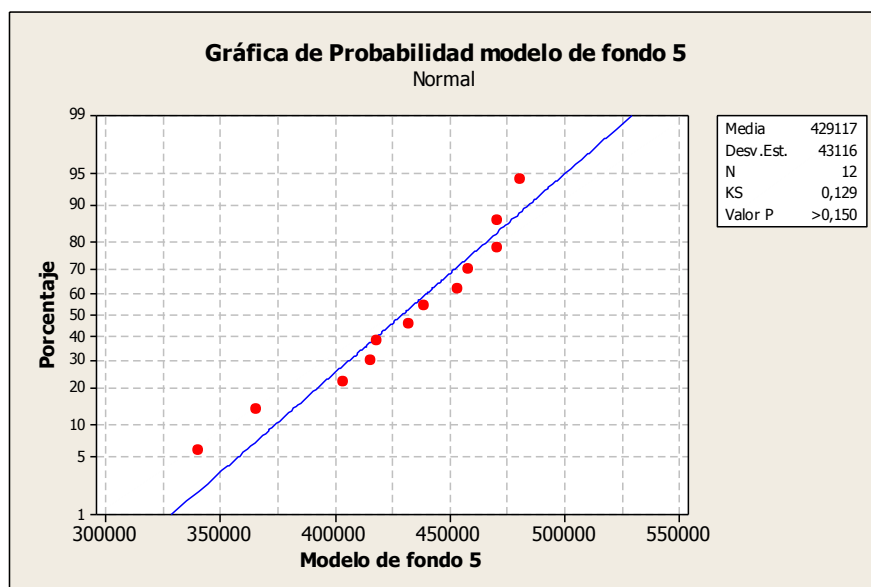
FIGURA 4. 23 PRUEBA DE NORMALIDAD MODELO DE FONDO 5
