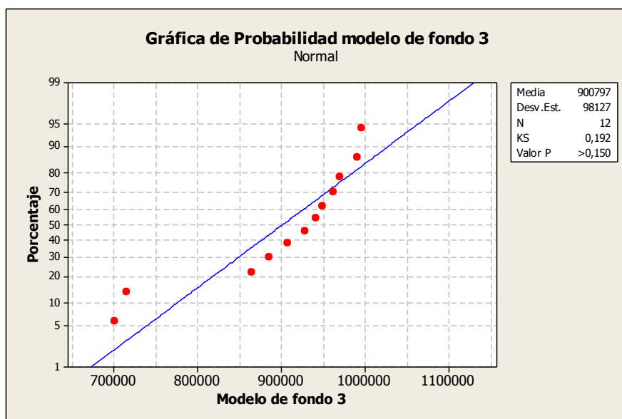
FIGURA 4. 18 PRUEBA DE NORMALIDAD MODELO DE FONDO 3
