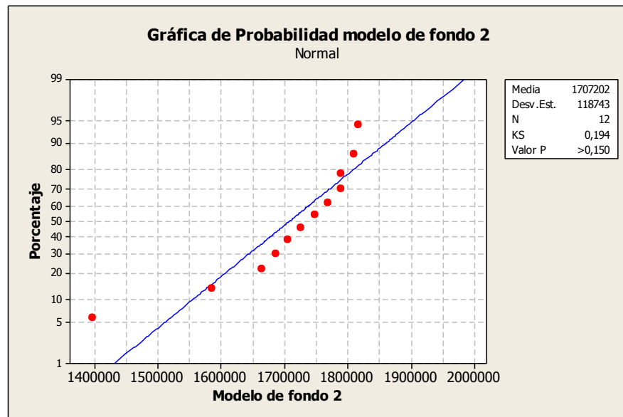
FIGURA 4. 16 PRUEBA DE NORMALIDAD MODELO DE FONDO 2
