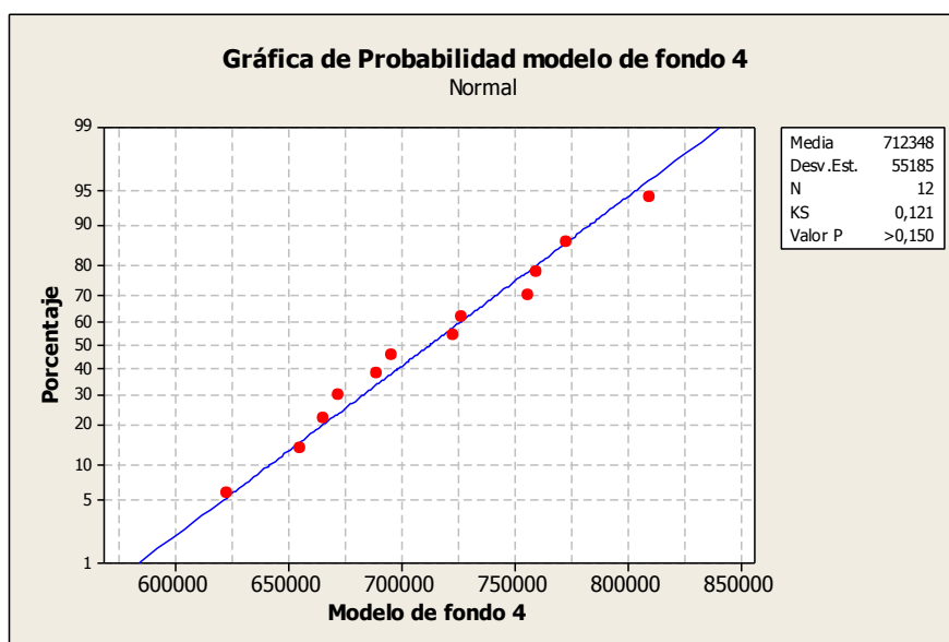
FIGURA 4. 20 PRUEBA DE NORMALIDAD MODELO DE FONDO 4
