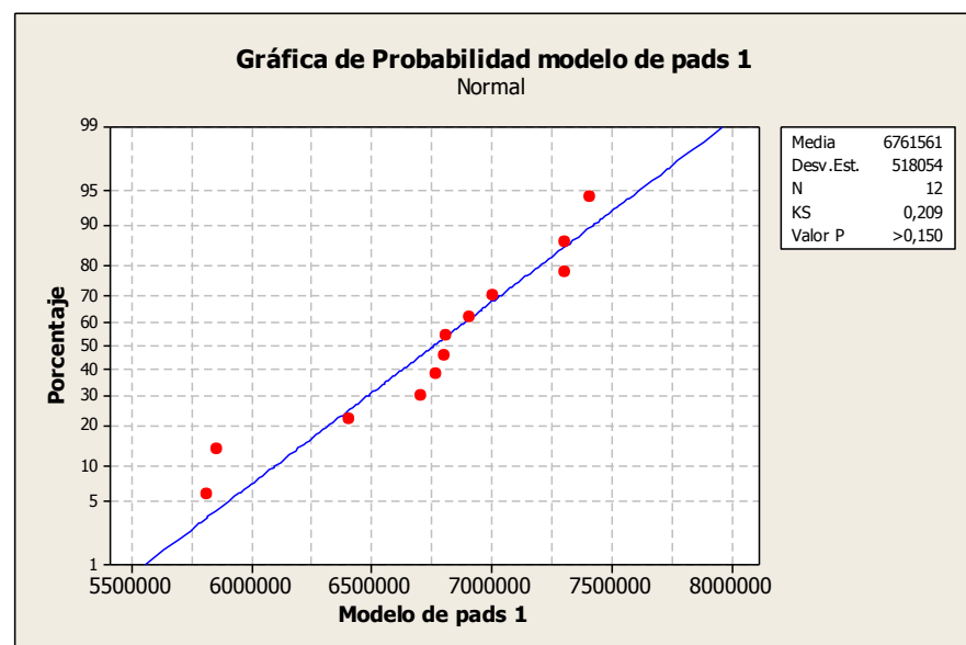
FIGURA 4. 13 PRUEBA DE NORMALIDAD MODELO DE PADS 1
