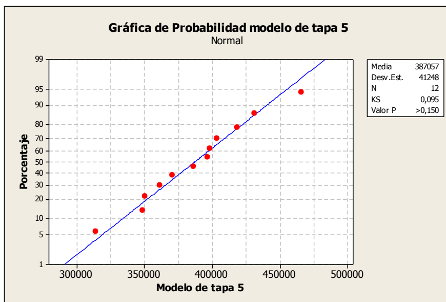
FIGURA 4. 24 PRUEBA DE NORMALIDAD MODELO DE TAPA 5
