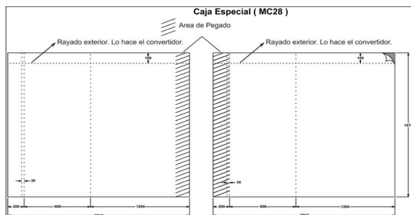
FIGURA 2. 34 MC289 CAJA ESPECIAL
