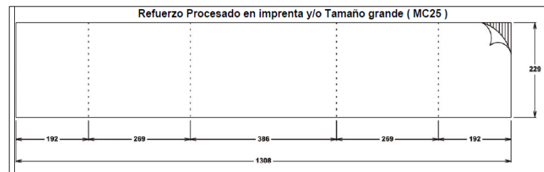
FIGURA 2. 32 MC25 REFUERZO PROCESADO EN IMPRENTA Y/O TAMAÑO GRANDE
