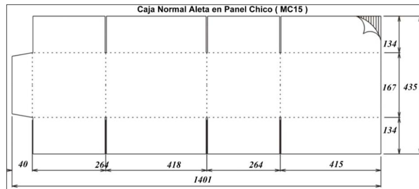
FIGURA 2. 22 MC15 CAJA NORMAL ALETA PANEL CHICO
