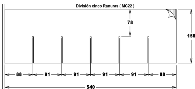
FIGURA 2. 30 MC22 DIVISIÓN CINCO RANURAS
