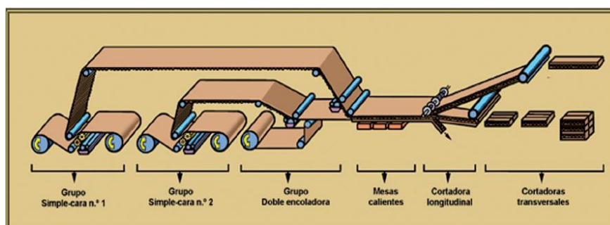
FIGURA 2. 39 OPERACIONES DE LA MÁQUINA ONDULADORA
