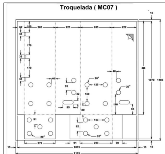
FIGURA 2. 15 MC07 CAJA TROQUELADA
