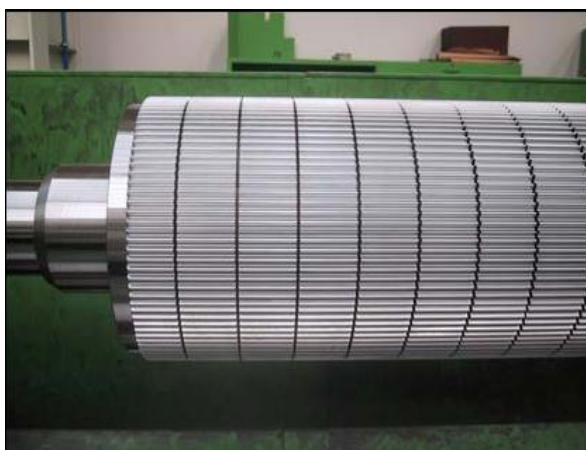
FIGURA 2. 43 RODILLO ONDULADOR
