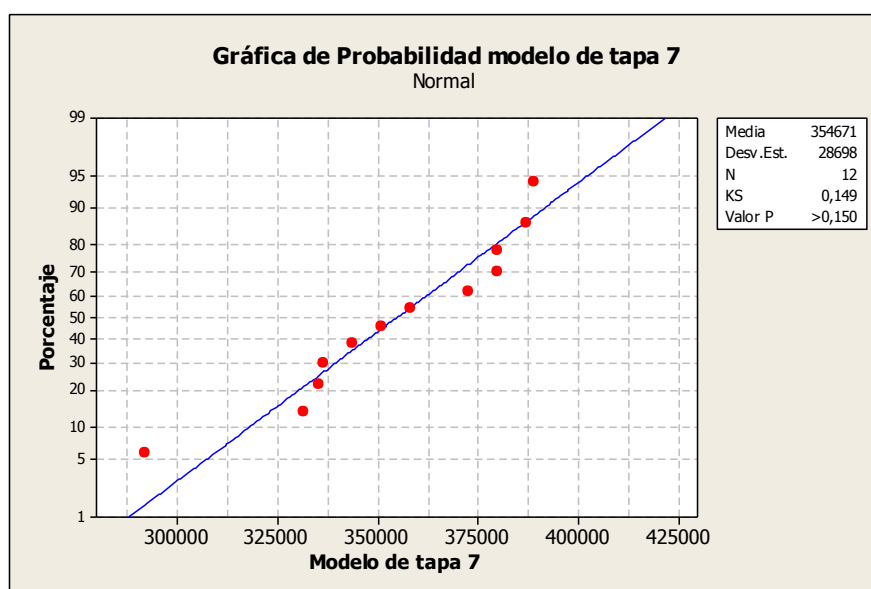
FIGURA 4. 27 PRUEBA DE NORMALIDAD MODELO DE TAPA 7
