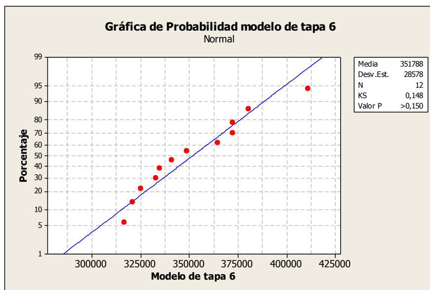
FIGURA 4. 26 PRUEBA DE NORMALIDAD MODELO DE TAPA 6
