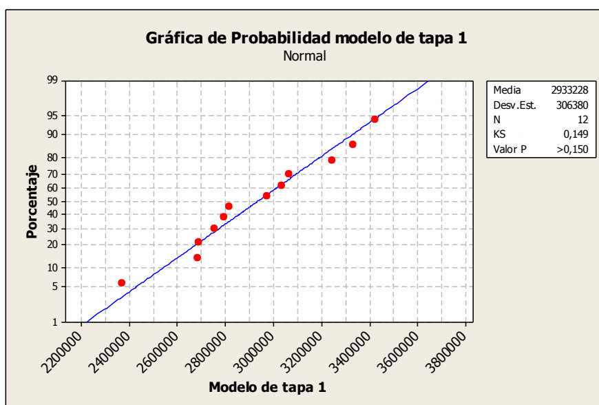
FIGURA 4. 15 PRUEBA DE NORMALIDAD MODELO DE TAPA 1
