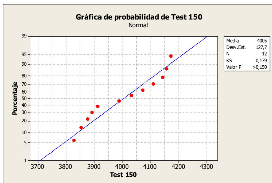
FIGURA 4. 4 PRUEBA DE NORMALIDAD TEST 150
