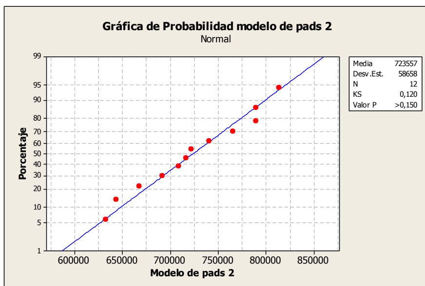
FIGURA 4. 19 PRUEBA DE NORMALIDAD MODELO DE PADS 2
