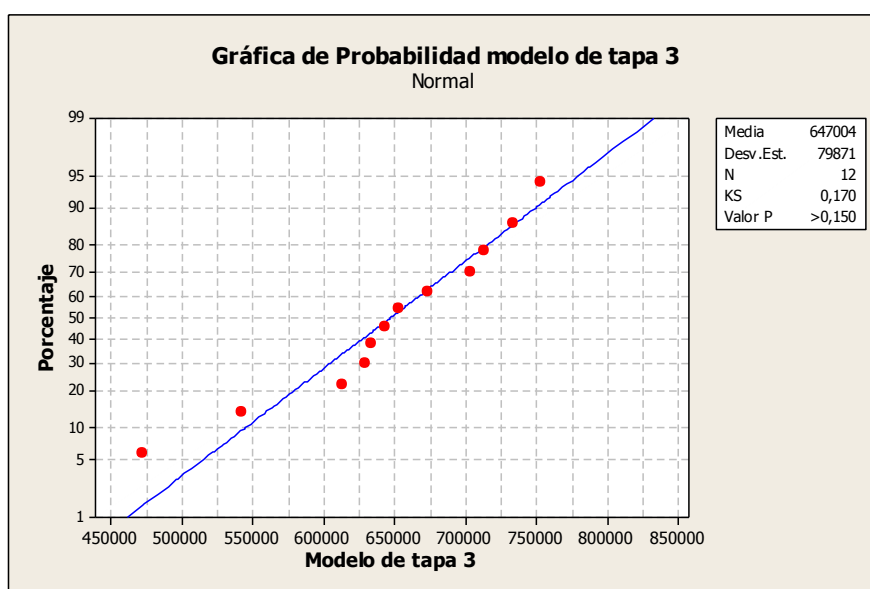
FIGURA 4. 21 PRUEBA DE NORMALIDAD MODELO DE TAPA 3
