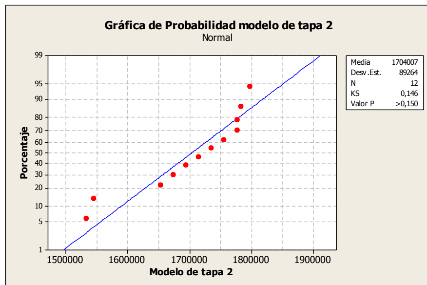
FIGURA 4. 17 PRUEBA DE NORMALIDAD MODELO DE TAPA 2
