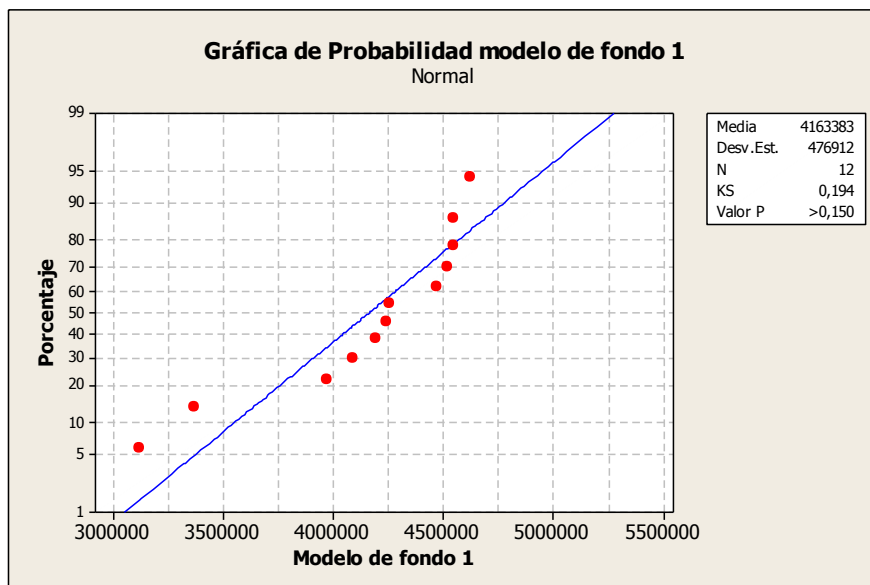
FIGURA 4. 14 PRUEBA DE NORMALIDAD MODELO DE FONDO 1
