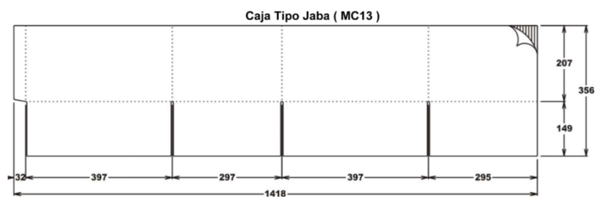
FIGURA 2. 20 MC13 CAJA TIPO JABA
