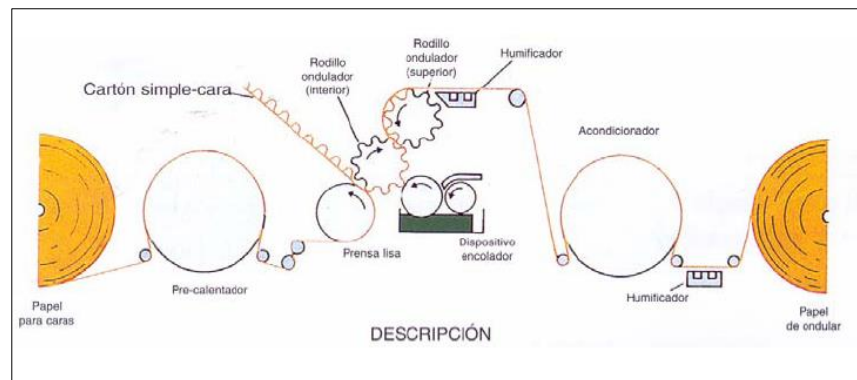
FIGURA 2. 40 OPERACIONES PARA ELABORAR SIMPLE CARA
