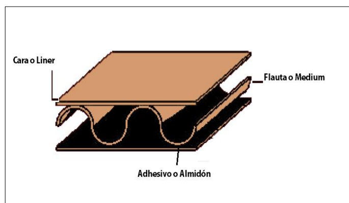
FIGURA 2. 1 PARTES DEL CARTÓN ONDULADO
