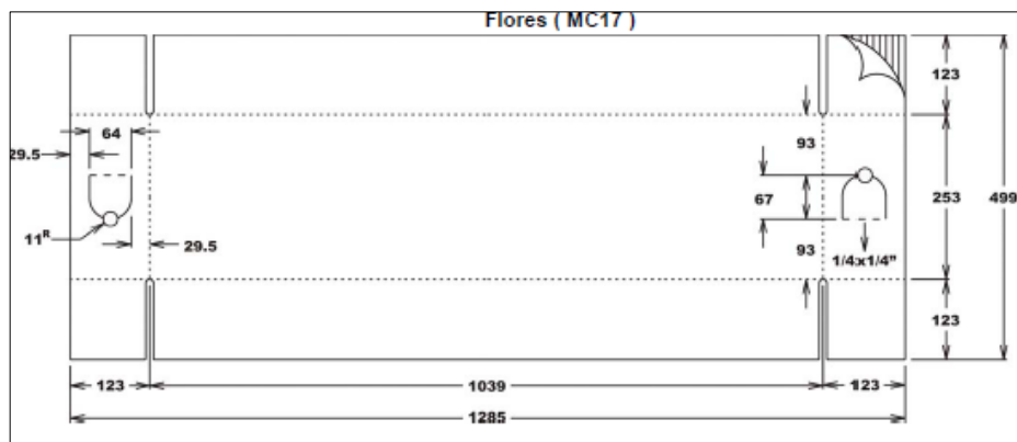
FIGURA 2. 23 MC17 TAPA DE FLORES
