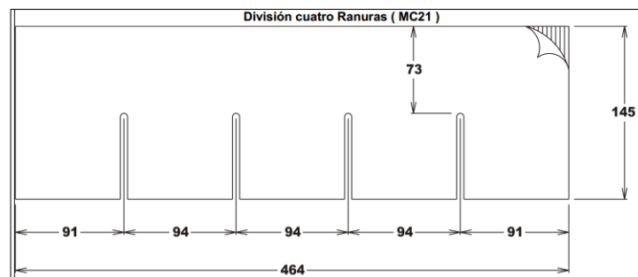
FIGURA 2. 29 MC21 DIVISIÓN CUATRO RANURAS
