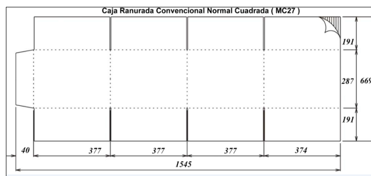
FIGURA 2. 33 MC27 CAJA RANURADA CONVENCIONAL NORMAL CUADRADA
