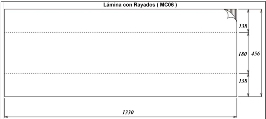
FIGURA 2. 14 MC06 LÁMINA CON RAYADOS
