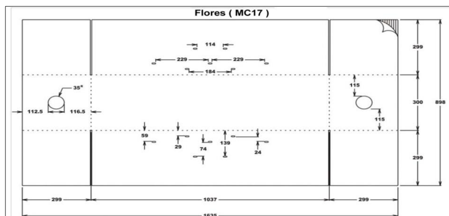
FIGURA 2. 24 MC17 FONDO DE FLORES
