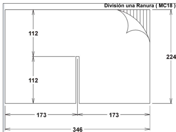
FIGURA 2. 25 MC18 DIVISIÓN UNA RANURA
