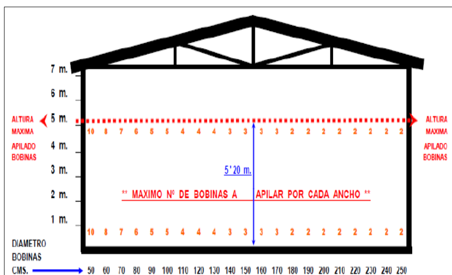
FIGURA 2. 38 APILAMIENTO DE BOBINAS SEGÚN DIÁMETRO
