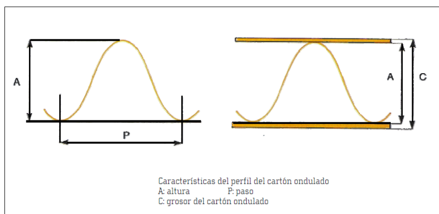
FIGURA 2. 5 CARACTERÍSTICAS DEL PERFIL DEL CARTÓN ONDULADO
