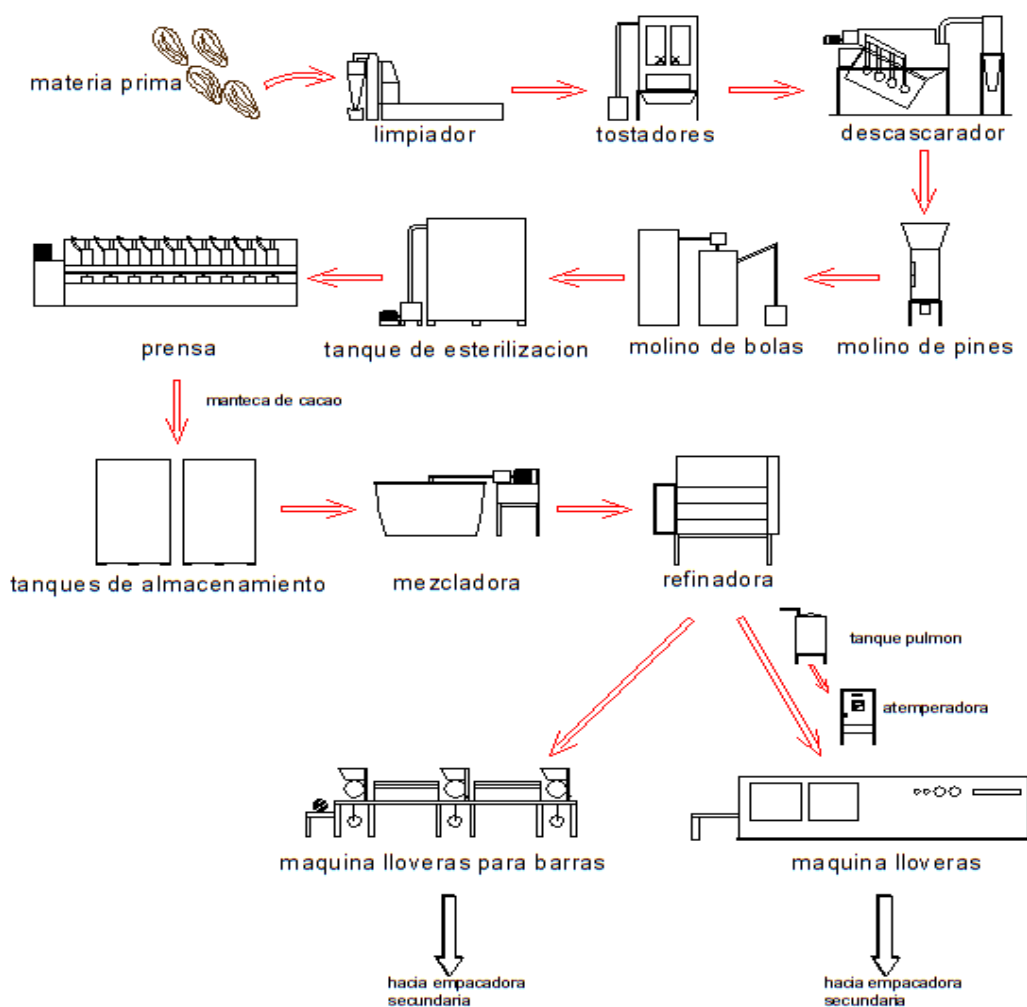
FIGURA 2.2 DIAGRAMA DE EQUIPOS DEL PROCESO
