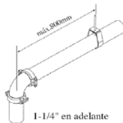
Corredor curvo de tubería
