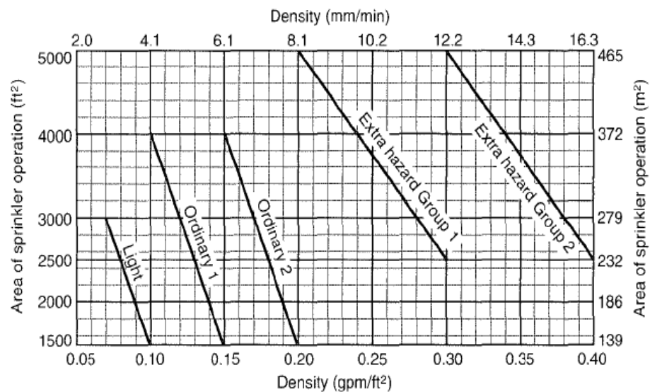
FIGURA 4.19 ÁREA/DENSIDAD [29]
