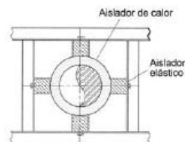
Tornillo pasador en U
