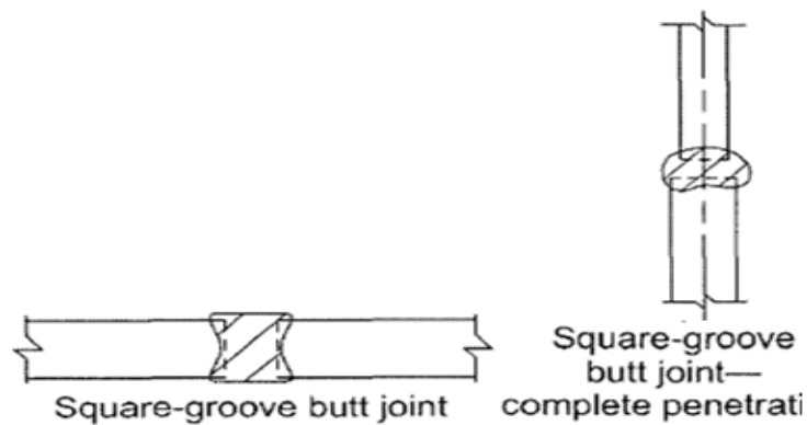
FIGURA 4.12 SOLDADURA DE TOPE A ESCUADRA HORIZONTAL
