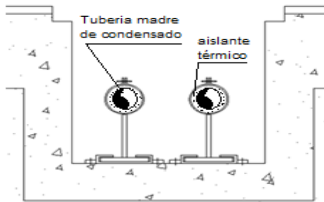
FIGURA 5.10 TUBERÍA DE RETORNO DE CONDENSADO MONTADA EN EL CANAL
