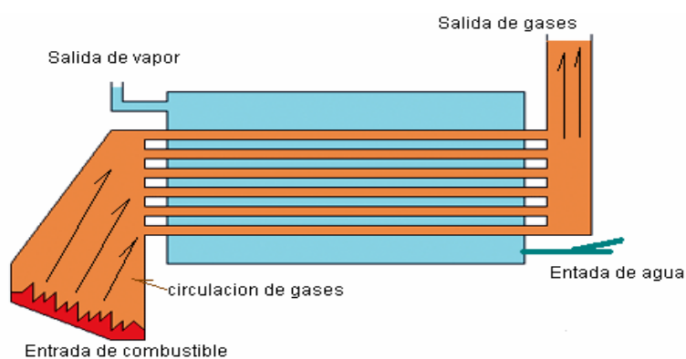
FIGURA 3.16 PRINCIPIO PIROTUBULAR [11]
