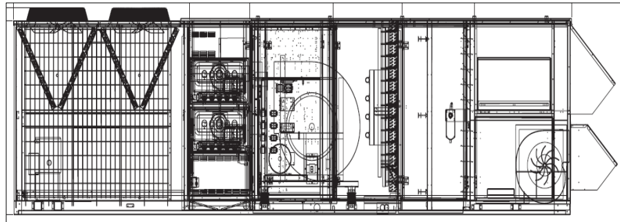
FIGURA 4.1 EQUIPO DE CLIMATIZACIÓN TIPO PAQUETE CON SISTEMA DE EXPANSIÓN DIRECTA 46
