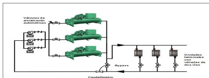
FIGURA 4.5 SISTEMA DE CAUDAL VARIABLE EN PRIMARIO (VPF)
