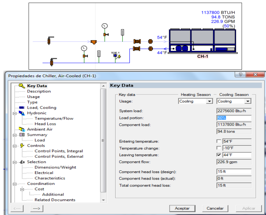
FIGURA 4.12 DIAGRAMA DE ENFRIADORES DE AGUA (CHILLERS) Y VENTANA DE INGRESO DE DATOS ELITE SOFTWARE – CHVAC SOLUTION PRO
