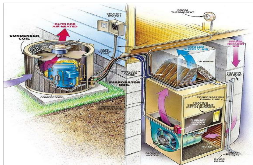
FIGURA 4.2 SISTEMA DE CLIMATIZACIÓN CENTRALIZADO CON MANEJADORAS DE AIRE 47
