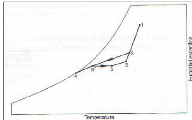
FIGURA 3.5.- REPRESENTACIÓN GRÁFICA DEL PROCESO DE ACONDICIONAMIENTO DE AIRE CON RECALENTAMIENTO 35
