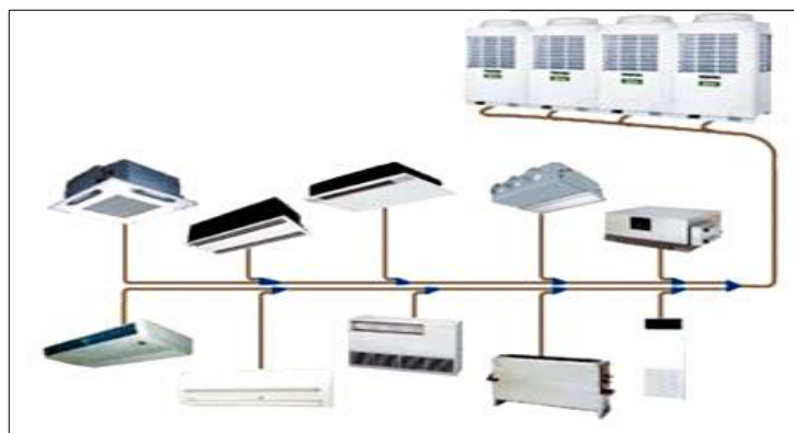
FIGURA 4.8 EQUIPO CON SISTEMA VRV Y SU VARIEDAD DE TIPO DE EVAPORADORES 49
