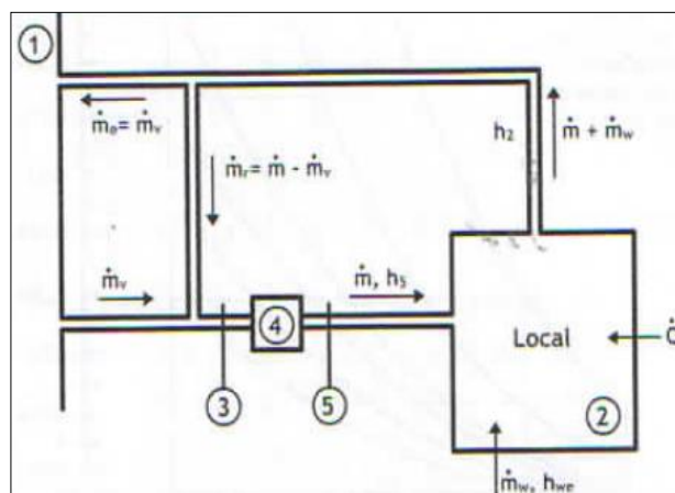
FIGURA 3.2 ESQUEMA DE UNA INSTALACIÓN DE PROCESO TÍPICO DE ENFRIAMIENTO DE AIRE 32
