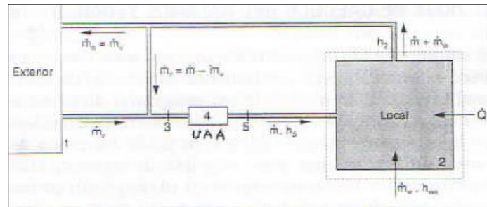
FIGURA 3.4 PROCESO DE ACONDICIONAMIENTO DE AIRE CON RECALENTAMIENTO 34
