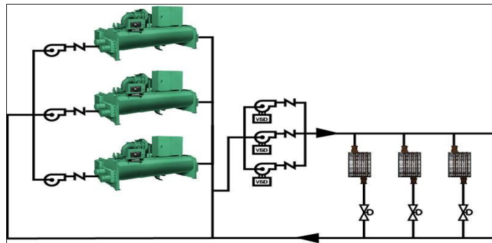
FIGURA 4.4 SISTEMA PRIMARIO/SECUNDARIO (PSF)
