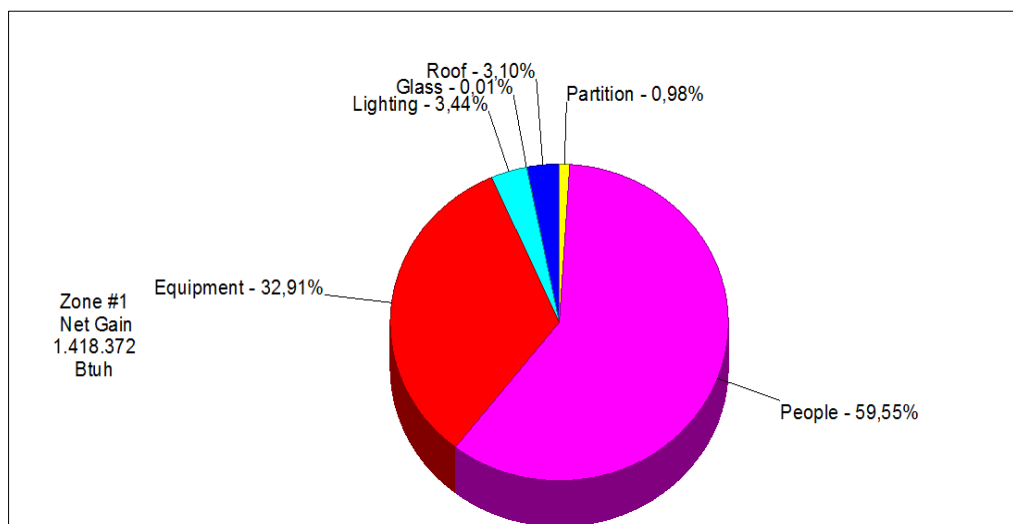
FIGURA 2.9 CARGAS TÉRMICAS “HORA A HORA” DE SALA DE PROCESO – CHAVC V7.0 / INCIDENCIA PORCENTUAL
