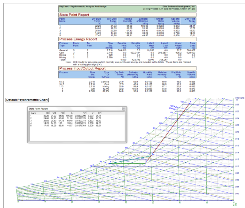
FIGURA 3.9 GRÁFICA Y REPORTE DE PSYCHART 2.01.60 PARA SALA DE PROCESO
