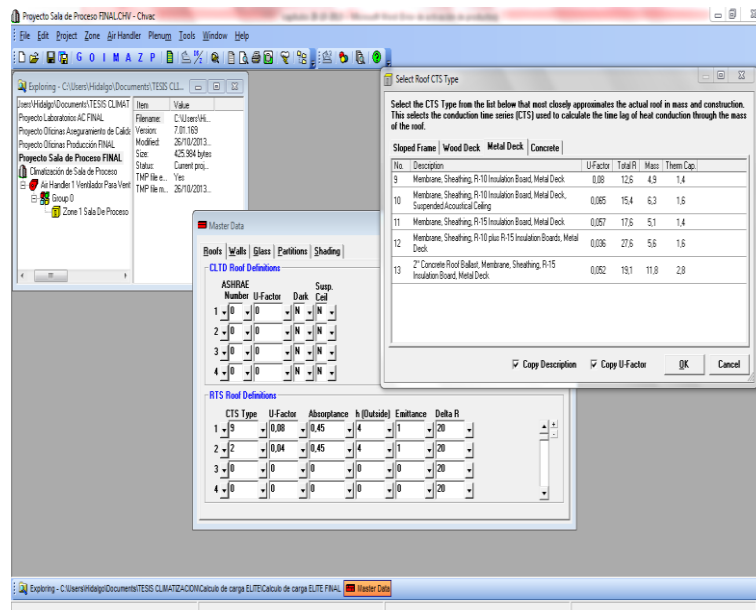
FIGURA 2.5 PANTALLA DE TRABAJO PARA EDITAR INFORMACIÓN MAESTRA – CHVAC V0.7
