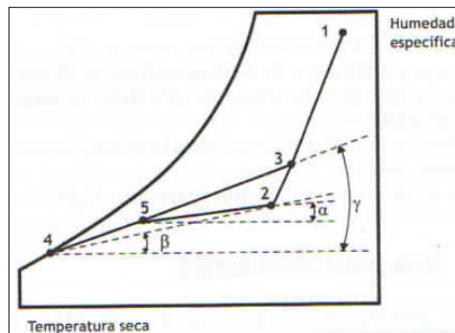
FIGURA 3.3 REPRESENTACIÓN GRÁFICA DEL PROCESO DE ENFRIAMIENTO DEL AIRE 33
