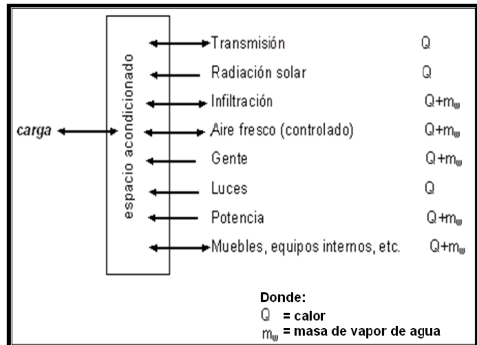
FIGURA 2.1 COMPONENTES BÁSICOS DE LAS CARGAS DE CALENTAMIENTO Y ENFRIAMIENTO. 18
