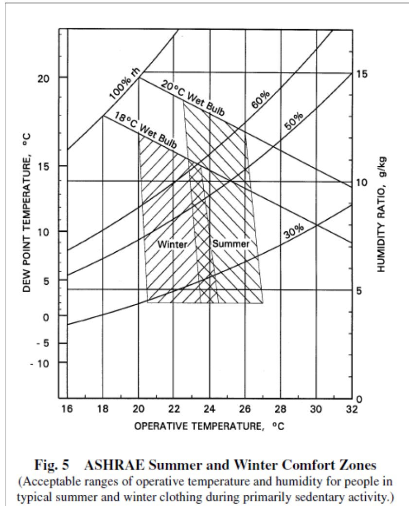
FIGURA 1.9 ASHRAE ZONAS DE CONFORT PARA INVIERNO Y VERANO 17
