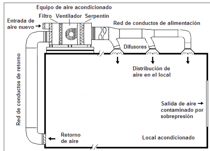
FIGURA 4.16 ESQUEMA BÁSICO DE SISTEMA DE DISTRIBUCIÓN DE AIRE. 53
