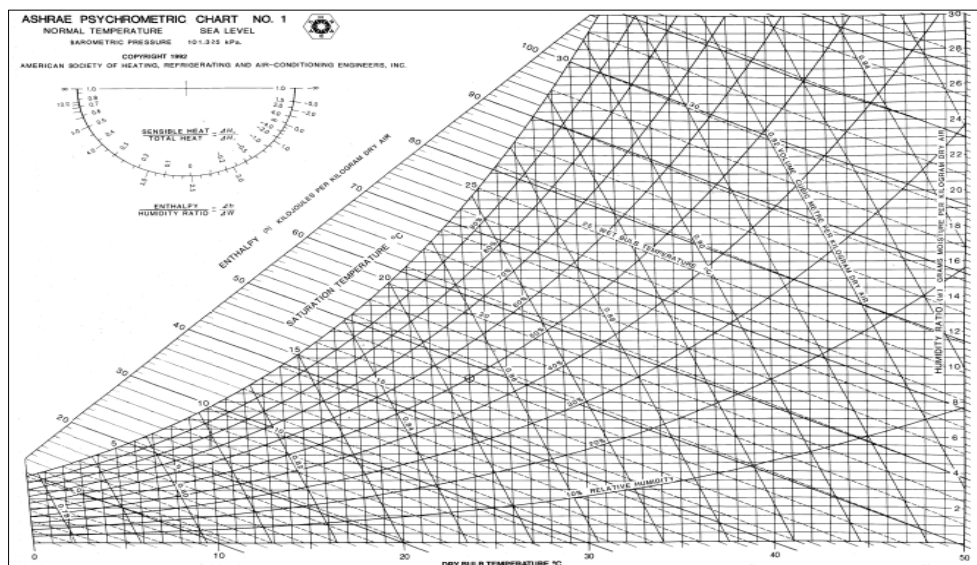
FIGURA 3.1 DIAGRAMA PSICROMÉTRICO 31
