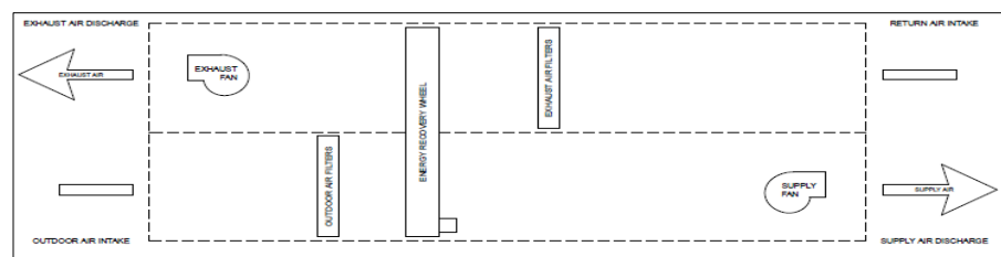
FIGURA 3.6 DIAGRAMA DE RECUPERADOR DE ENERGÍA GREENHECK 43
