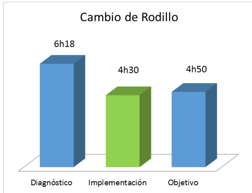
Gráfico 5.11. Tiempo utilizado en cambio de rodillo durante la etapa de diagnóstico e implementación
