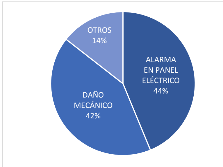
Gráfico 4.4. Causas de mayor cantidad de TPM en máquina empaquetadora 2
