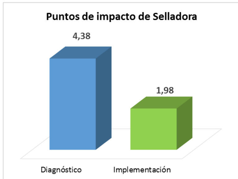
Gráfico 5.7. Puntos de la selladora ante el OEE durante la etapa de diagnóstico e implementación por el frente de TPM
