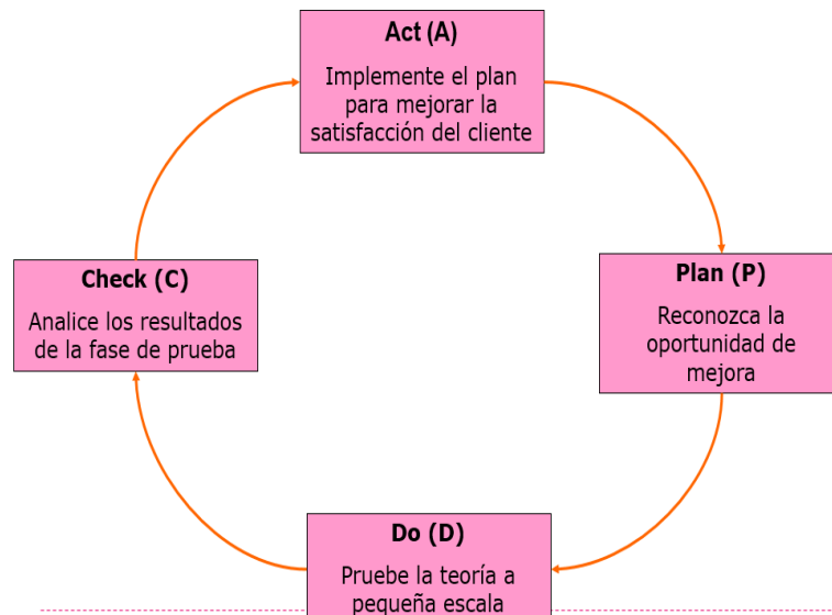
Figura 2.1. Ciclo Deming-Diapositivas.
