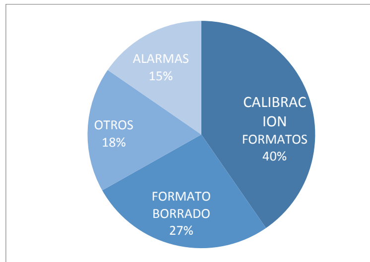
Gráfico 4.2. Causas de mayor cantidad de paradas menores en máquina empaquetadora 2
