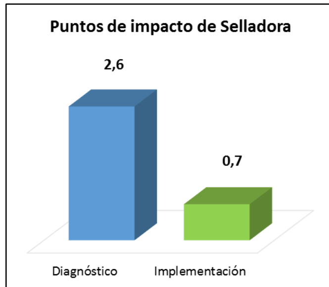
Gráfico 5.2. Puntos de la selladora ante el OEE durante la etapa de diagnóstico e implementación por el frente de Paradas Menores
