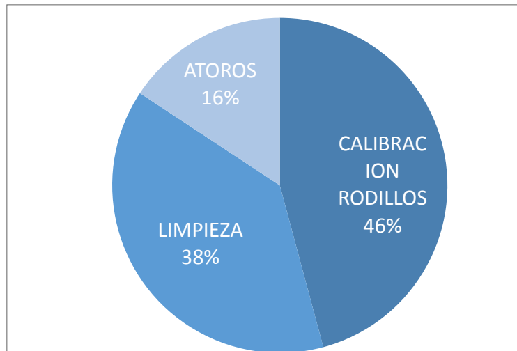
Gráfico 4.1. Causas de mayor cantidad de paradas menores en máquina rebobinadora
