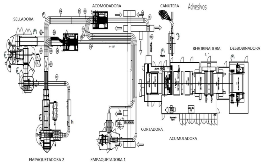
Figura 3.2. Esquema de línea de producción de papel higiénico. Fuente: Área de proyectos de la compañía
