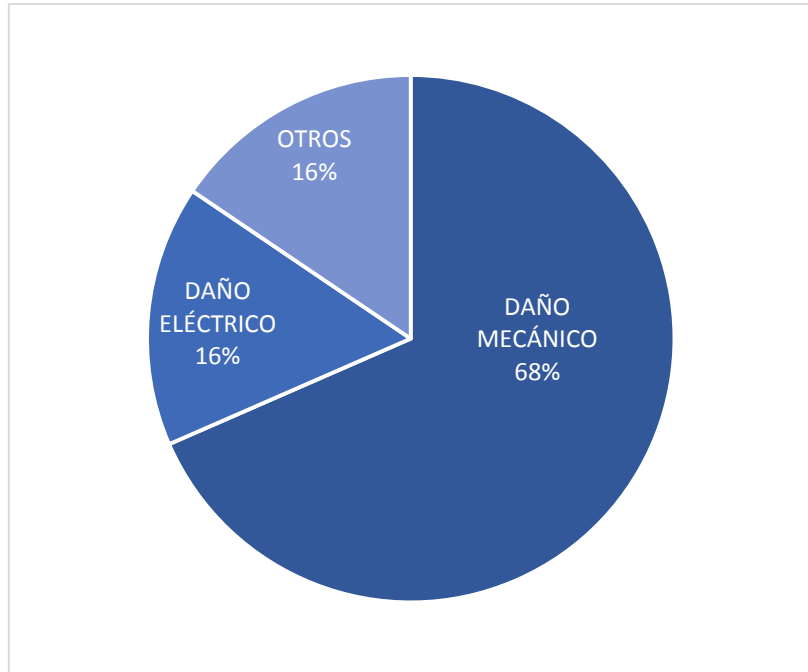
Gráfico 4.6. Causas de mayor cantidad de TPM en máquina selladora
