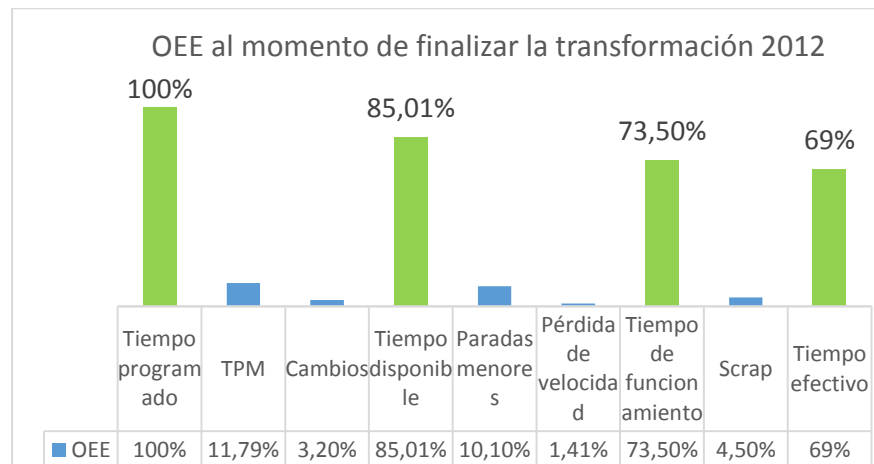
Gráfico 5.24. Escalera de OEE al finalizar la transformación lean manufacturing
