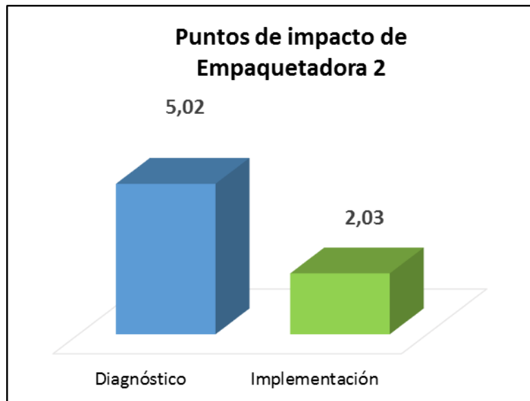
Gráfico 5.6. Puntos de la empaquetadora 2 ante el OEE durante la etapa de diagnóstico e implementación por el frente de TPM
