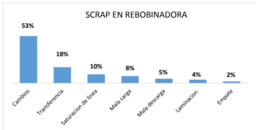
Gráfico 4.11. Porcentaje de scrap en rebobinadora
