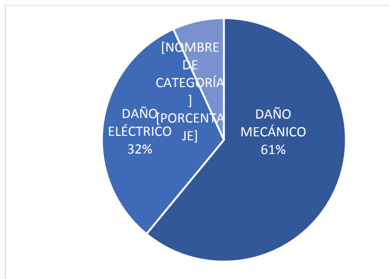
Gráfico 4.5. Causas de mayor cantidad de TPM en máquina cortadora
