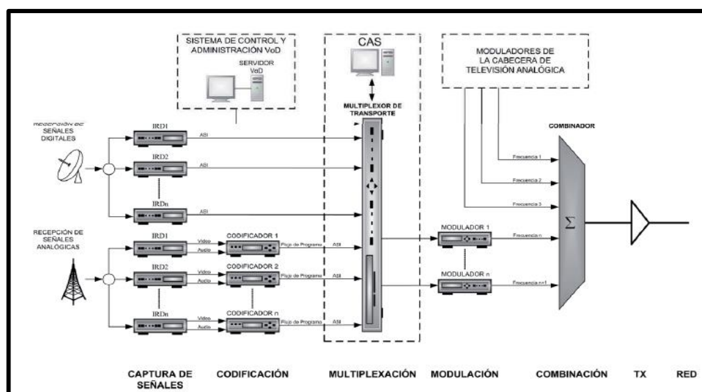
Figura 3. 14. Esquema de una Cabecera. [20]
