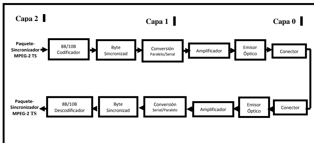
Figura 3. 3. Transmisión ASI por fibra óptica. [19]
