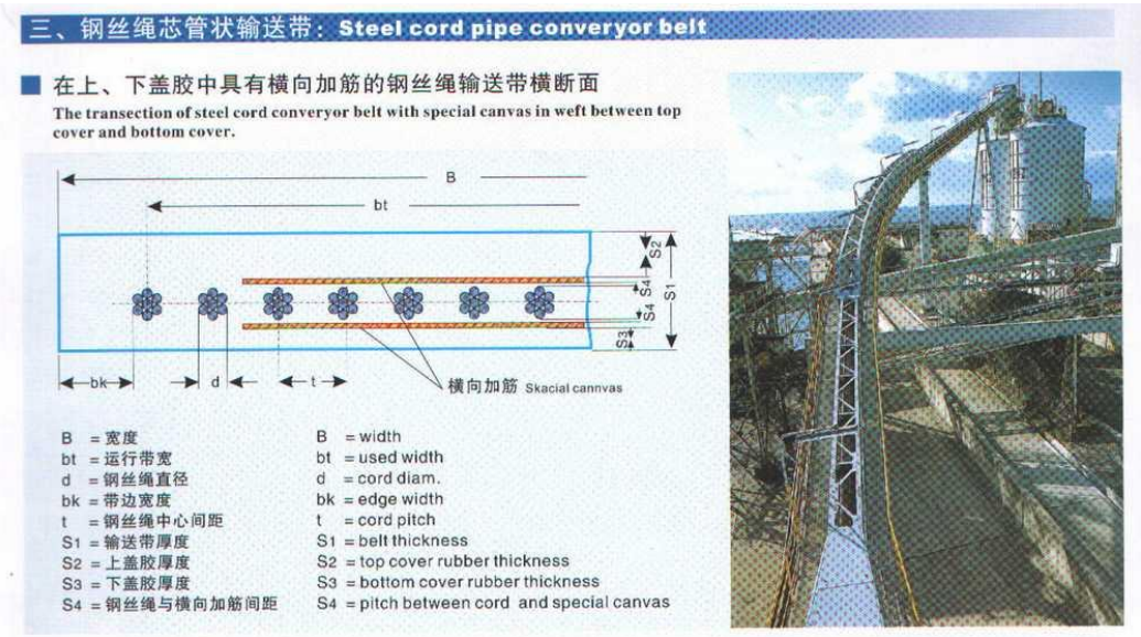
钢丝绳芯管状带主要技术参数 Technical data for steel cord pipe conveyer belt
