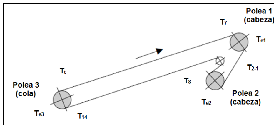
FIGURA 4.6 DISTRIBUCIÓN DE POTENCIA DEL TRANSPORTADOR
