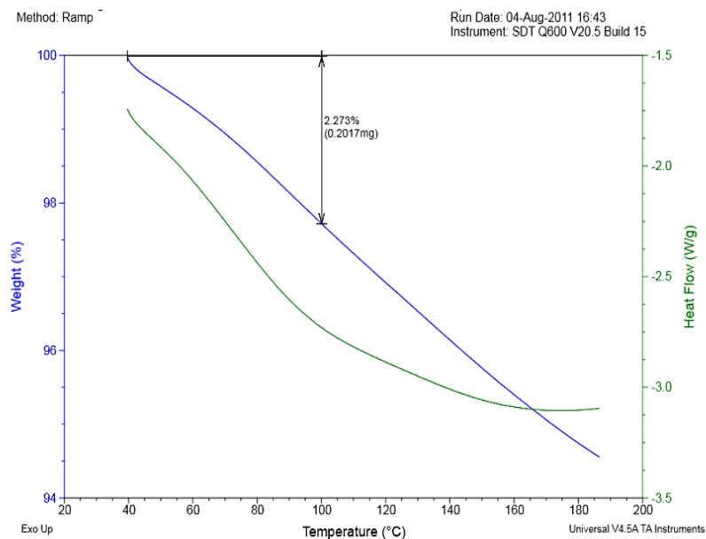
Figura 3.8. Termograma final del testigo x_3
