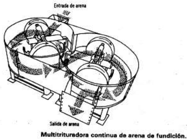
FIGURA 1.5. MOLINO PARA ARENA DE FUNDICIÓN
