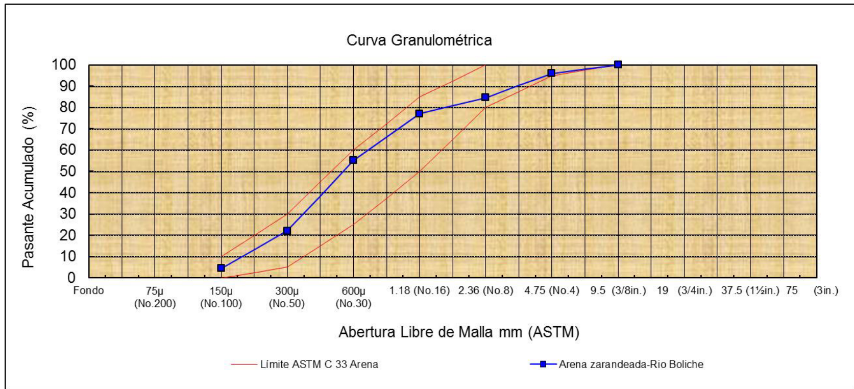
Gráfico 2. Curva Granulométrica de la Arena de Rio
