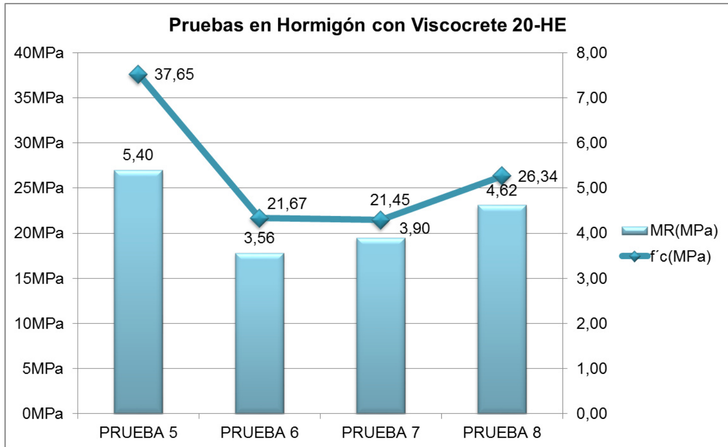
Gráfico 9 Resultados de pruebas en Hormigón con el aditivo Viscocrete 20 HE
