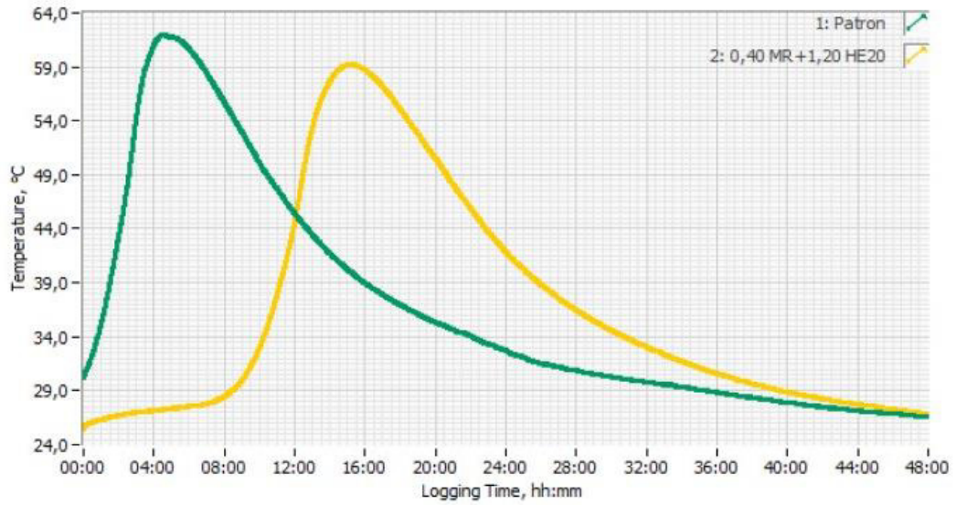
Gráfico 6 Grafico de Tiempo vs Generación de Temperatura con el Holcim Heat
