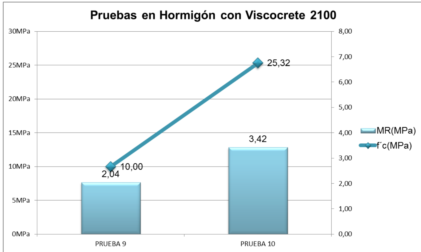
Gráfico 10 Resultados de pruebas en Hormigón con el aditivo: Viscocrete 2100
