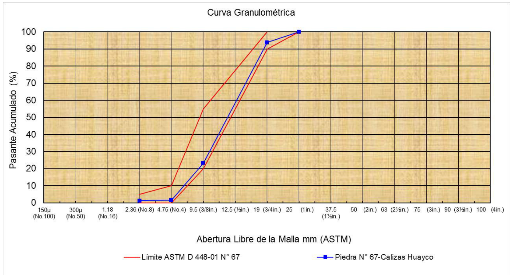
Gráfico 5 Curva Granulométrica de la Piedra # 67
