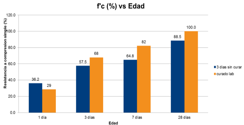
Gráfico 1 Resistencia a la compresión de hormigón curado continuo y de hormigón curado después de 3 días sin hidratar.
