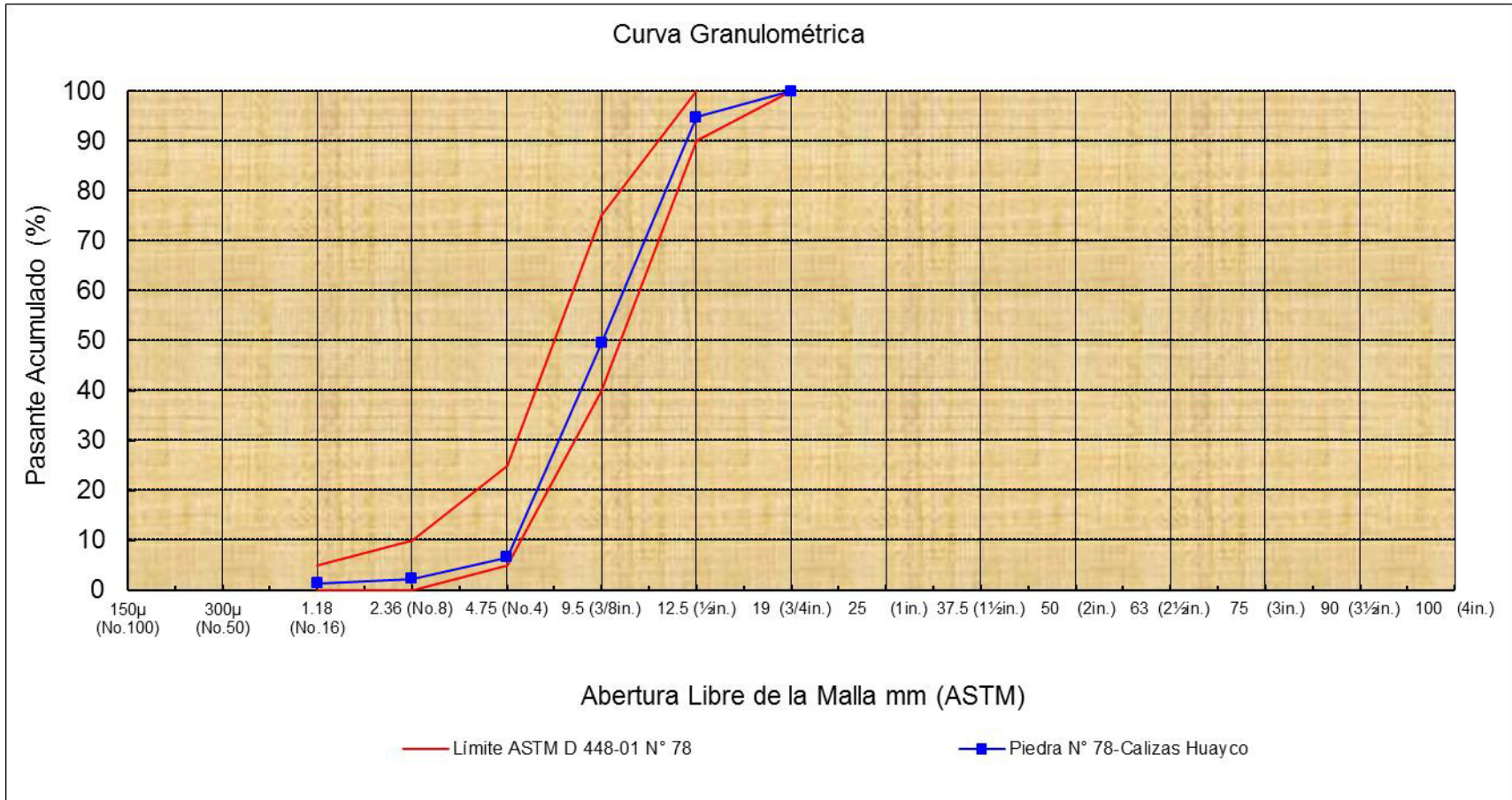
Gráfico 4 Curva Granulométrica de la Piedra # 78
