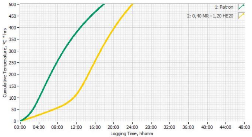
Gráfico 7 Grafico Tiempo vs Temperatura Acumulada con el HolcimHeat
