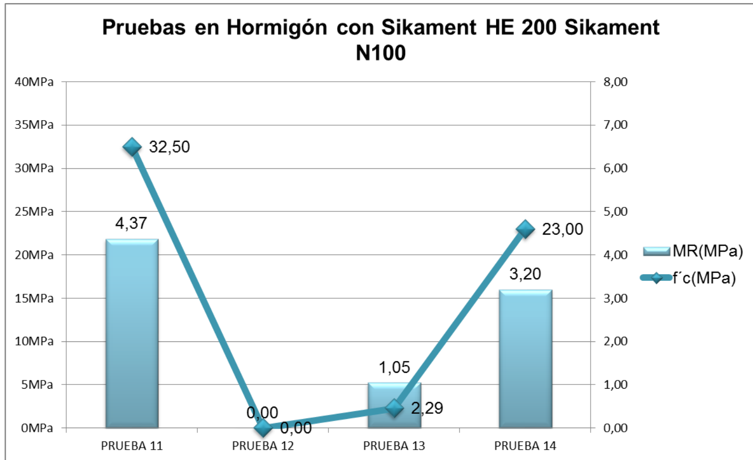
Gráfico 11 Resultados de pruebas en Hormigón con los aditivos: Sikament HE200 y Sikament N100
