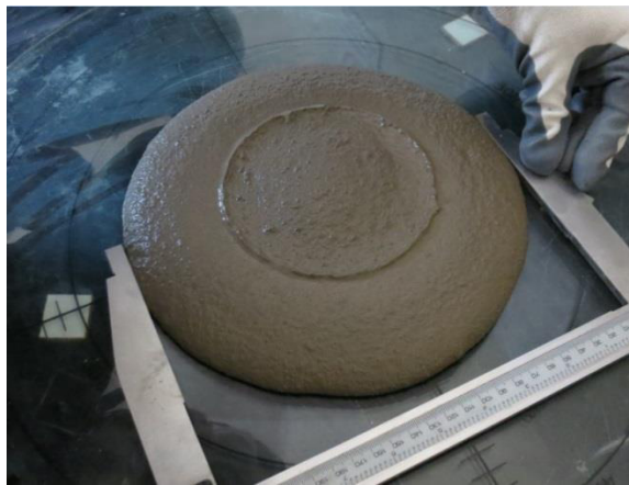
Fotografía 4.21 Medición de Flujo a los 10 minutos
