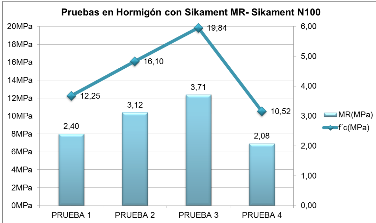
Gráfico 8 Resultados de pruebas en Hormigón con los aditivos: Sikament MR-Sikament N100
