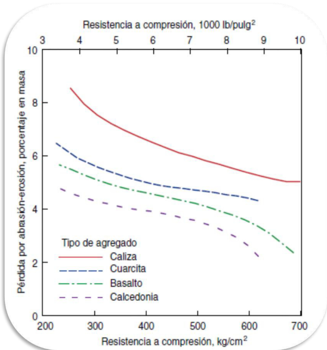
Gráfico 1 Efecto de la resistencia a la compresión y del tipo de agregado sobre la resistencia a la abrasión del hormigón
