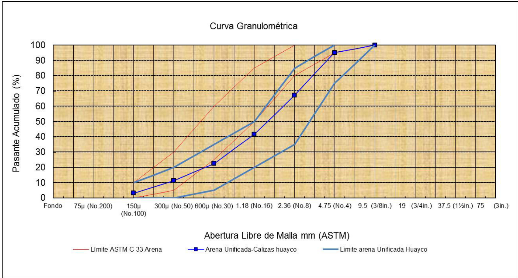
Gráfico 3 Curva Granulométrica de la Arena Unificada
