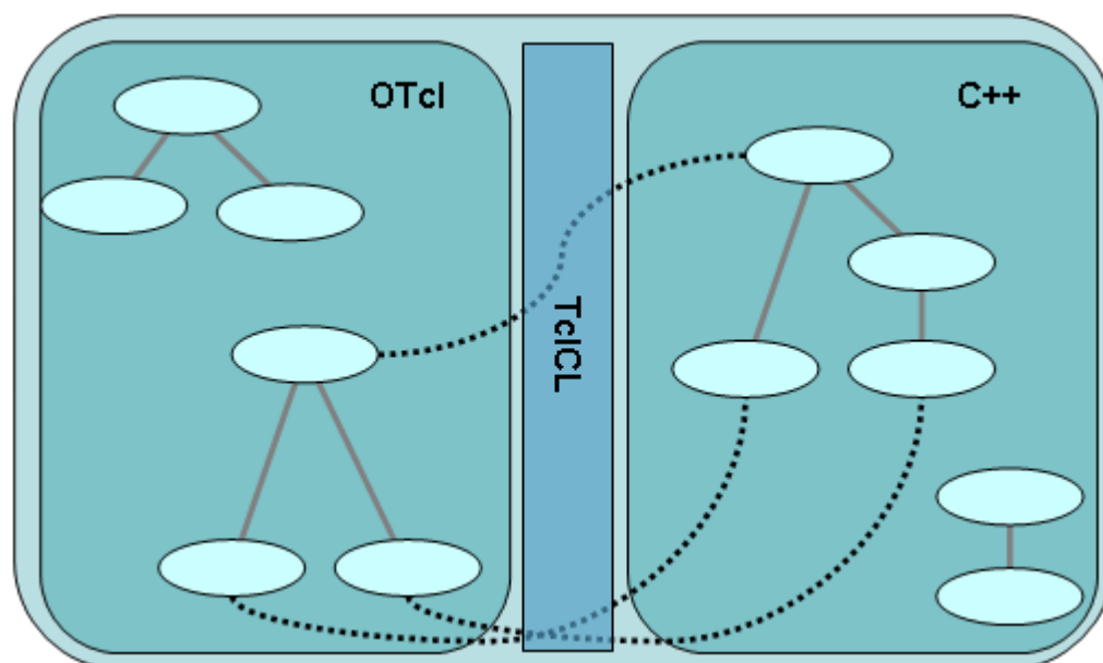
Figura 3.1. Modelo de Programación de dos lenguajes.
