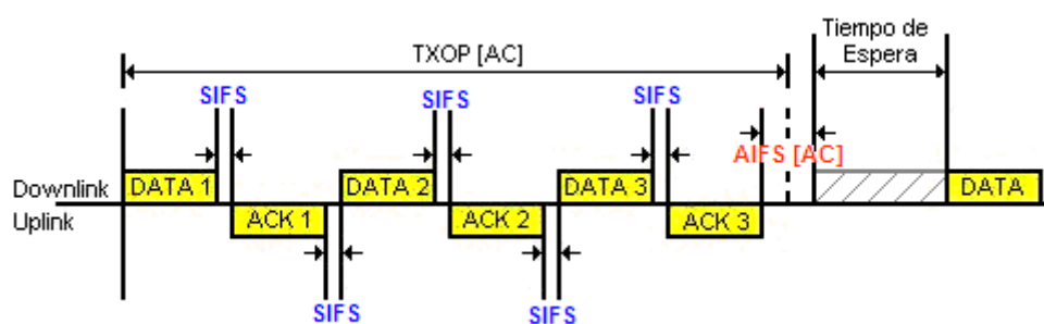
Figura 2.3. CFB
