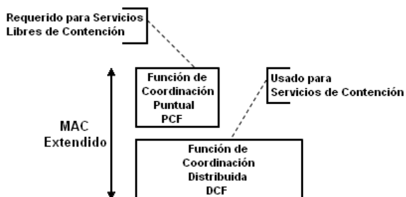
Figura 2.1. Arquitectura MAC
