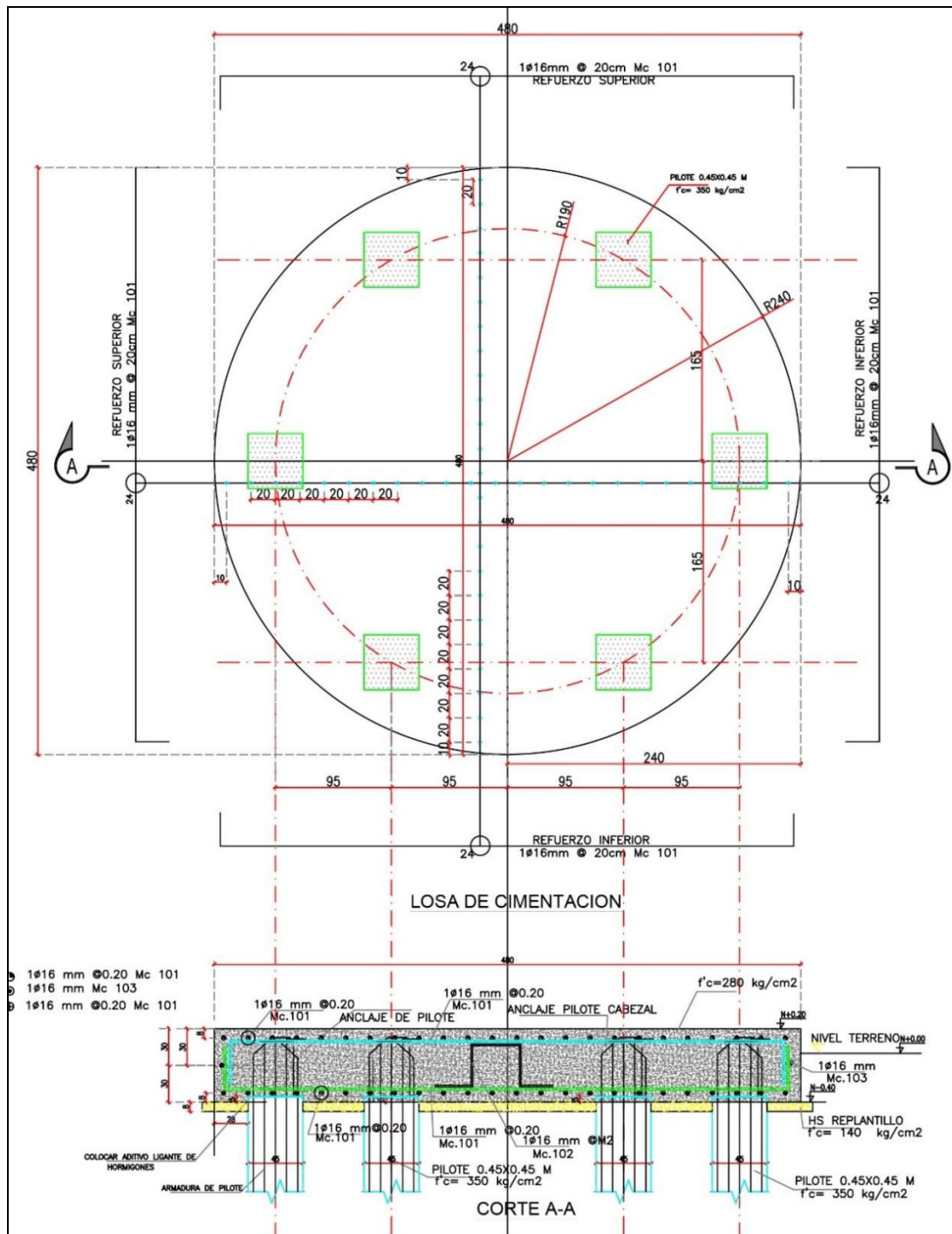
Figura 5.12. Diseño estructural de la losa.
