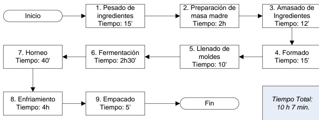
Elaborado por: Everaldo Ramírez, 2012 Figura 2.2- Diagrama de flujo del proceso tradicional de elaboración de pan de molde blanco.
