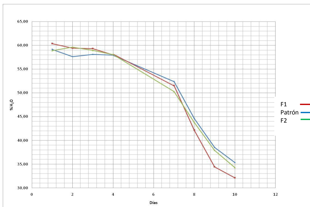
Figura 2.16- Curva de Variación de la Humedad vs. Tiempo
