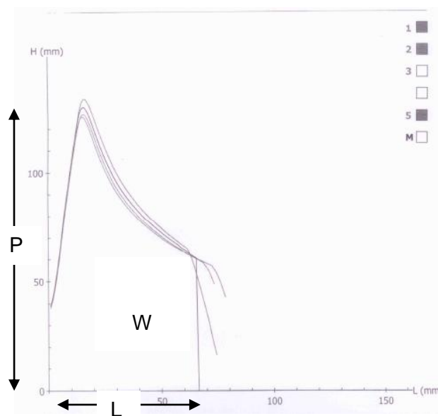
Figura 2.1- Curva del alveograma de muestra 2 de harina, seleccionada para elaboración de pan de molde blanco.
