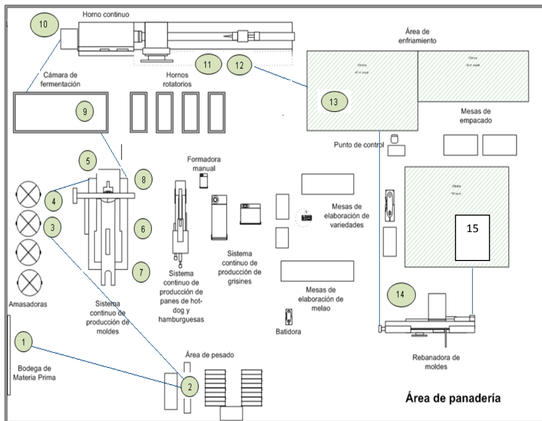
Elaborado por: Everaldo Ramírez, 2012 Figura 2.5- Layout del proceso mejorado de la planta Fantasía
