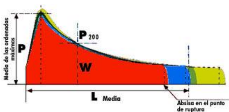
Fuente. http://www.grupomoliner.com.ar/grupo_moliner_alveograma.htm Figura 1.9- Alveograma obtenido con Alveógrafo NG de Chopin
