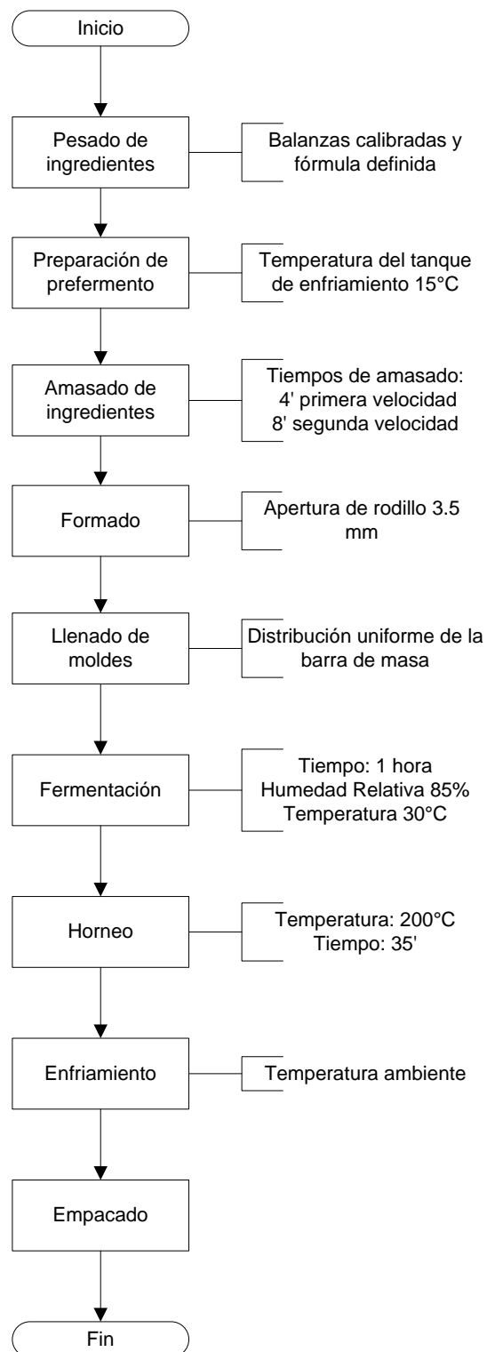
Elaborado por: Everaldo Ramírez, 2012 Figura 2.3- Diagrama de flujo del proceso mejorado y puntos de control
