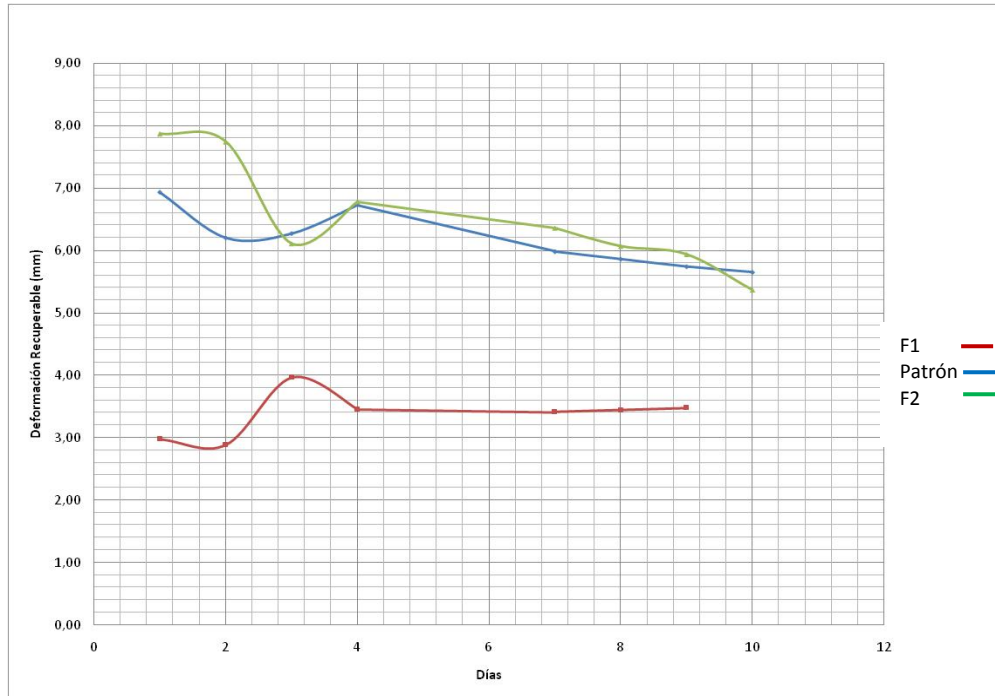
Figura 2.14- Curva de Deformación recuperable vs. Tiempo
