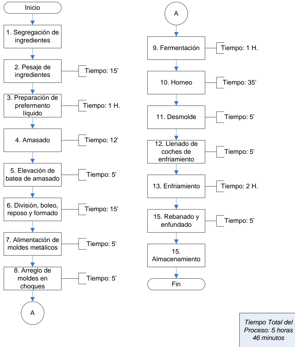
Figura 2.4- Diagrama de flujo del proceso mejorado y tiempos de proceso
