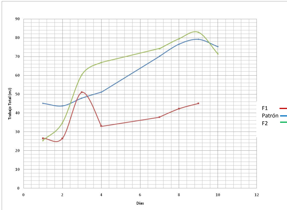
Figura 2.15- Curva de Variación de Trabajo Total vs. Tiempo
