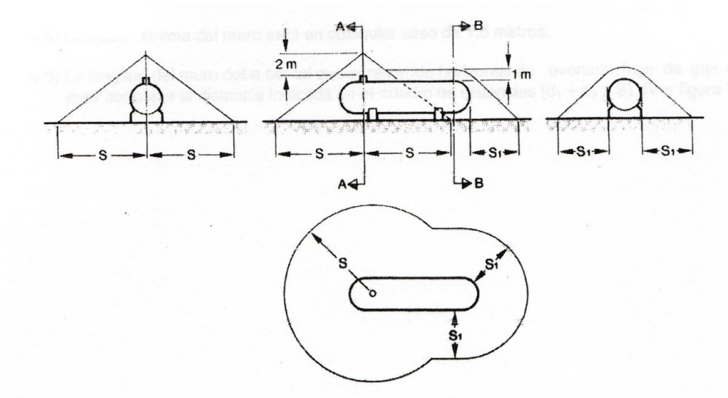
FIGURA 1: TANQUES SOBRE EL NIVEL DEL TERRENO
