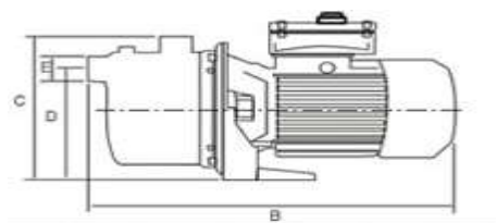
Figura 3.14 Bomba.
