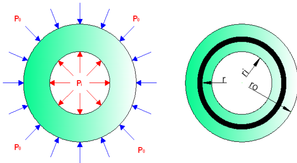
FIGURA 2.2. CILINDRO SOMETIDO A PRESIONES INTERNAS Y EXTERNAS
