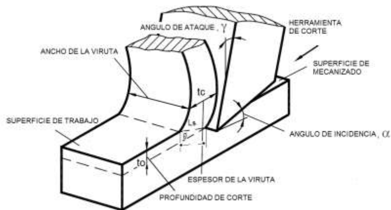
Figura 1.8 Modelo de corte ortogonal 2
