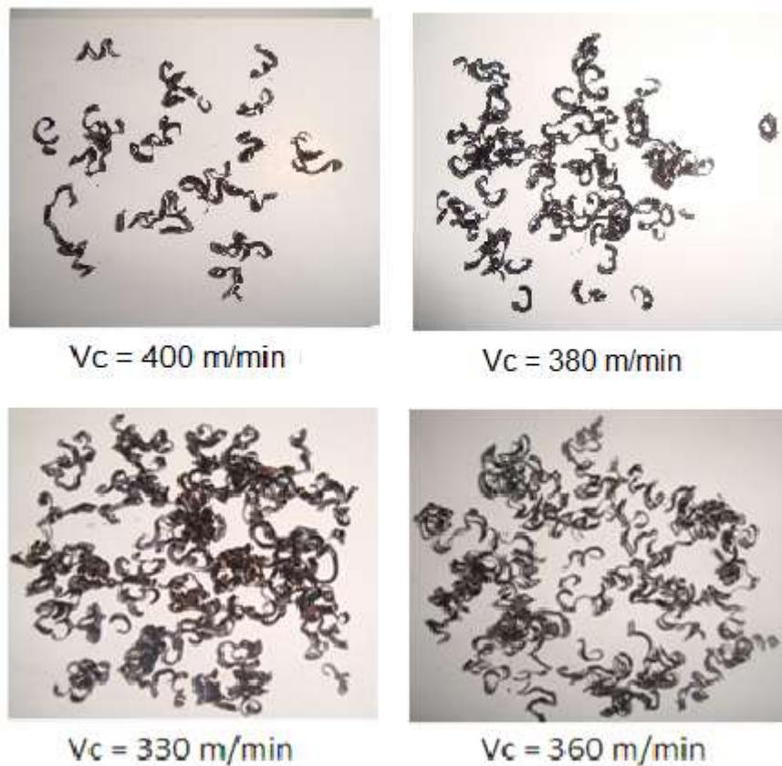
Figura 4.7. Formación de la viruta con la herramienta TNMG160404-PF GC4215 a distintas velocidades de corte
