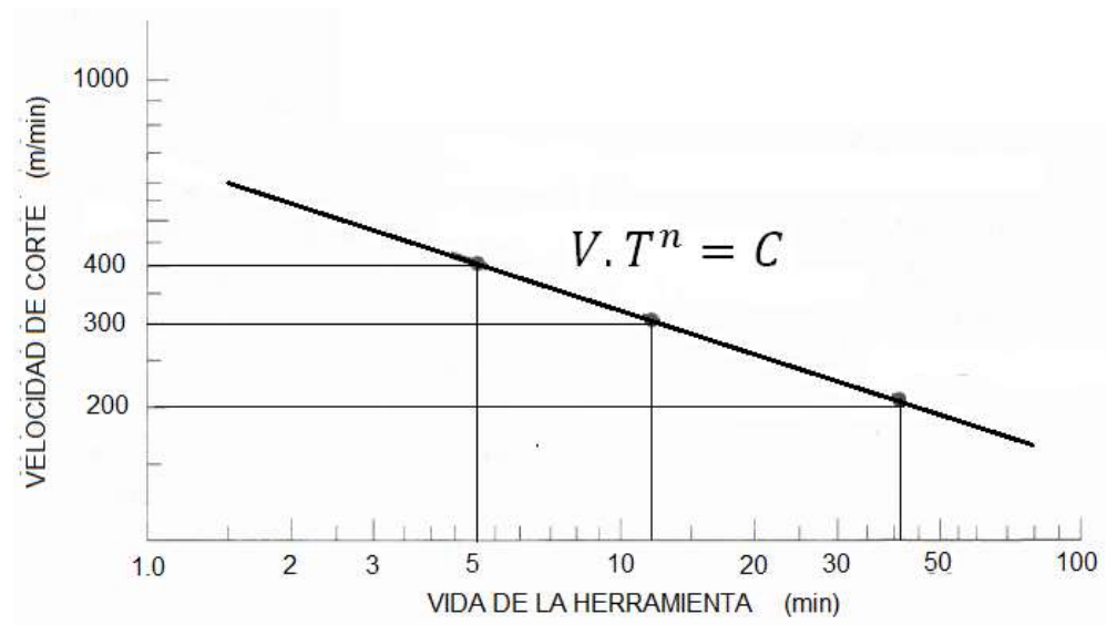
Figura 1.21. Gráfico de velocidad de corte vs tiempo de maquinado en escalas logarítmicas
