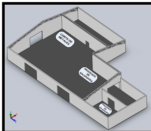
FIGURA 3.3. SECTORES PARA EXTRACCIÓN LOCALIZADA
