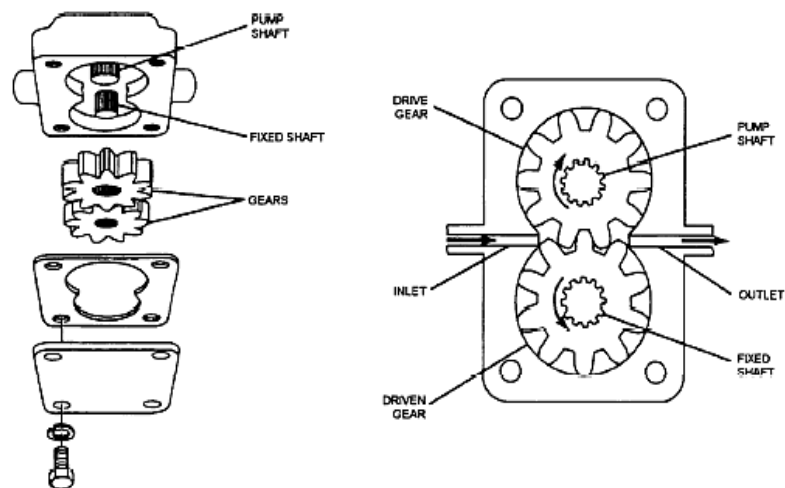
FIGURA 4.4 BOMBA DE ENGRANES PARA COMBUSTIBLE
