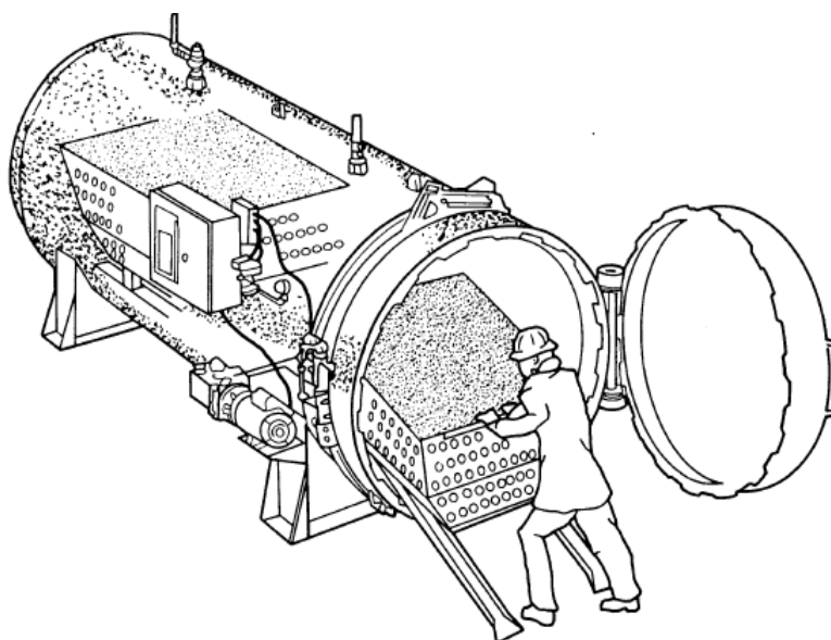
FIGURA 2.9 AUTOCLAVE DE AMSCO, ERIE, PA. SIENDO CARGADO POR OPERADOR
