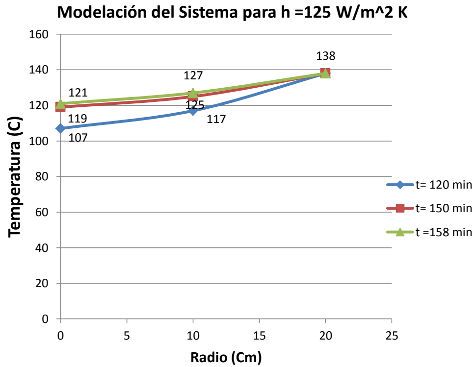
FIGURA 3.5 MODELACIÓN DE CURVA DE CALENTAMIENTO PARA COEFICIENTE CONVECTIVO DE GASES DE 125 \text{ W/M}^2 \text{ K}
