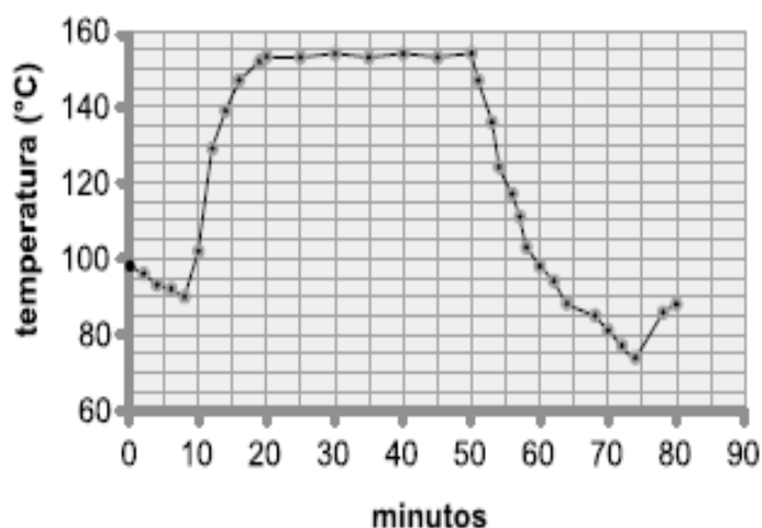
FIGURA 2.7 CUADRO TÍPICO DE TEMPERATURA VS TIEMPO EN AUTOCLAVES USANDO VACÍO EN SU PROCESO
