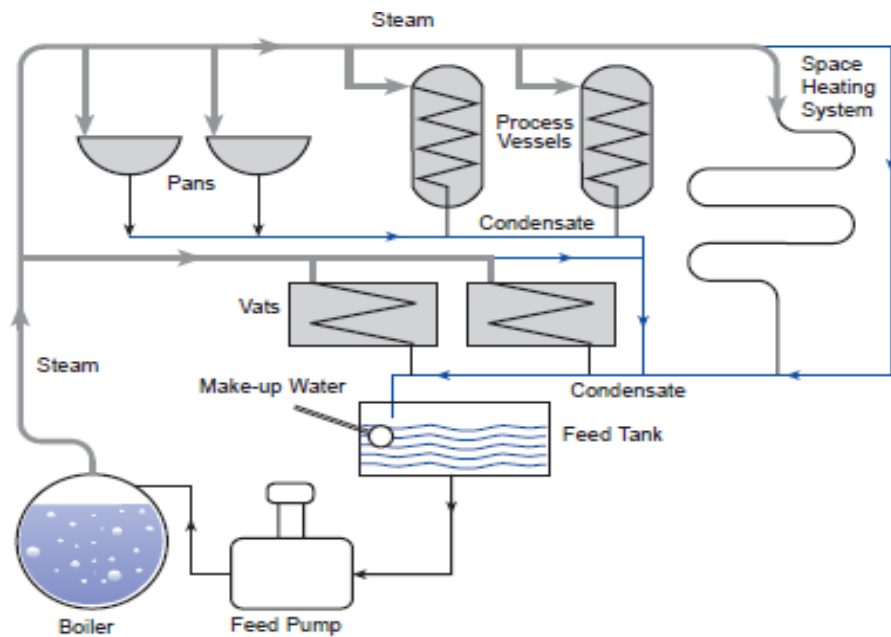
FIGURA 4.3 CIRCUITO TÍPICO DE SUMINISTRO DE VAPOR.
