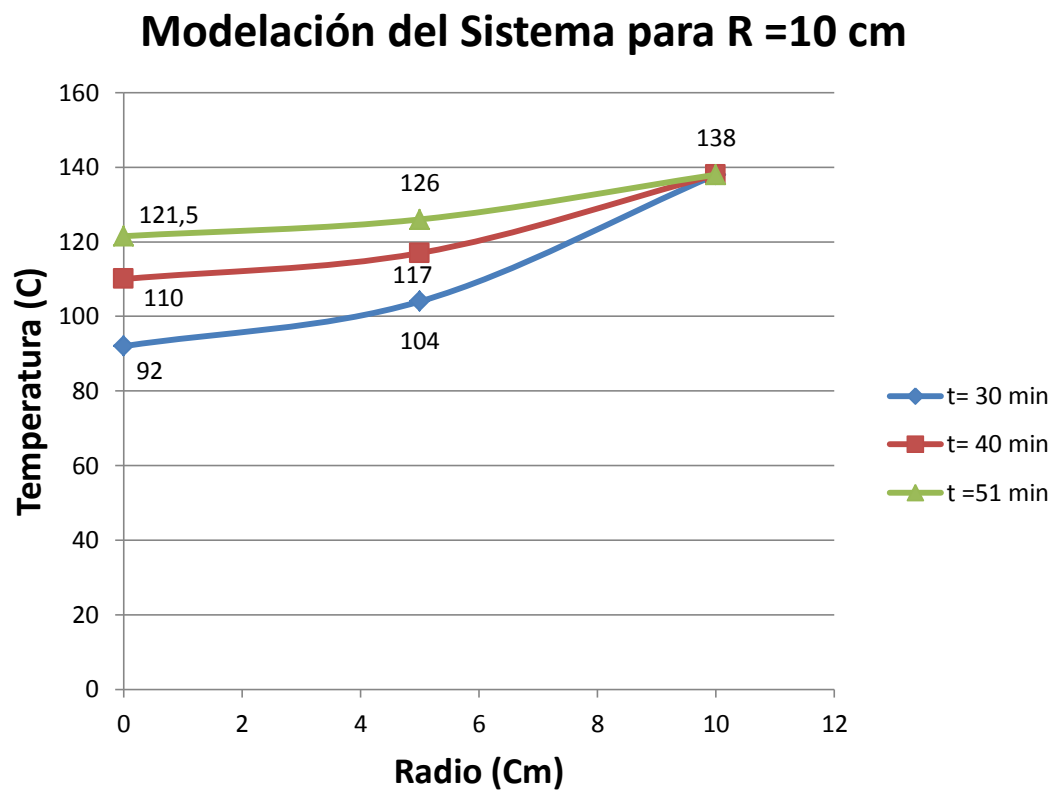
FIGURA 3.8 MODELACIÓN DE CURVA DE CALENTAMIENTO PARA BOLSA DE RSH CON RADIO DE 10 CM.
