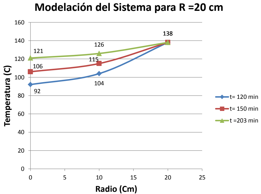
FIGURA 3.7 MODELACIÓN DE CURVA DE CALENTAMIENTO PARA BOLSA DE RSH CON RADIO DE 20 CM.
