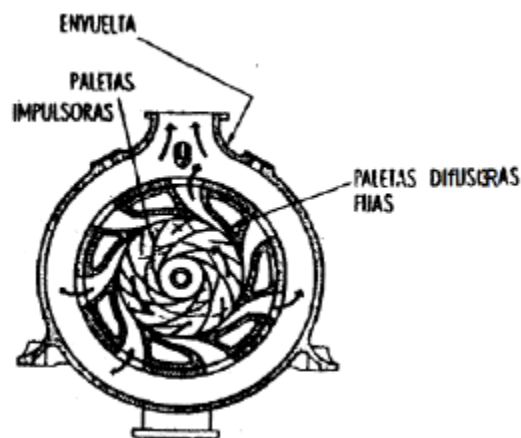
FIGURA 4.2 BOMBA TIPO TURBINA
