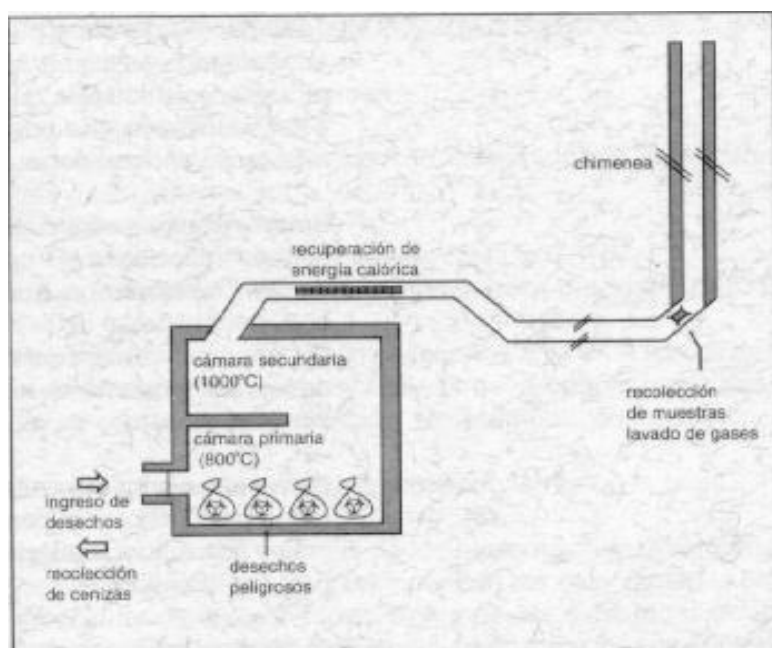
FIGURA 2.6 INCINERADOR DE DOBLE CÁMARA
