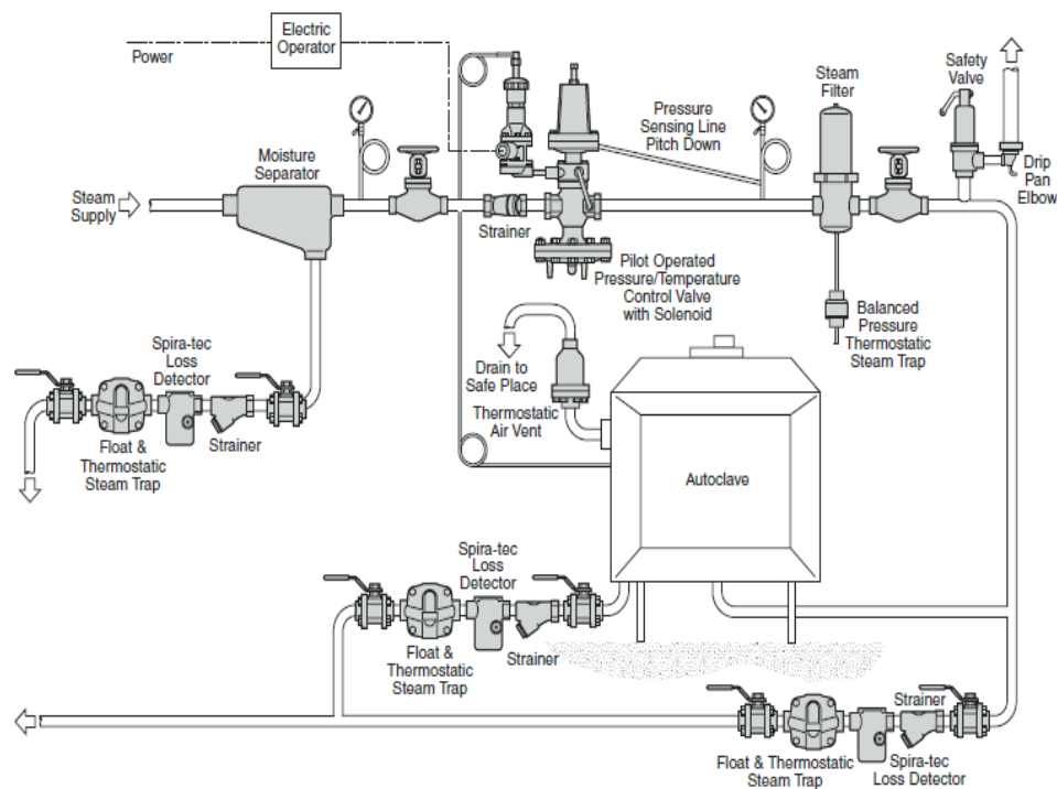
FIGURA 4.5 AUTOCLAVE CON SISTEMA ELECTRÓNICO DE CONTROL POR LOTES
