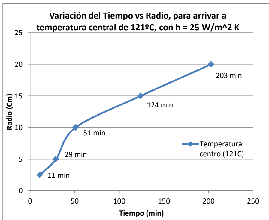
FIGURA 3.9 RELACIÓN TIEMPO VS RADIO DE LAS BOLSAS DE RSH PARA LLEGAR A 121^{\circ}\text{C} EN EL CENTRO
