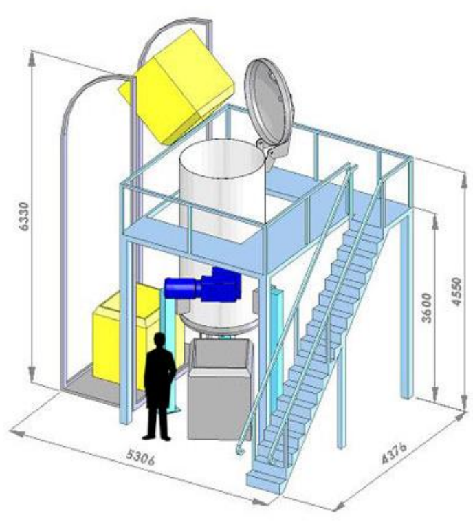
FIGURA 3.1 ESQUEMA DE AUTOCLAVE T1000 ECODAS, 150 KG/CICLO
