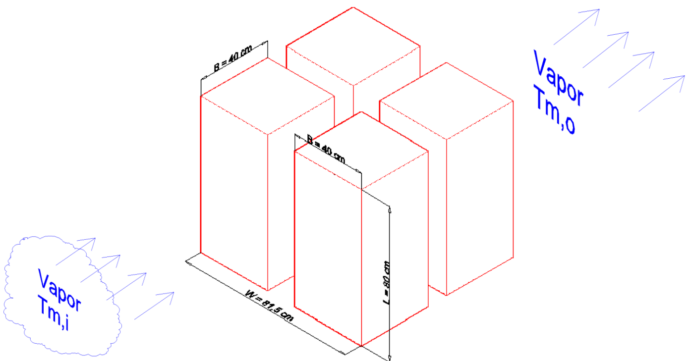
FIGURA 3.2 MODELACIÓN DEL PROCESO, VAPOR CON BOLSAS DE RSH
