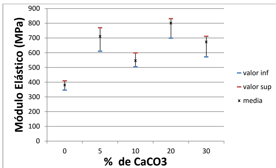
FIGURA 4.1 MÓDULO DE ELASTICIDAD DE LOS COMPUESTOS
