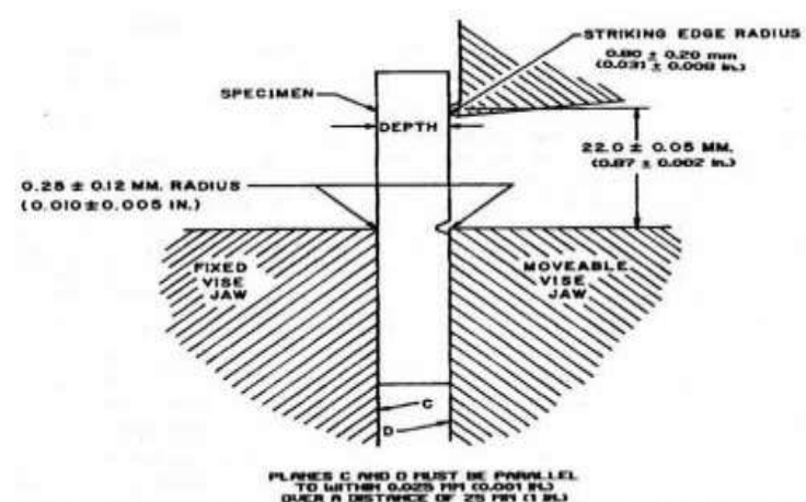
FIGURA 3.14 RELACIÓN DEL TORNILLO DE SUJECIÓN, ESPÉCIMEN Y BORDE DE IMPACTO.
