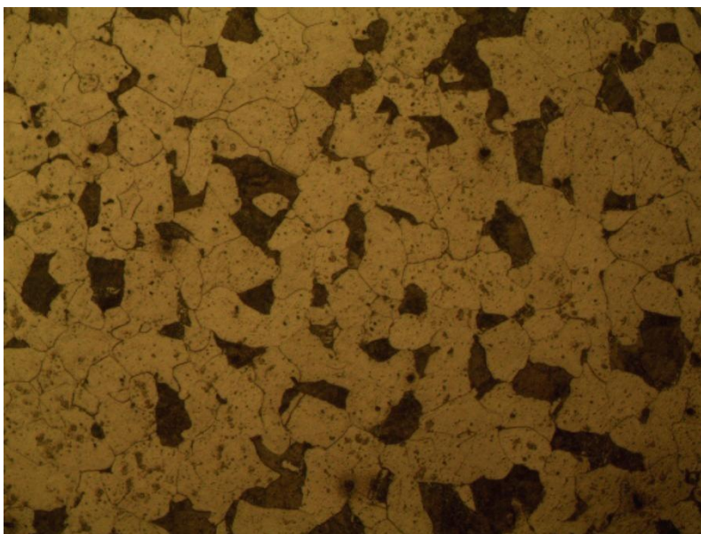
FIGURA 3.5: MICROESTRUCTURA SECCIÓN TRANSVERSAL (500 X). NITAL 3%
