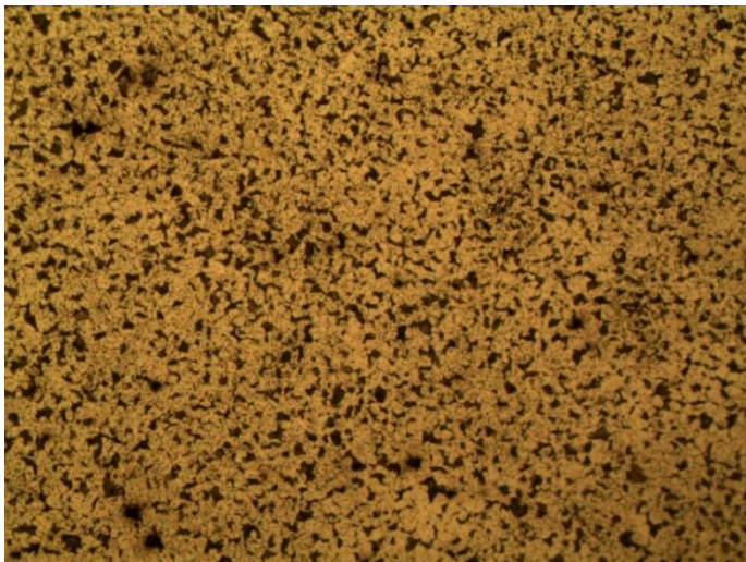
FIGURA 3.4: MICROESTRUCTURA SECCIÓN TRANSVERSAL (100 X). NITAL 3%
