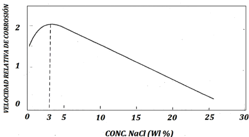
FIGURA 2.3: INFLUENCIA DE LA CONCENTRACIÓN DE NaCl EN LA VELOCIDAD DE CORROSIÓN DEL ACERO
