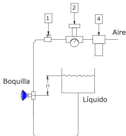
Fig 4 Sistema de atomización por sifón
