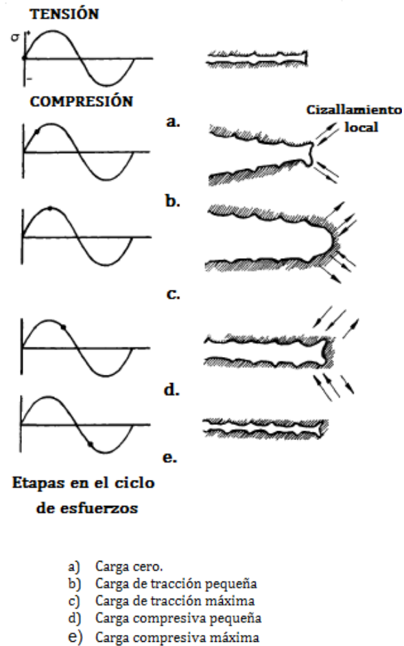
FIGURA 1.5: ILUSTRACIÓN ESQUEMÁTICA DE LOS MECANISMOS DE PROPAGACIÓN DE FISURAS (ETAPA II)
