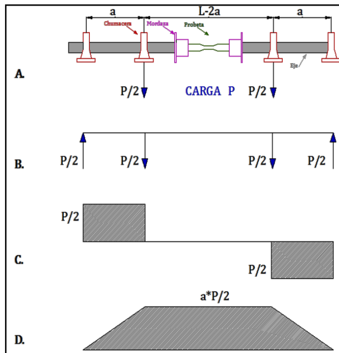
FIGURA 3.12: DIAGRAMA GENERAL DE ESFUERZOS DE UNA PROBETA A FATIGA EN FLEXIÓN ROTATIVA
