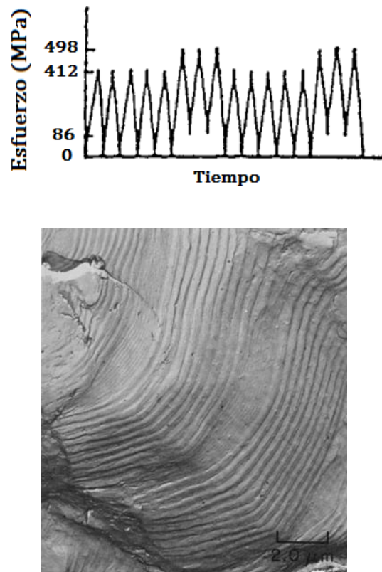
FIGURA 1.8: ESTRÍAS DE FATIGA CUANDO SE CAMBIA LA AMPLITUD DE TENSIONES
