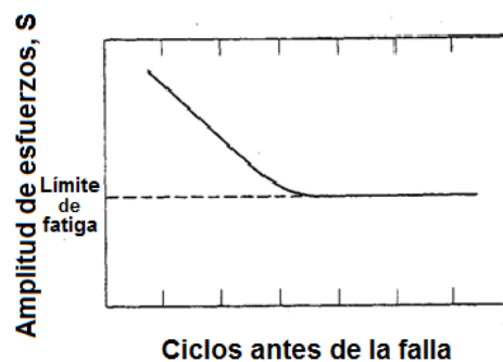
a) Material que muestra un límite de fatiga.
