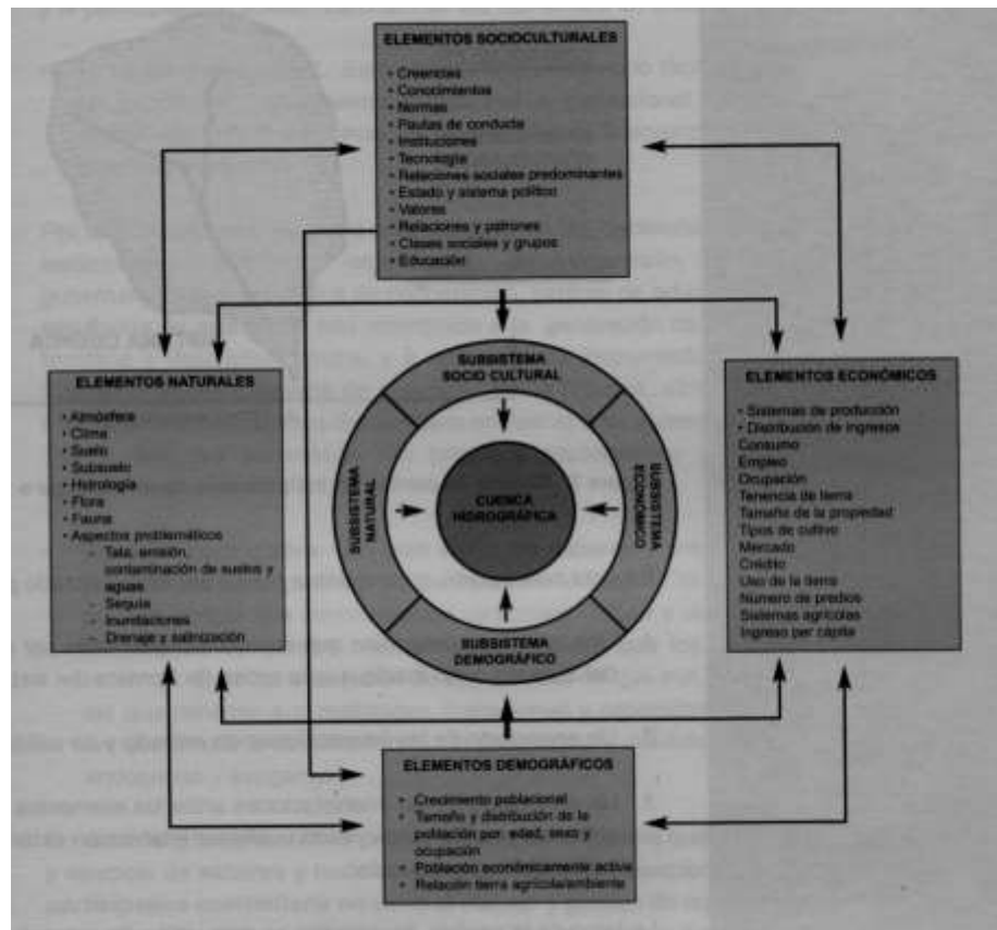
FIGURA 5. LA CUENCA HIDROGRÁFICA COMO SISTEMA, SUS ELEMENTOS E INTERACCIONES (16).
