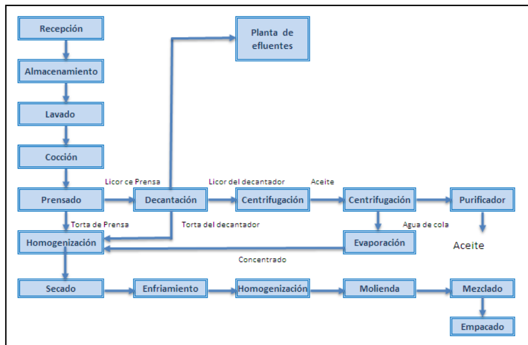
FIGURA 1.1 DIAGRAMA DE BLOQUES PARA ELABORACIÓN DE HARINA DE PESCADO
