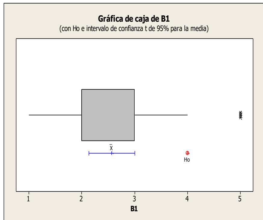
FIGURA 3.4: GRÁFICO DE CAJA MUESTRA B1
