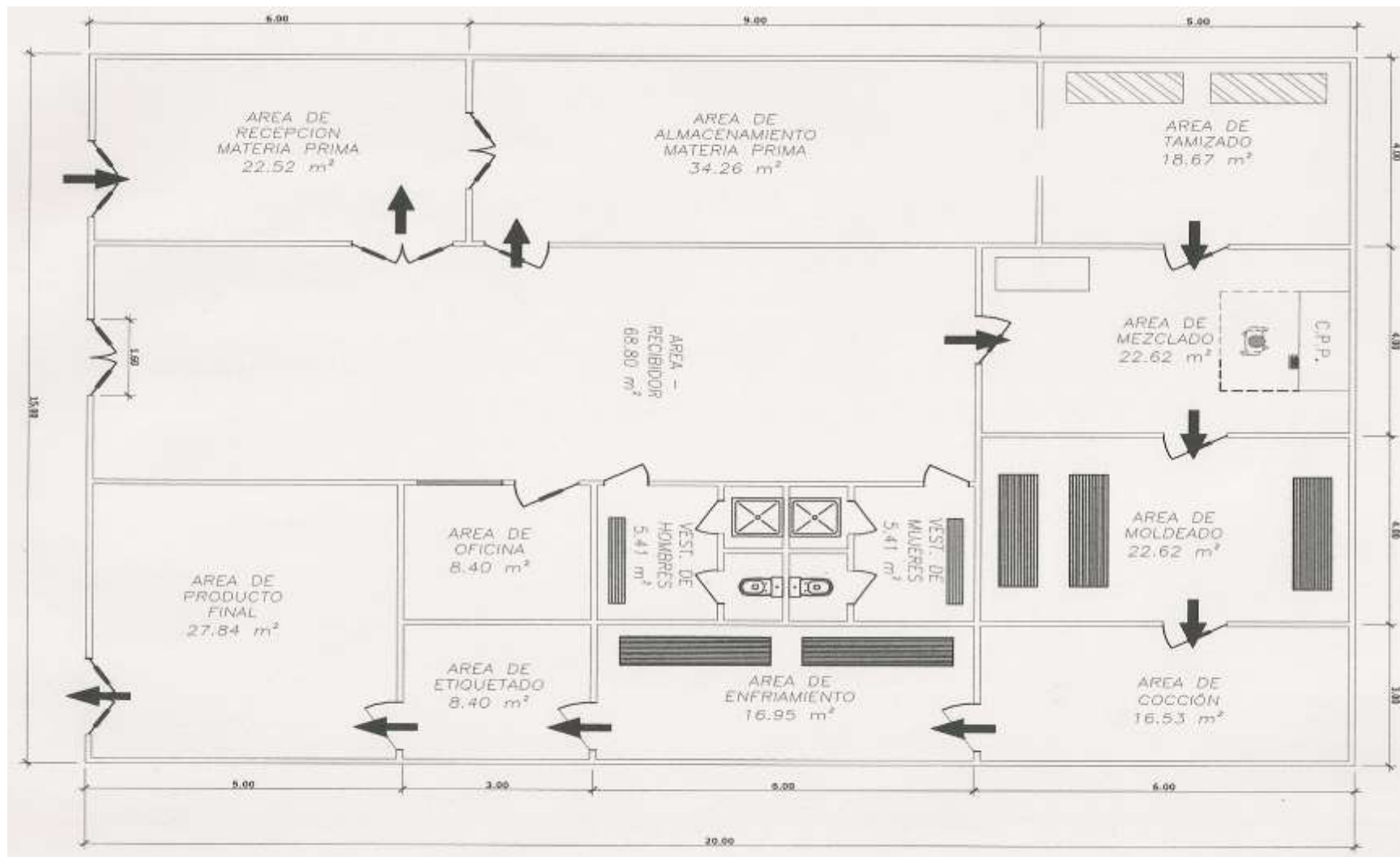
PLANO DE LA PLANTA, VISTA SUPERIOR
