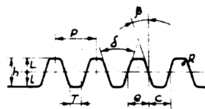
Seccion del filete segun eje
