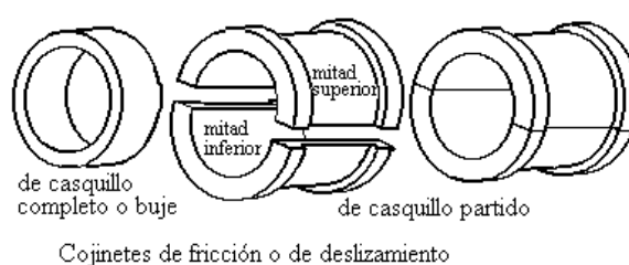
FIGURA 1.26. COJINETES DE DESLIZAMIENTO
