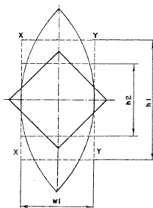
FIGURA 3.2. MÉTODO DEL RECTÁNGULO EQUIVALENTE
