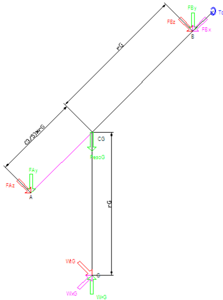
FIGURA 2.20. DIAGRAMA DE CUERPO LIBRE CORONA
