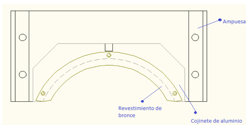
FIGURA 1.30. ESQUEMA DE UBICACIÓN DE MATERIALES EN COJINETE
