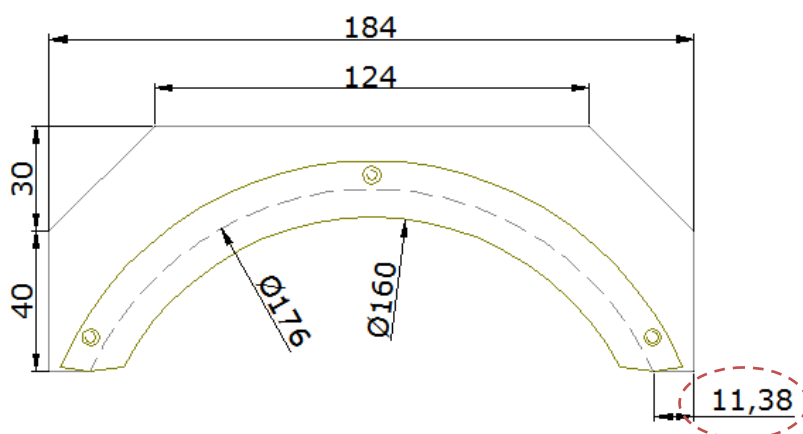
FIGURA 1.33. DIMENSIONES DEL COJINETE
