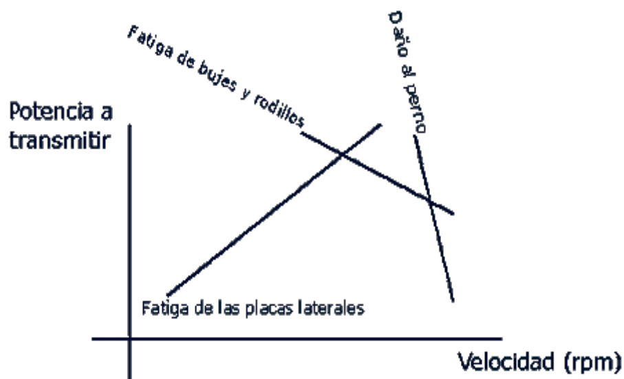
FIGURA 2.9. TIPOS DE FALLAS DE CADENAS.
