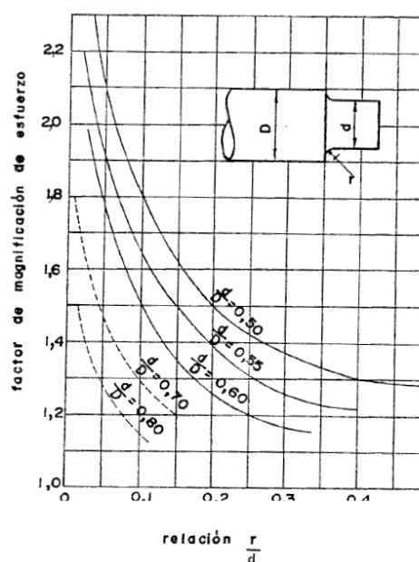
FIGURA 1.7. CURVA PARA DETERMINAR EL FACTOR DE MAGNIFICACIÓN DE ESFUERZOS
