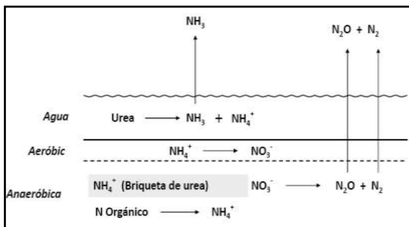
Figura 1.3. Esquema de la aplicación de urea al voleo vs aplicación de briquetas (W. Bowen, 2008).
