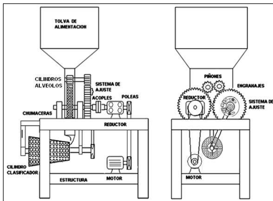
Figura 1.1. Plano general de la maquina Briquetadora (O. Contreras).
