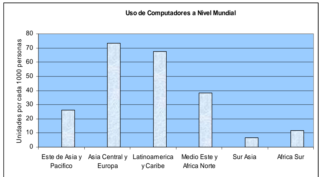
Figura 1.1 Utilización de Computadores en el mundo por zonas. (Datos tomados de International Telecommunication Union's (ITU) Año 2003)
