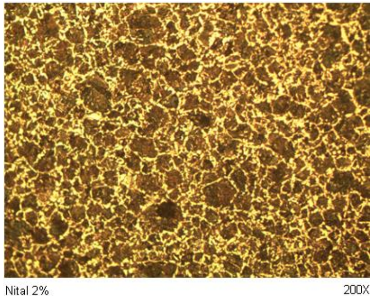
Figura 2.5 Microfotografía con una Ampliación de 200X del Acero ASTM A42
