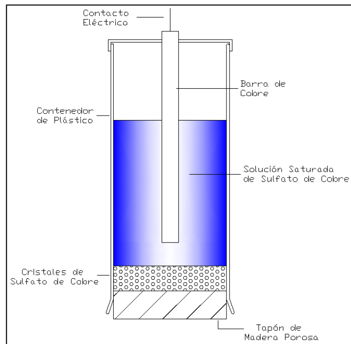
Figura 1.5 Electrodo de Cobre/Sulfato de Cobre.
