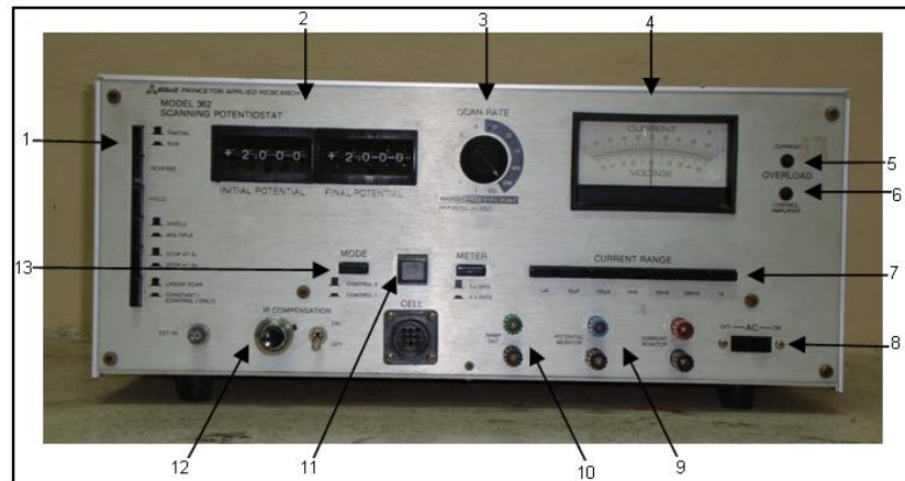
Figura 2.7 Potencio/Galvanostato Modelo 362.
