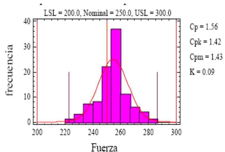
FIGURA 2.8. CAPABILIDAD DE PROCESO PARA UNA FUERZA
