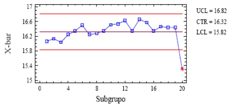
FIGURA 2.17. GRÁFICA X-BAR PARA CEREAL
