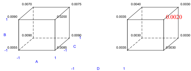
FIGURA 4.4. ANÁLISIS DE CUBO PARA DISMINUIR VARIACIÓN
