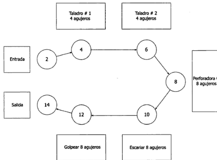
Figura 4-5 Distribución de la celda de manufactura.
