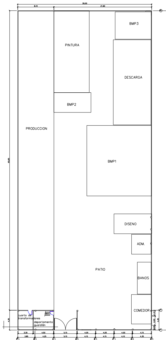
PLANO 4: LAYOUT #3 MÉTODO SPL
