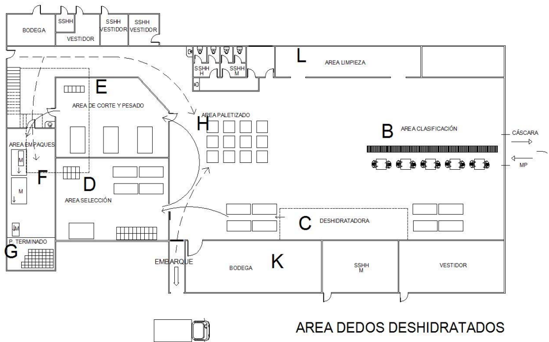
Fig. # 3.5. Layout de la planta
