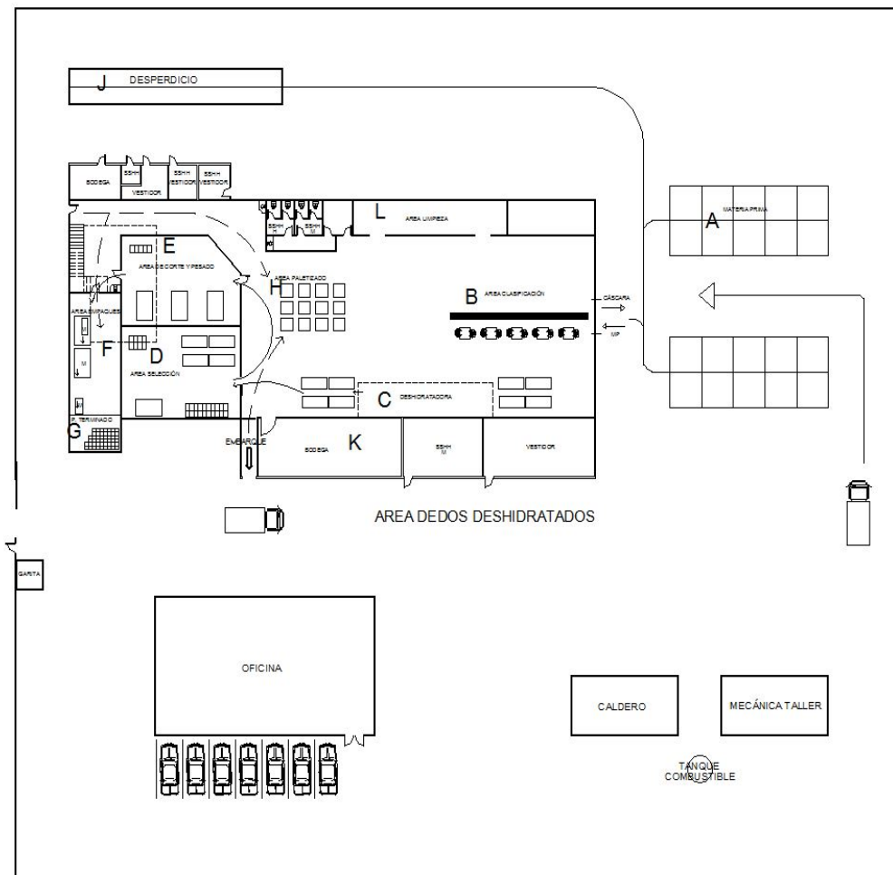
Fig. # 3.4. Layout de la planta
