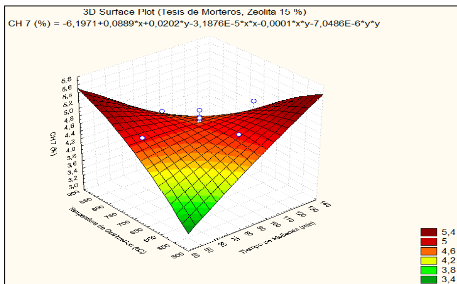
Fig. 5.26 Superficie de Respuesta para CH 7
