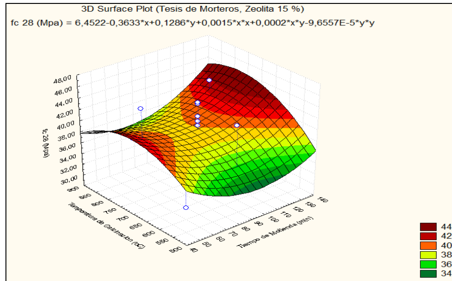
Fig. 5.5 Superficie de Respuesta para fc 28
