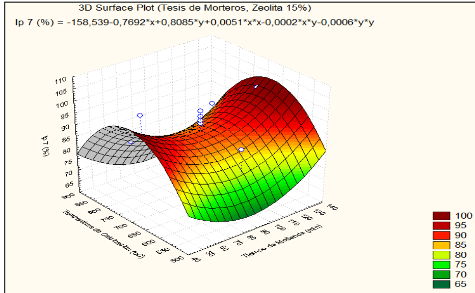
Fig. 5.20 Superficie de Respuesta para Ip 7
