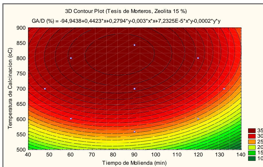
Fig. 5.33 Contornos- Región de Interés para GA/D
