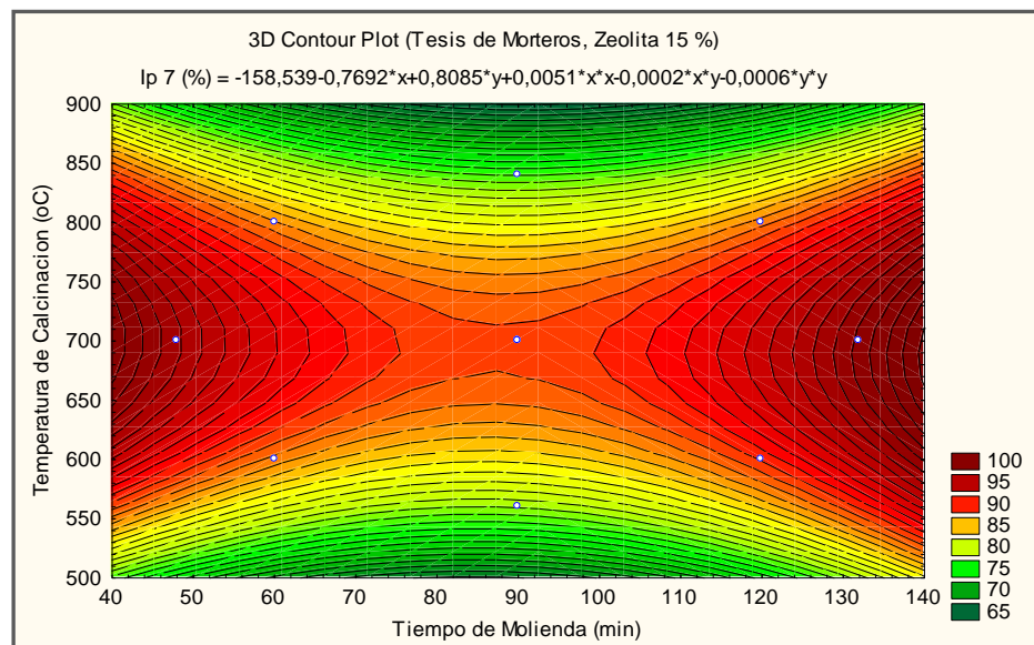
Fig. 5.21 Contornos- Región de Interés para Ip 7
