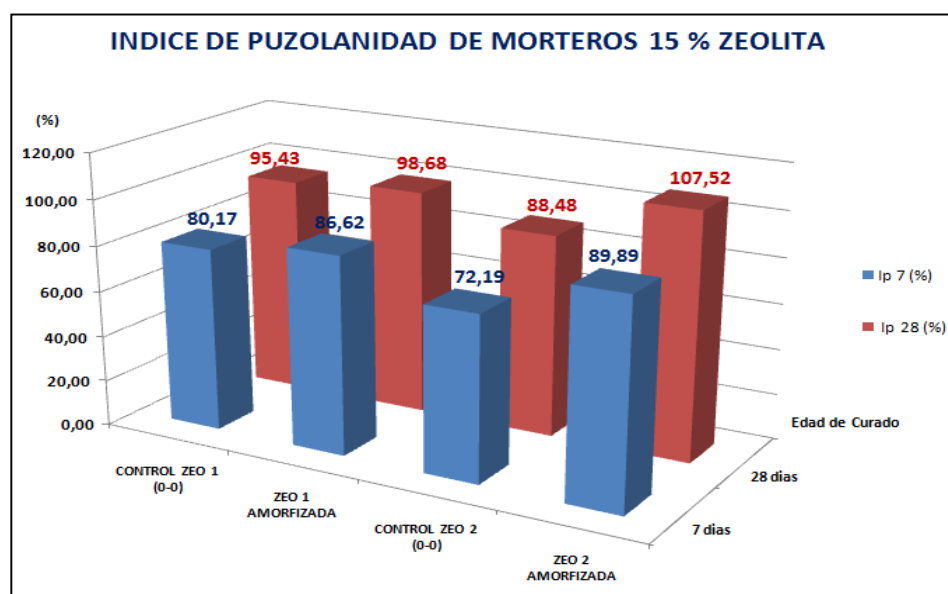
Fig. 5.36 Índice de Puzolanidad de Morteros 15 % Zeolita
