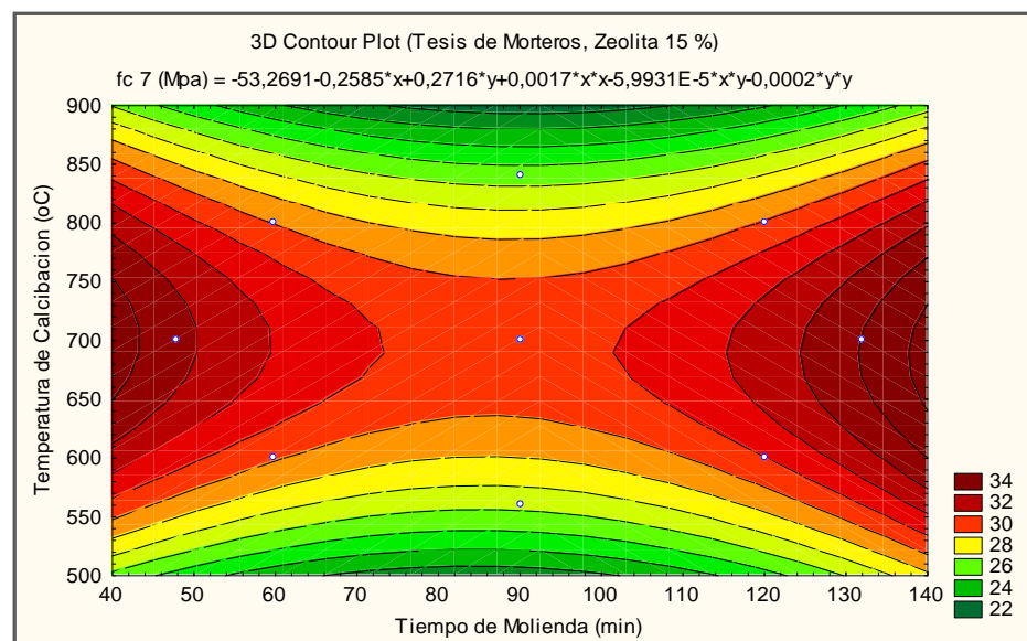
Fig. 5.3 Contornos- Región de Interés para f_c 7
