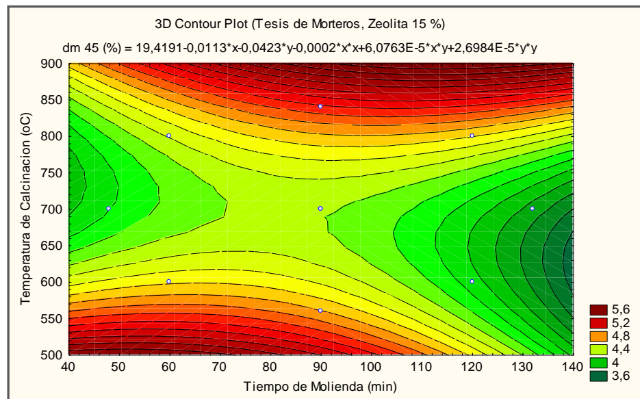
Fig. 5.18 Contornos- Región de Interés para dm 45
