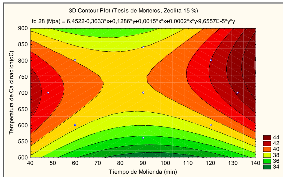
Fig. 5.6 Contornos- Región de Interés para fc 28
