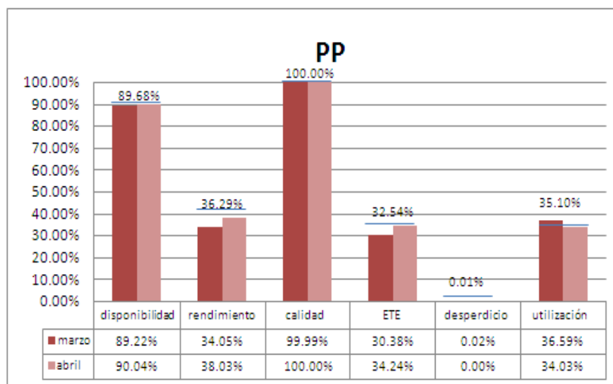
FIGURA 6.13. VALORES DE INDICADORES MES DE MARZO Y ABRIL DE LA PLEGADORA PESADA
