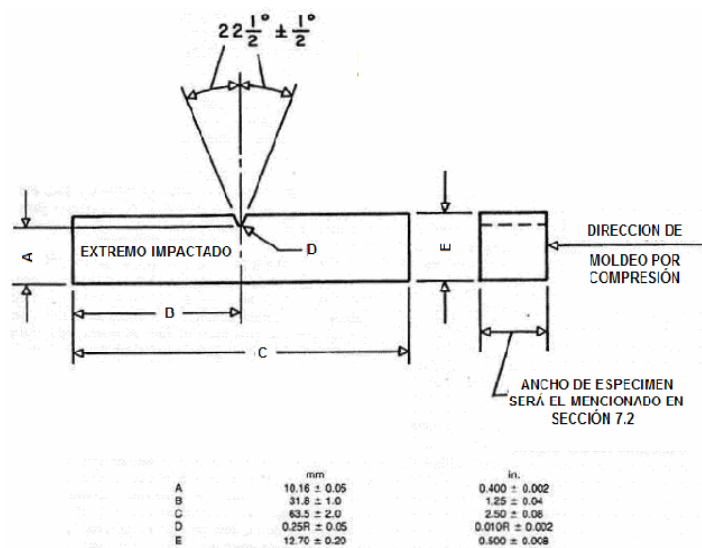
FIGURA 3.11 DIMENSIONES DE UN ESPÉCIMEN DE PRUEBA TIPO IZOD
