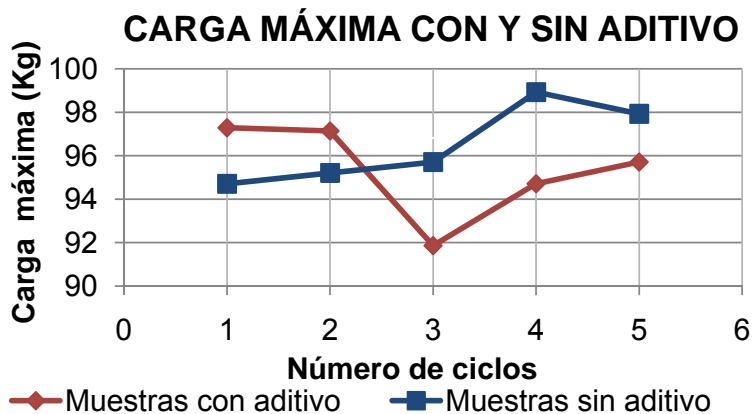
FIGURA 5.5 CARGA MÁXIMA EN 5 CICLOS CON Y SIN ADITIVO
