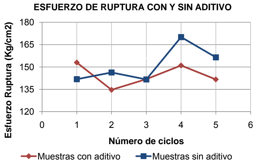
FIGURA 5.7 ESFUERZOS DE RUPTURA EN 5 CICLOS CON Y SIN ADITIVO
