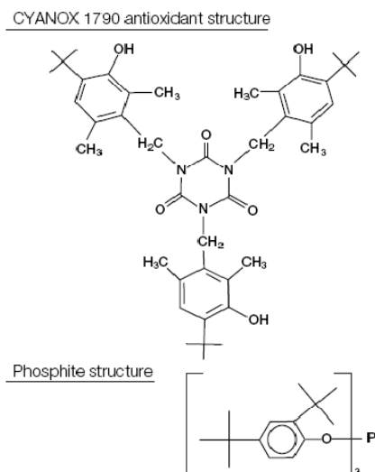
FIGURA 2.4 ESTRUCTURA DEL CYANOX 1790 EN BASE DE FOSFITO
