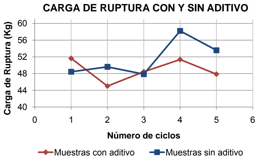
FIGURA 5.8 CARGAS DE RUPTURAS EN 5 CICLOS CON Y SIN ADITIVO
