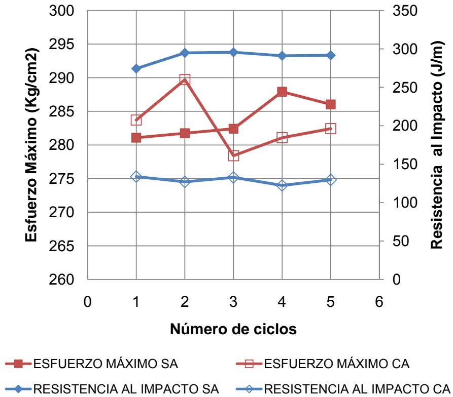
FIGURA 5.12 RESISTENCIA AL IMPACTO Y ESFUERZO MÁXIMO EN COMPARACIÓN CON LOS 5 CICLO DE INYECCIÓN.
