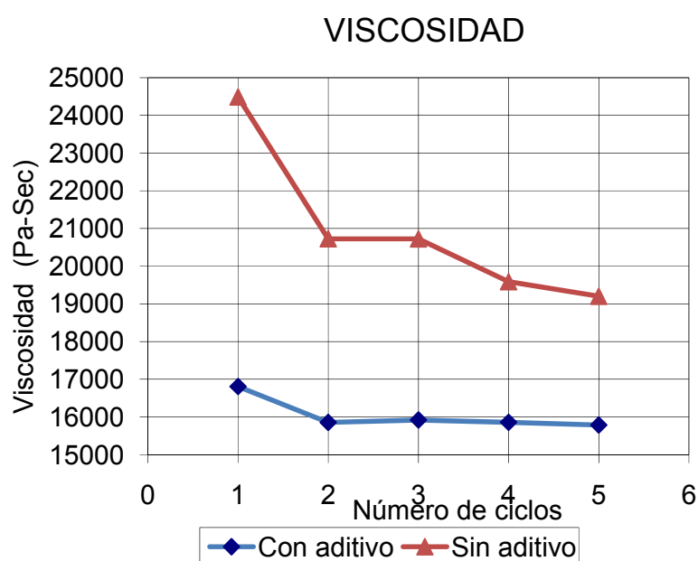
FIGURA 5.2 VISCOSIDAD
