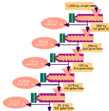
FIGURA 2.3 LAZO CONTINUO DE SCRAP
