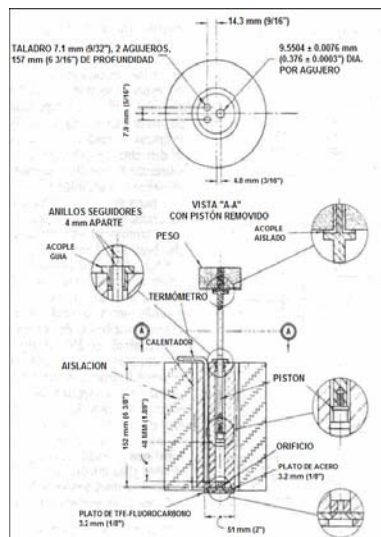
FIGURA 3.6 ESQUEMA DE LA MÁQUINA DE MFI
