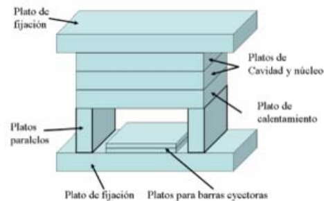
FIGURA 2.11 DISEÑO DE MOLDE
