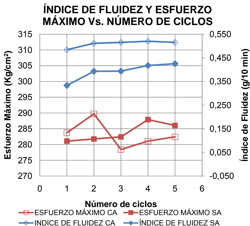
FIGURA 5.11 ÍNDICE DE FLUIDEZ Y ESFUERZO MÁXIMO EN COMPARACIÓN CON LOS 5 CICLOS DE INYECCIÓN
