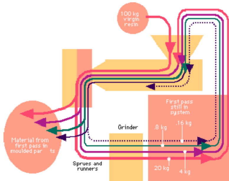
FIGURA 2.2 LAZO CONTINUO DE SCRAP Y RESINA
