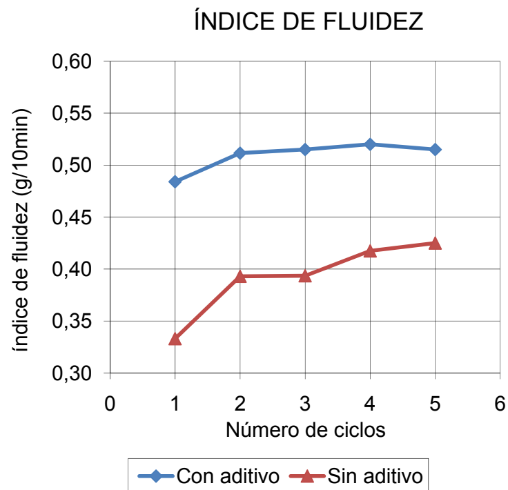
FIGURA 5.1 ÍNDICE DE FLUIDEZ EN 5 CICLOS CON Y SIN ADITIVO
