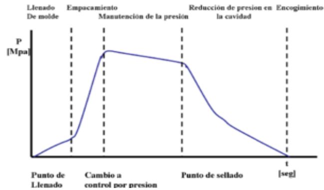
FIGURA 2.12 LLENADO DE MOLDE POR INYECCIÓN.
