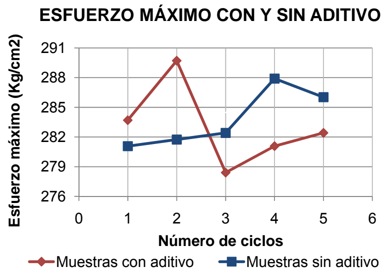
FIGURA 5.6 ESFUERZOS MÁXIMOS EN 5 CICLOS CON Y SIN ADITIVO
