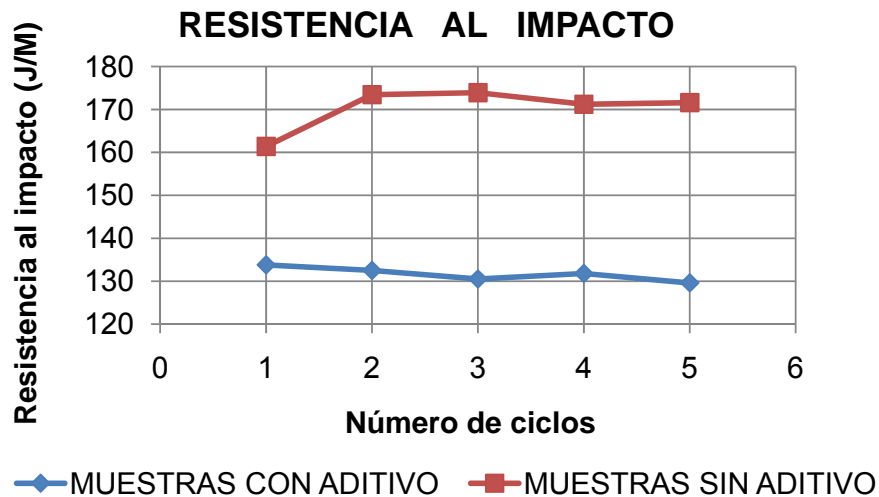
FIGURA 5.4 RESISTENCIA AL IMPACTO
