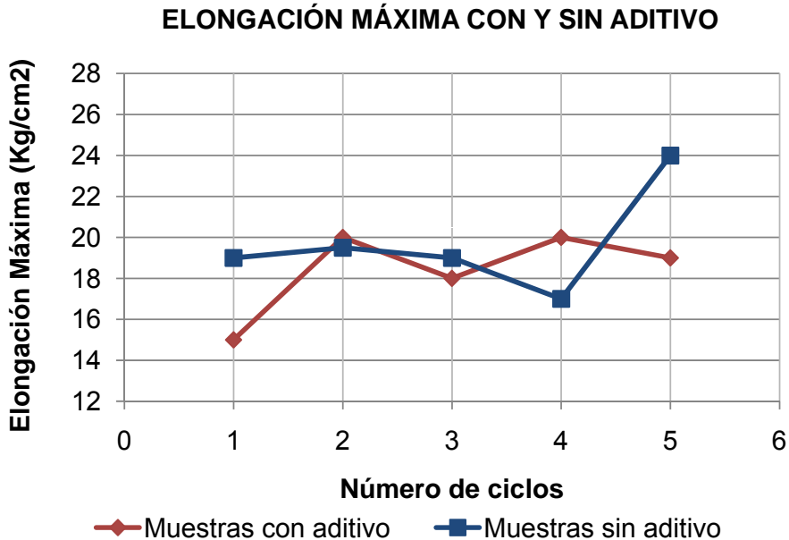
FIGURA 5.9 ELONGACIONES EN 5 CICLOS CON Y SIN ADITIVO
