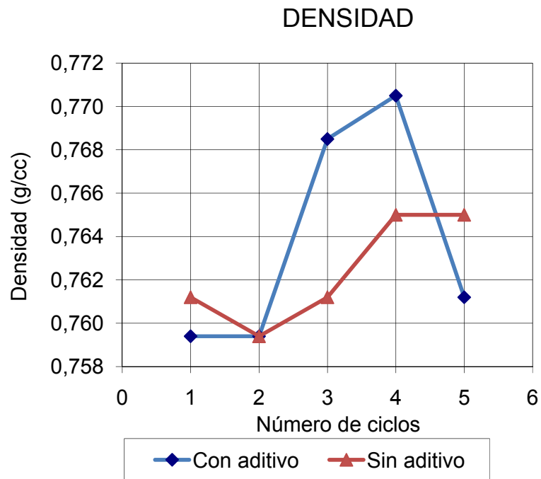
FIGURA 5.3 DENSIDAD EN CINCO CICLOS CON Y SIN ADITIVO
