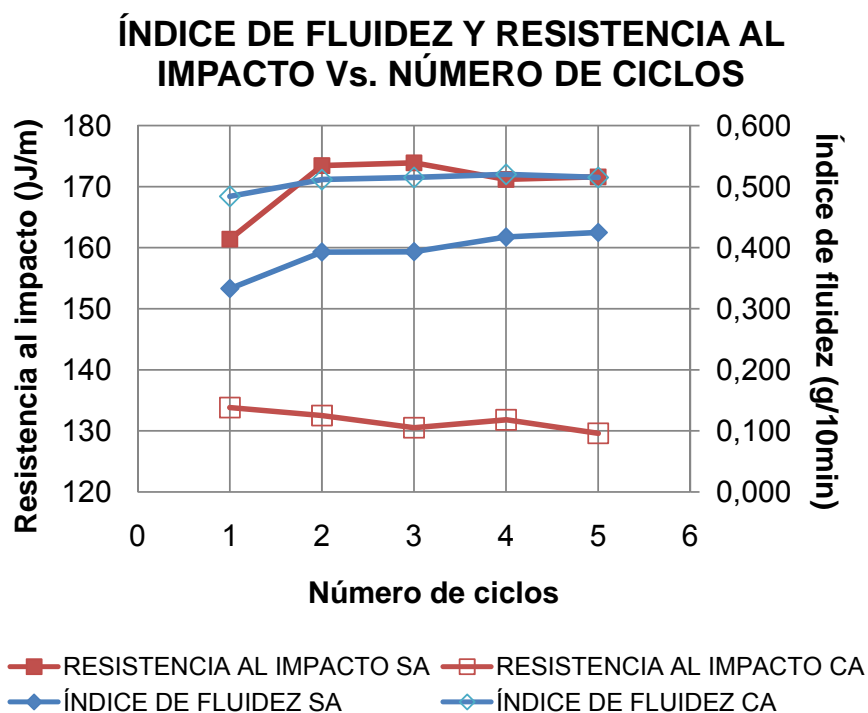
FIGURA 5.10 ÍNDICE DE FLUIDEZ Y RESISTENCIA AL IMPACTO EN COMPARACIÓN CON LOS 5 CICLOS DE INYECCIÓN.
