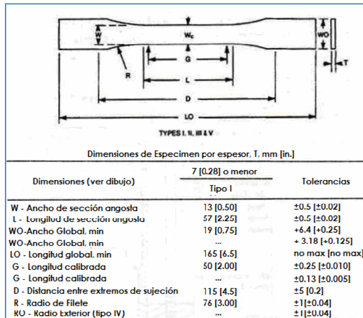
FIGURA 3.14 ESPÉCIMEN DE PRUEBA Y MEDIDAS
