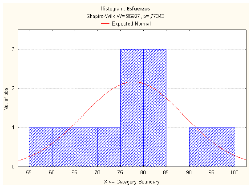
FIGURA 4.8. HISTOGRAMA DE ESFUERZOS AL 22.5% DE ZEOLITA 2
