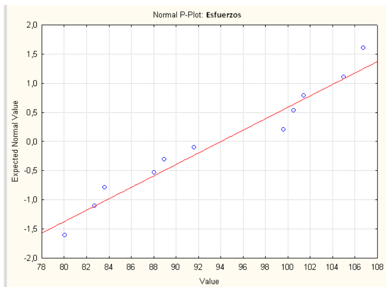
FIGURA 4.5. NORMALIZACIÓN DE ESFUERZOS AL 20% DE ZEOLITA
