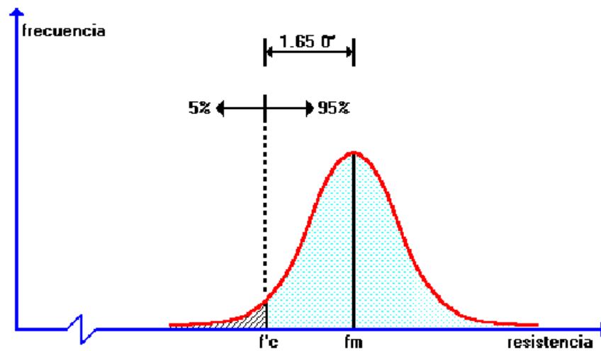
FIGURA 2.2. DISTRIBUCIÓN NORMALIZADA DE LOS ENSAYOS DE ROTURA [17]
