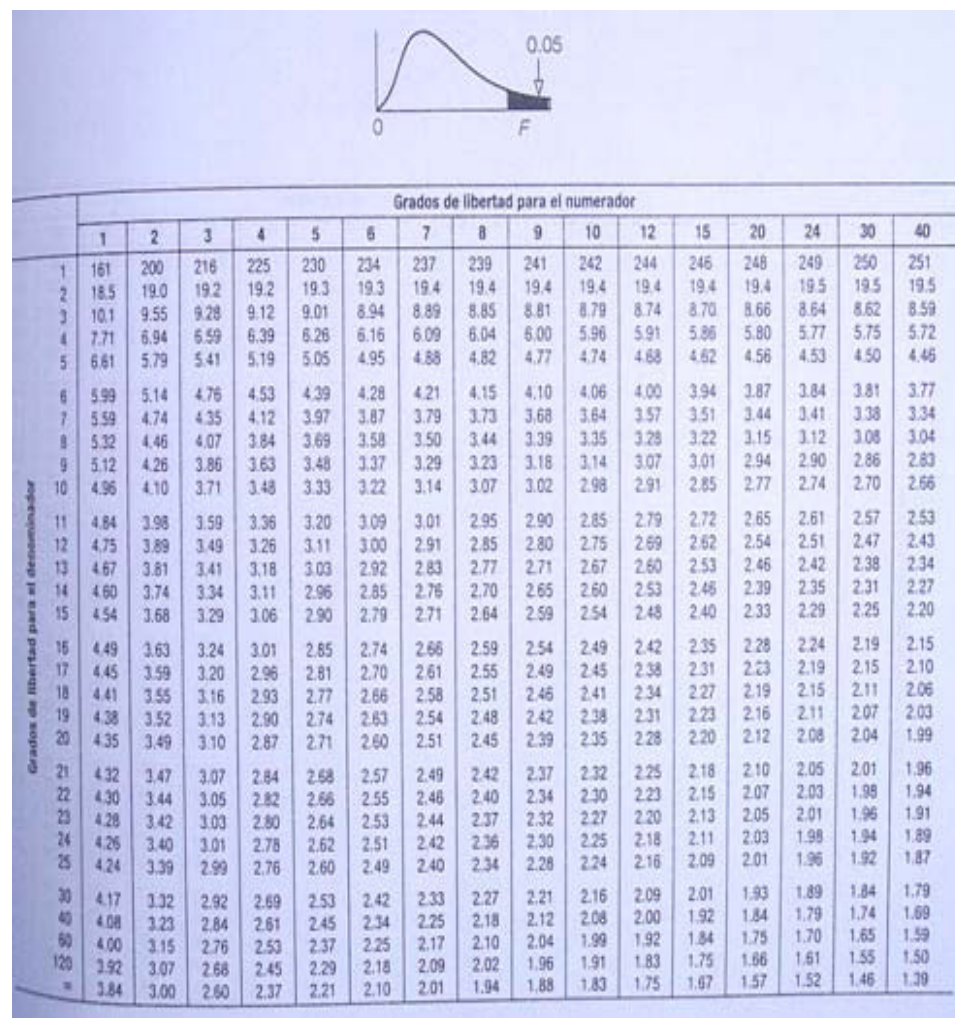
FIGURA 2.4 VALORES CRÍTICOS DE LA DISTRIBUCIÓN F
