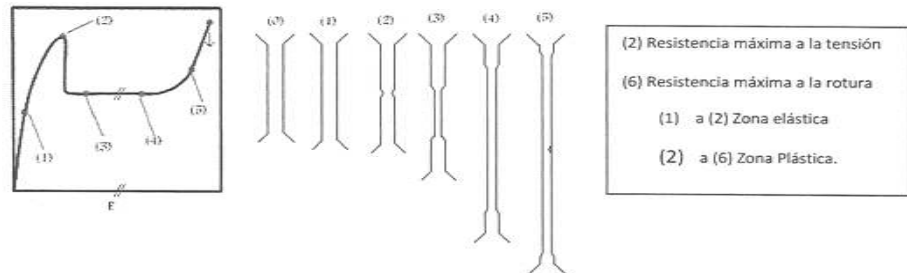
FIGURA 2.5 GRÁFICA ESFUERZO VS DEFORMACIÓN
