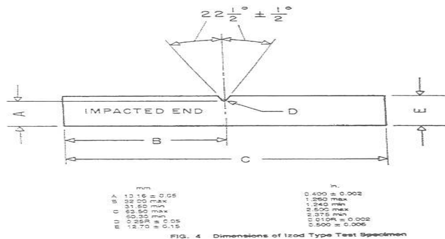
FIGURA 2.8 DIMENSIONES DE LA PROBETA PARA EL ENSAYO IZOD.
