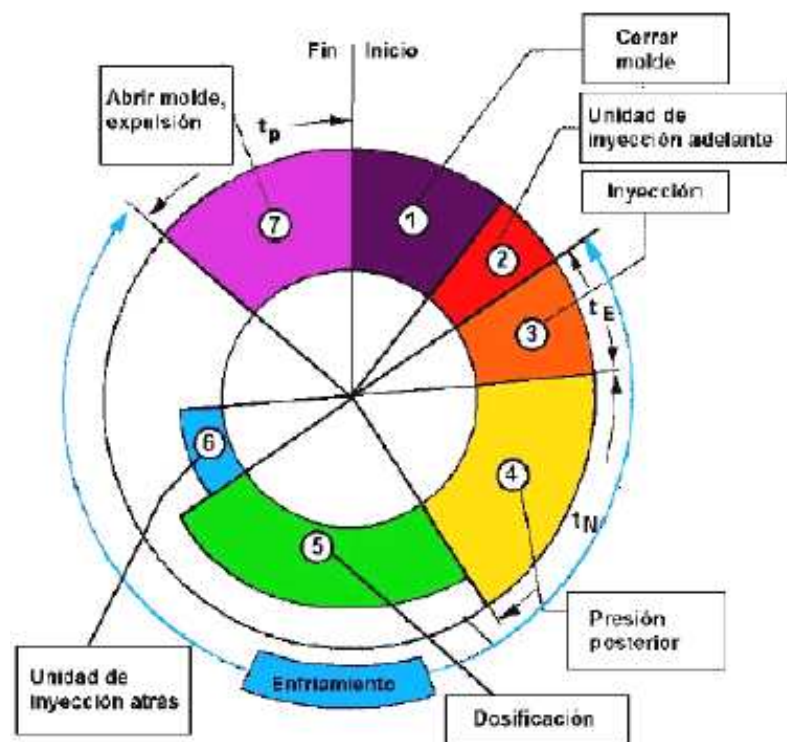
FIGURA 2.2 CICLO DE INYECCIÓN
