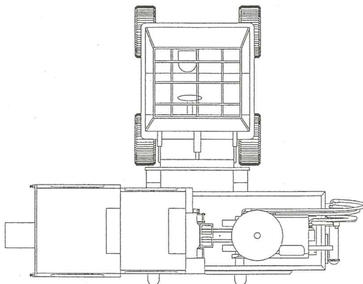
FIGURA 4.1 APLICACIÓN DE MONTACARGAS A LA INYECTORA
