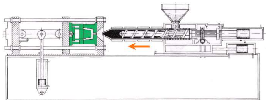
FIGURA 2.1 ESQUEMA BÁSICO DE MÁQUINA DE INYECCIÓN
