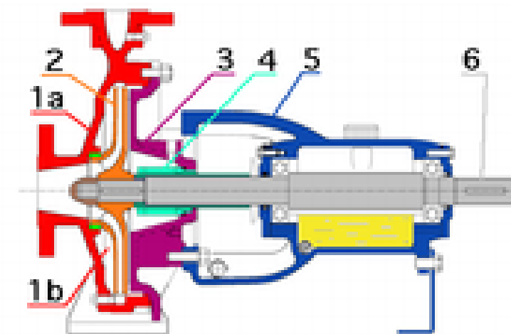
FIGURA 3.10. CORTE ESQUEMÁTICO DE UNA BOMBA CENTRÍFUGA.
