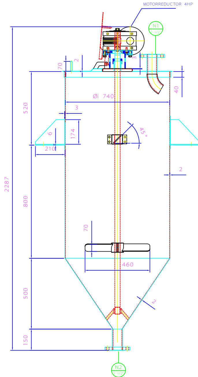
ELEVACION
