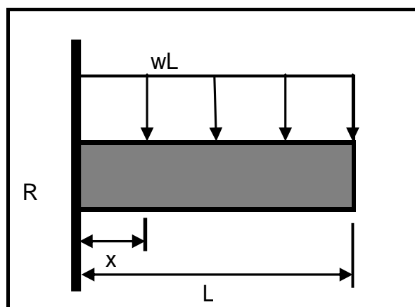
FIGURA 3.3. VIGA EN VOLADIZO CON CARGA UNIFORME
