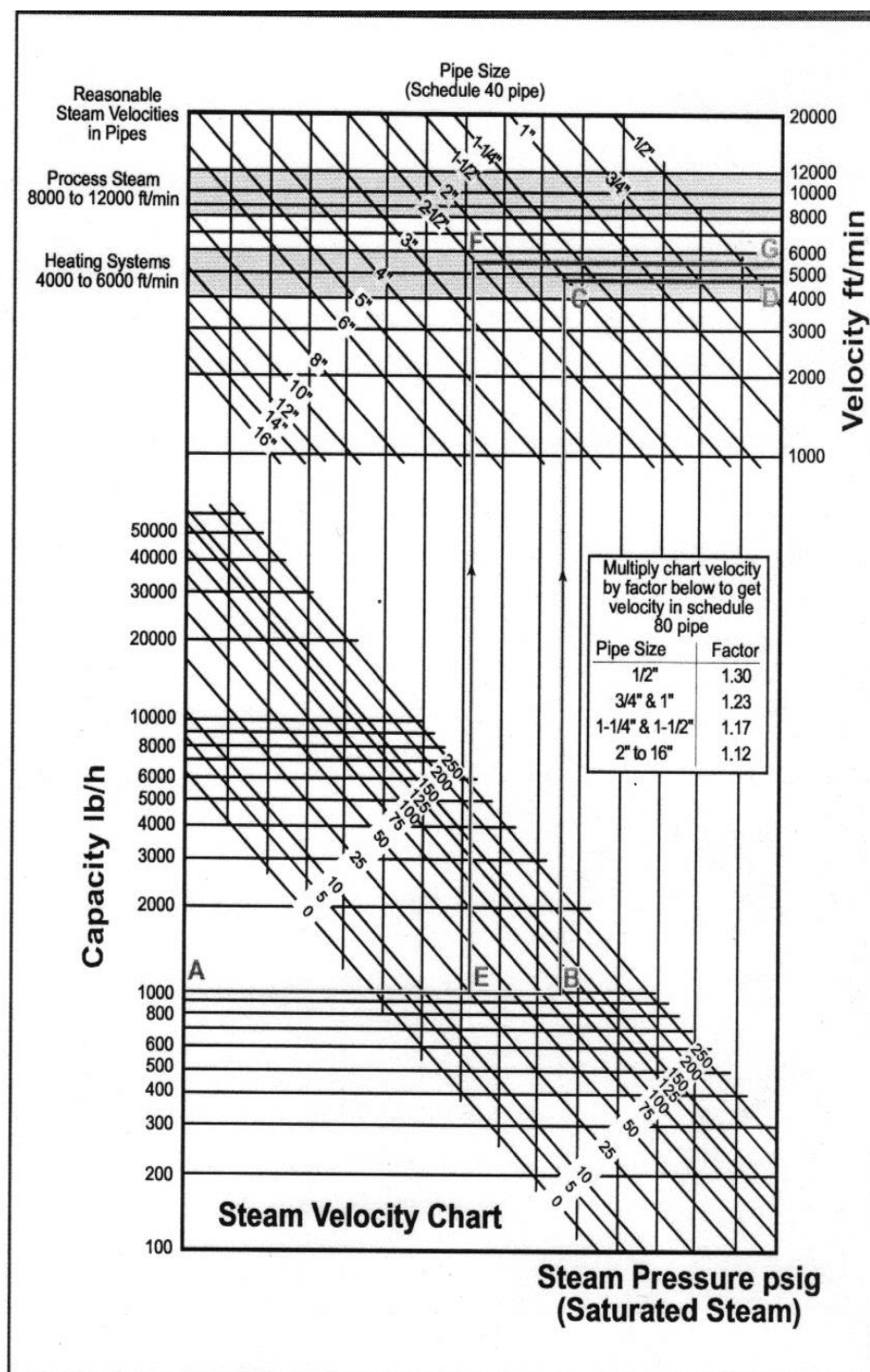
FIGURA 3.13. DIAGRAMA VELOCIDAD DE VAPOR
