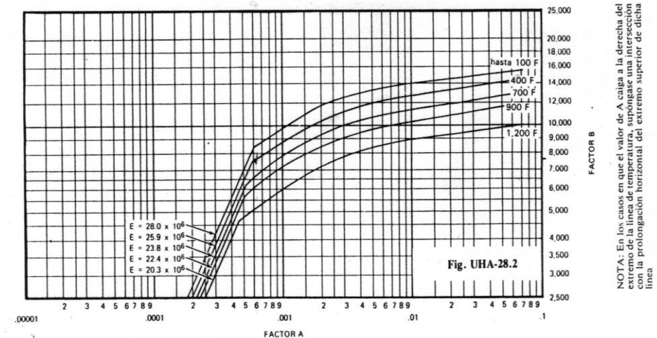
FIGURA 3.7. VALORES DEL FACTOR B QUE SE EMPLEAN EN LAS FORMULAS PARA RECIPIENTES SUJETOS A PRESIÓN EXTERNA (CASO ACERO AUSTENÍTICO 316)
