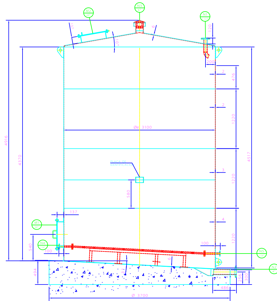
ELEVACION
