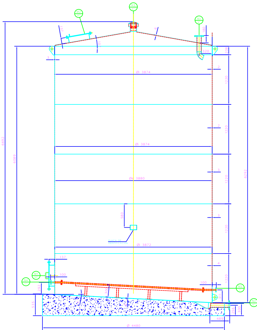
ELEVACION
