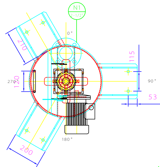
ORIENTACION
