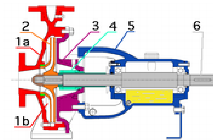
FIGURA 3.10. CORTE ESQUEMÁTICO DE UNA BOMBA CENTRÍFUGA.
