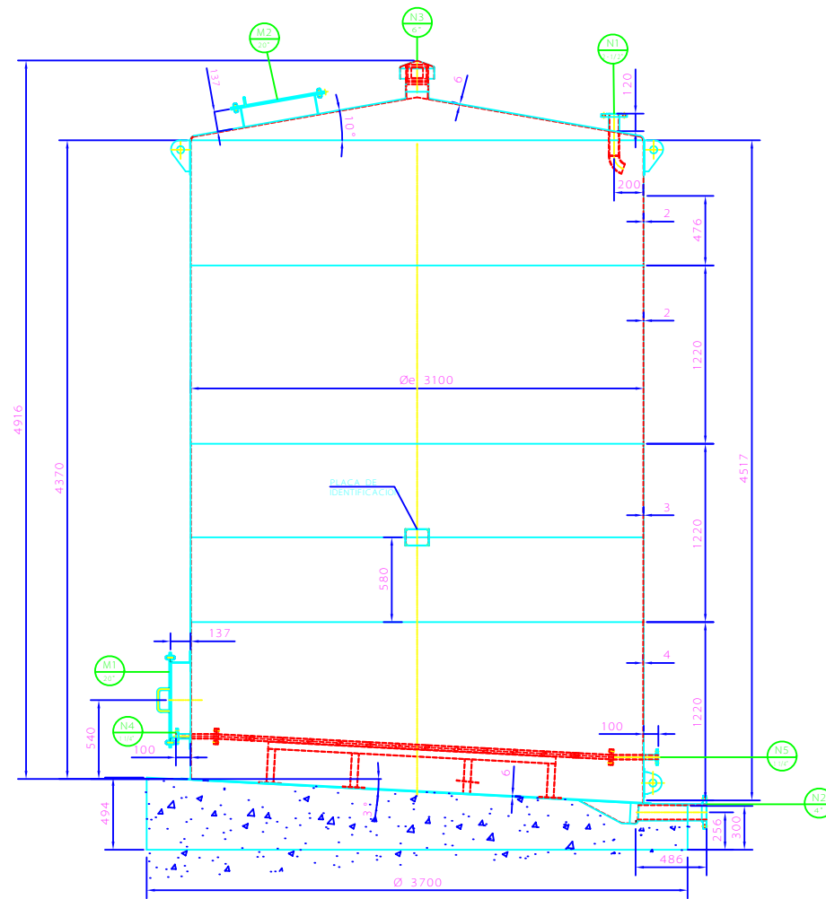
ELEVACION
