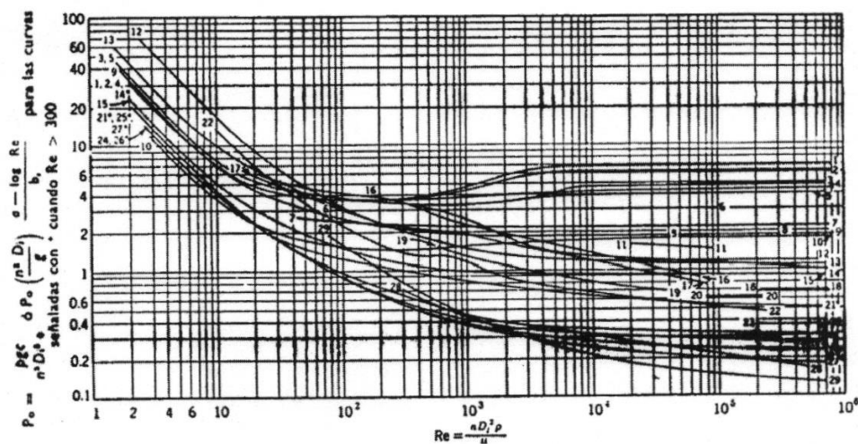
FIGURA 3.5. NÚMERO DE POTENCIA VS REYNOLDS PARA VARIOS TIPOS DE AGITADORES
