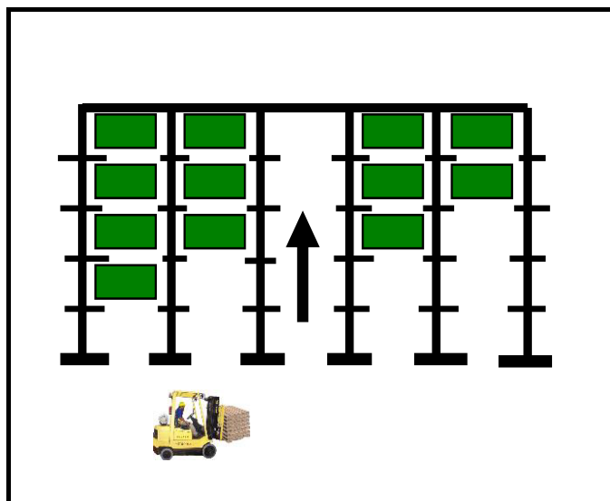
FIGURA 3.20. ESTANTERÍA CON ACCESO EN UN SOLO SENTIDO
