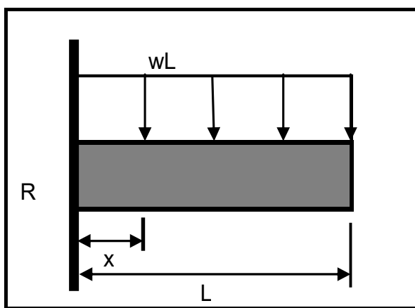
FIGURA 3.3. VIGA EN VOLADIZO CON CARGA UNIFORME
