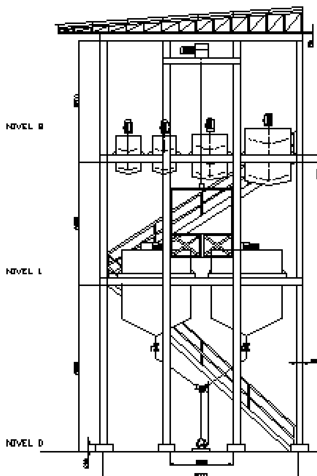
FIGURA 3.8. ESQUEMA DE TORRE FABRICACIÓN
