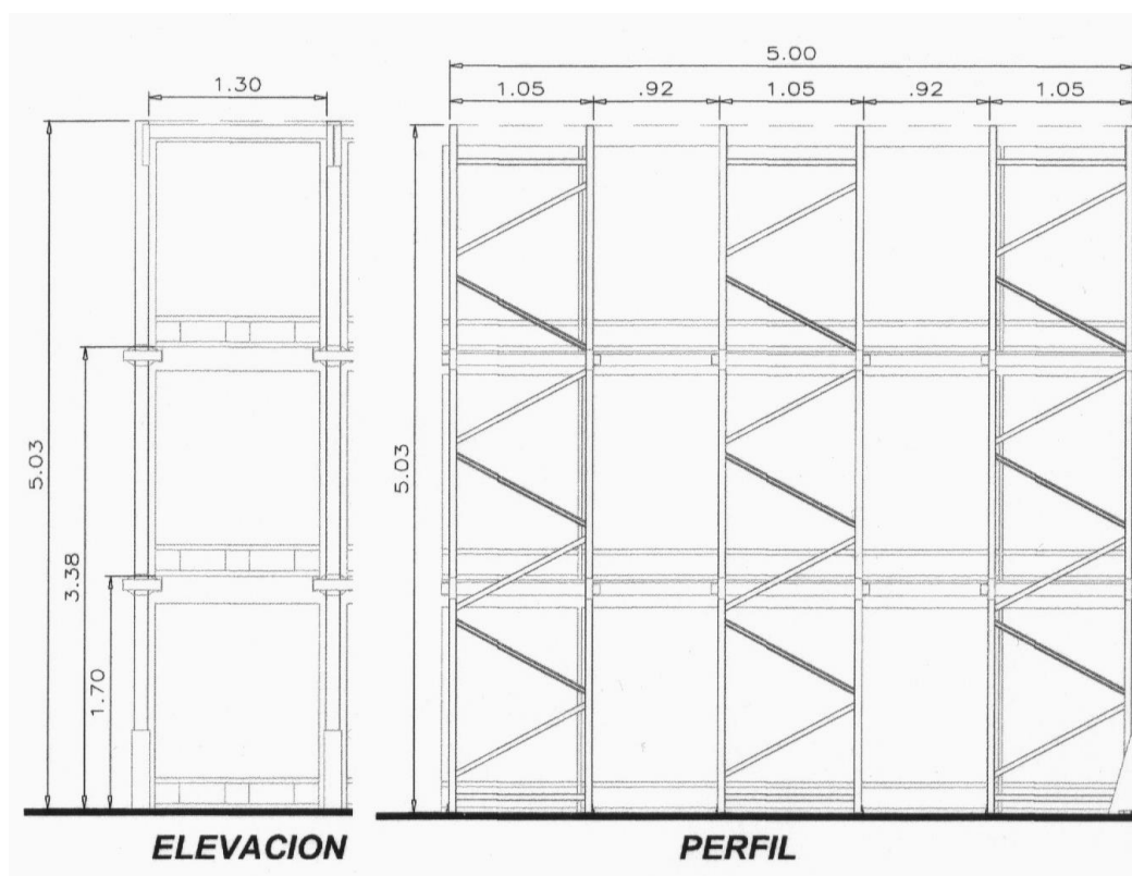
FIGURA 3.25. ESQUEMA DE SISTEMA DE ALMACENAMIENTO SELECCIONADO
