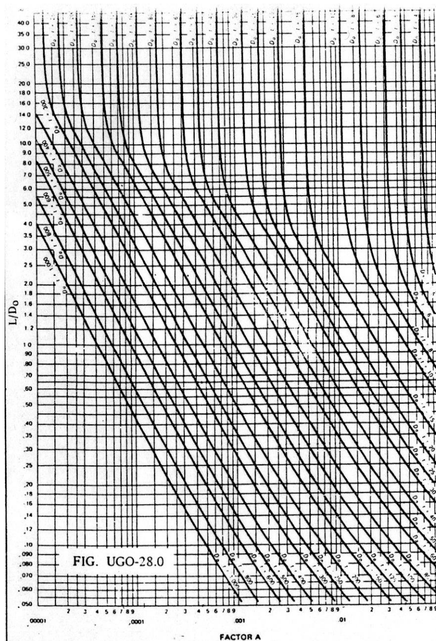
FIGURA 3.6. VALORES DEL FACTOR A QUE SE USAN EN LAS FORMULAS PARA RECIPIENTES SOMETIDOS A PRESIÓN EXTERNA
