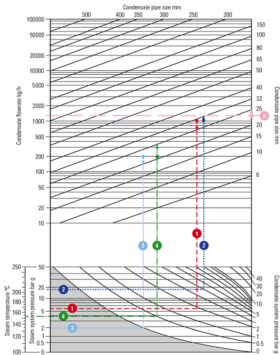
FIGURA 3.15. DIAGRAMA PARA DIMENSIONAMIENTO DE TUBERÍA DE CONDENSADO
