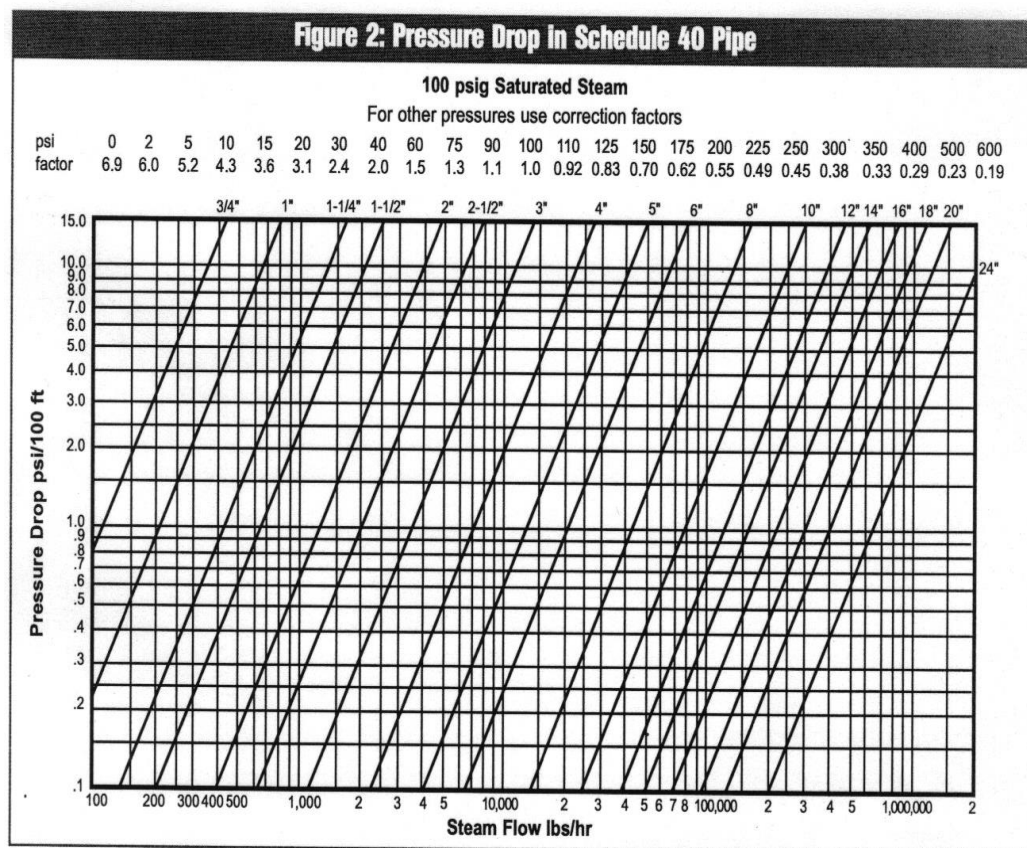
FIGURA 3.14. CAÍDAS DE PRESIÓN EN TUBERÍA DE VAPOR CÉDULA 40
