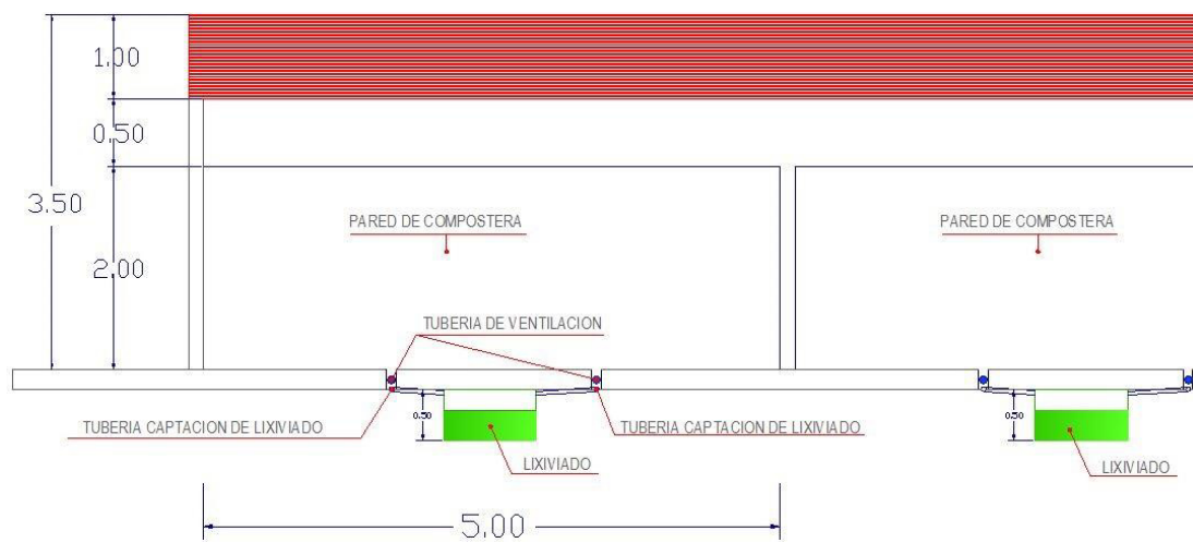
FIGURA 23. Corte A-A' de la planta de compostaje.
