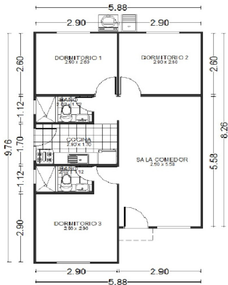
FIGURA 15. Villa modelo de 55.45 m 2 .
