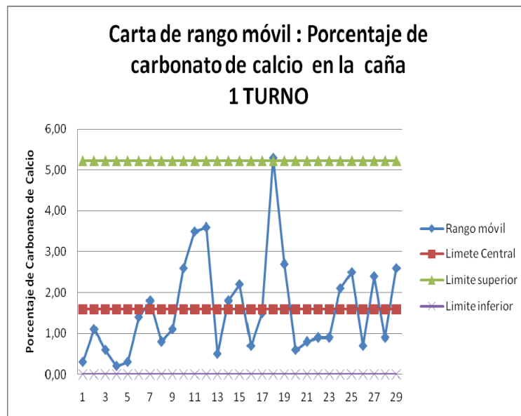
Figura 3.9 : Carta de control de rangos móviles, botas de PVC, Porcentaje de carbonato de calcio en la caña, 1 turno.
