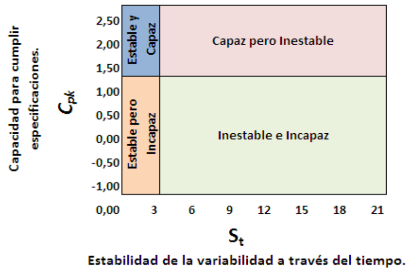
Figura 2.5: Estado de un proceso.
