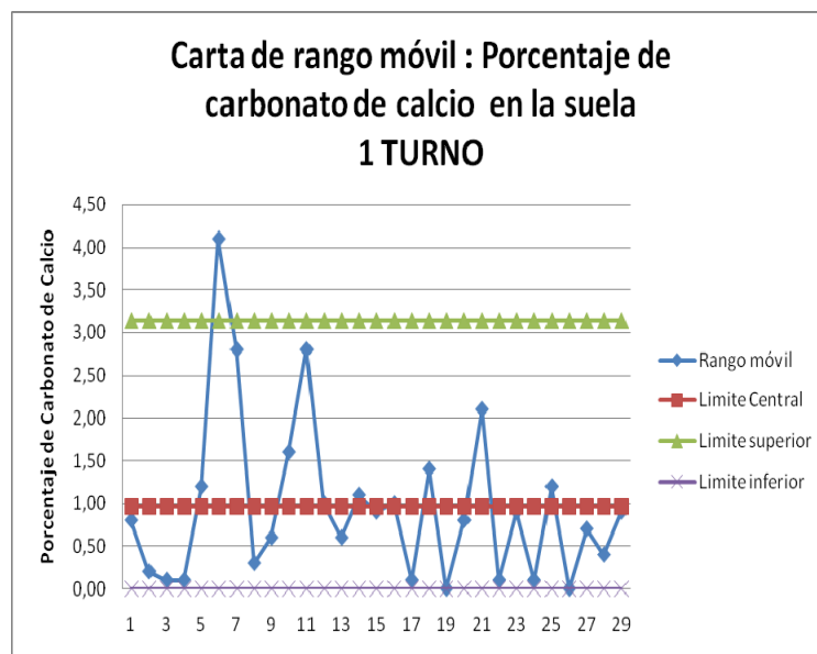
Figura 3.7 : Carta de control de rangos móviles, botas de PVC, Porcentaje de carbonato de calcio en la suela, 1 turno.
