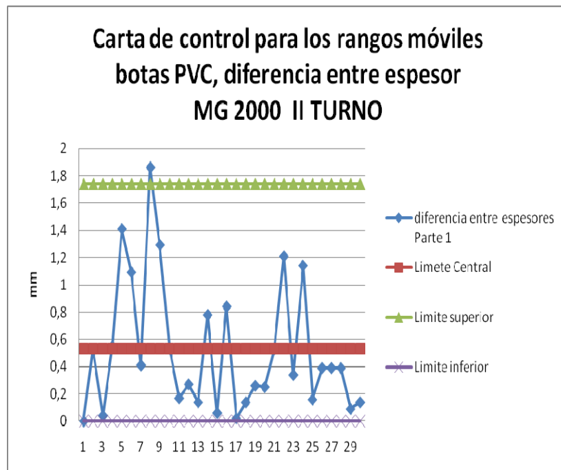
Figura 3.29: Carta de control de rangos móviles, II parte bota izquierda, diferencia entre espesor. Máquina MG 2000 II turno.
