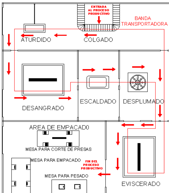
FIGURA 4.8. Alternativa 1- SLP del departamento de Producción
