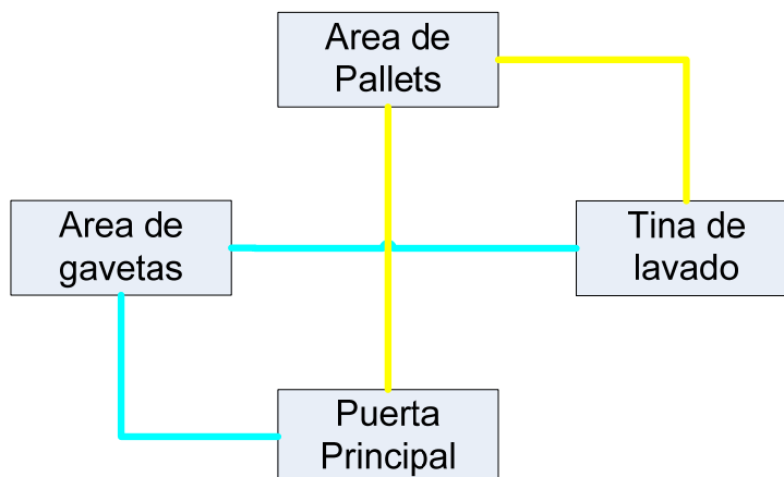
FIGURA 4.27. Diagrama de relaciones-SLP de la Bodega de gavetas y pallets.
