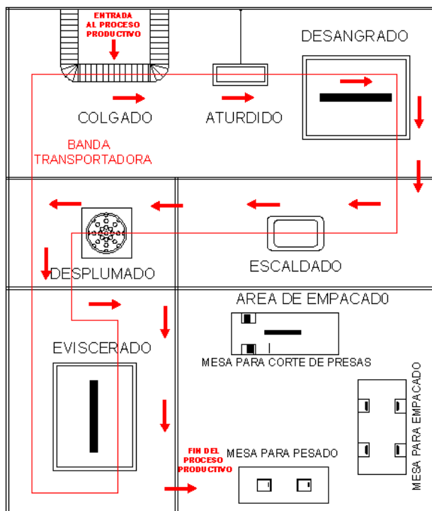
FIGURA 4.10. Alternativa 3- SLP del departamento de Producción.
