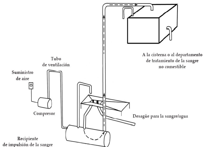
FIGURA 3.31. Representación de la recolección de residuos líquidos.
