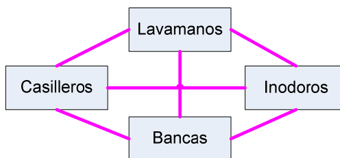
FIGURA 4.39. Diagrama de relaciones-SLP del Área de vestidores.
