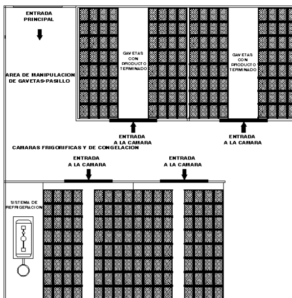
FIGURA 4.34. Alternativa 3-SLP de la Bodega de producto terminado.
