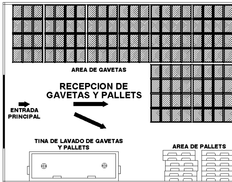
FIGURA 4.9. Alternativa 2-SLP de la Bodega de gaveta y pallets.
