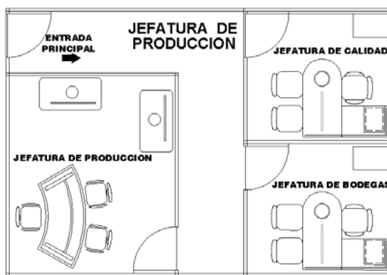
FIGURA 4.20. Alternativa 1 - SLP de la Jefatura de Producción.
