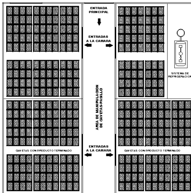
FIGURA 4.33. Alternativa 2-SLP de la Bodega de producto terminado.
