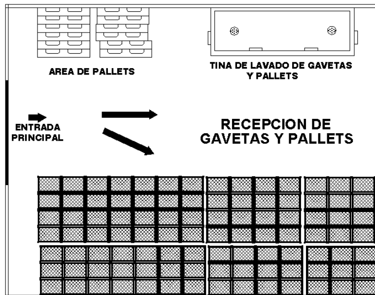
FIGURA 4.30. Alternativa 3-SLP de la Bodega de gavetas y pallets.
