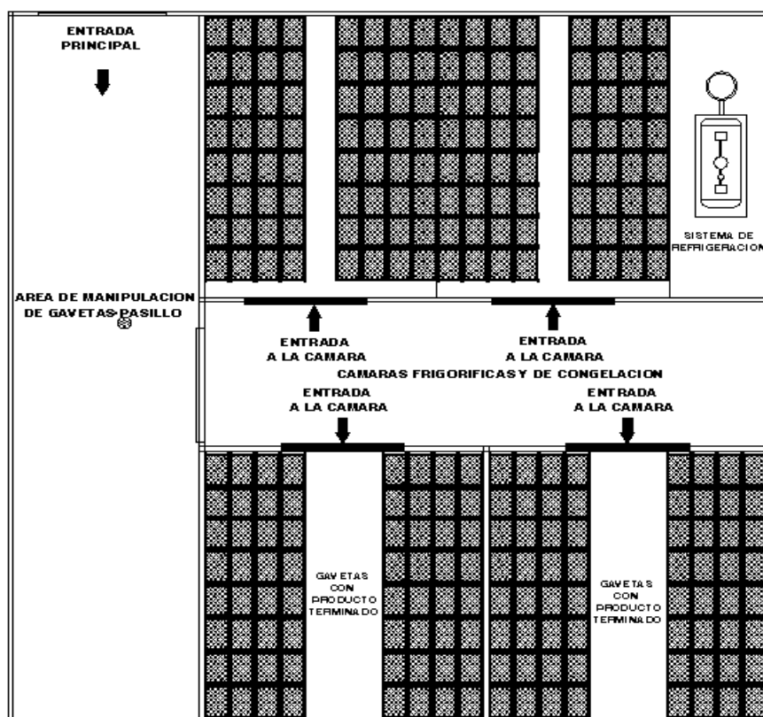
FIGURA 4.32. Alternativa 1-SLP de la Bodega de producto terminado.
