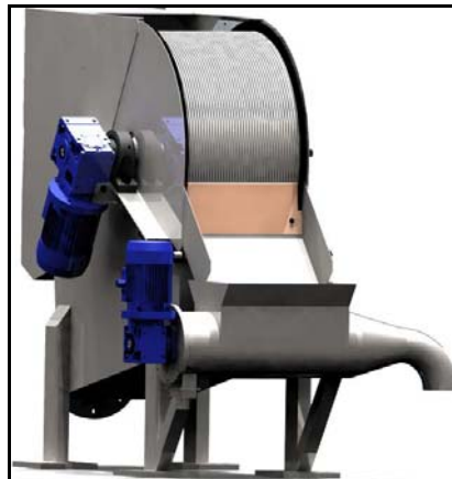
FIGURA 3.33. Maquina tamizadora
