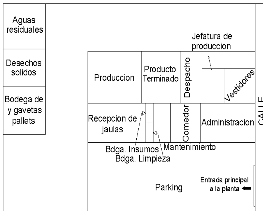
FIGURA 4.4. Alternativa 1 para la elección del Block Layout final.
