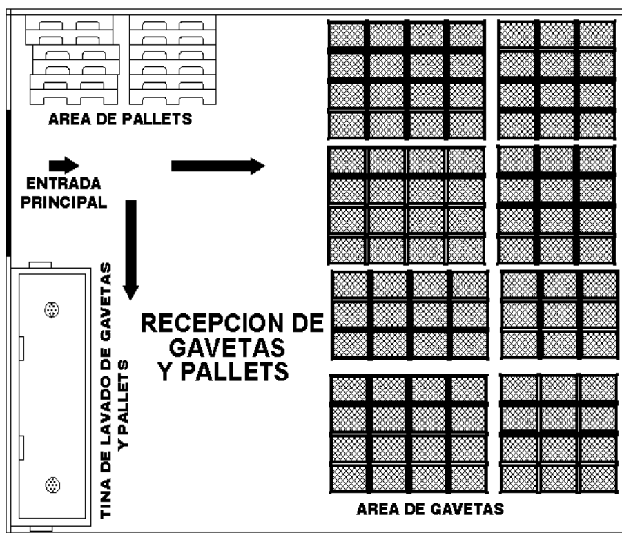
FIGURA 4.28. Alternativa 1-SLP de la Bodega de gavetas y pallets.
