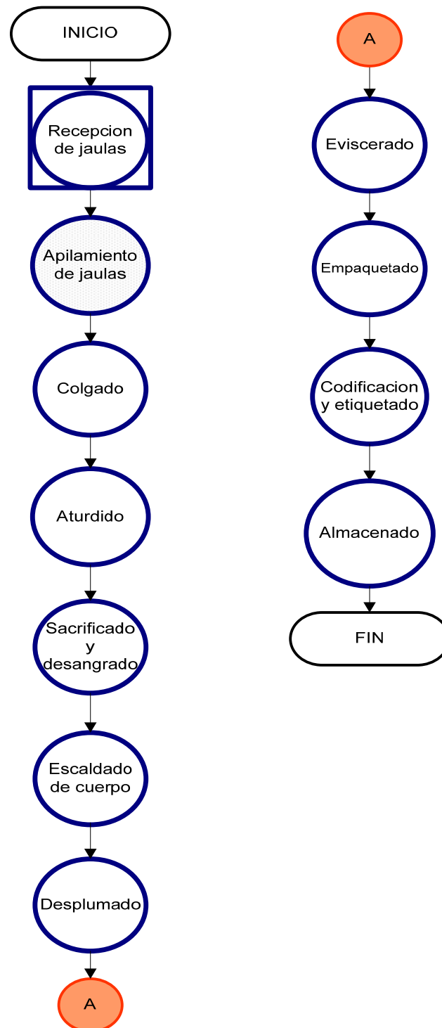
FIGURA 3.20. Diagrama de operaciones del proceso productivo.
