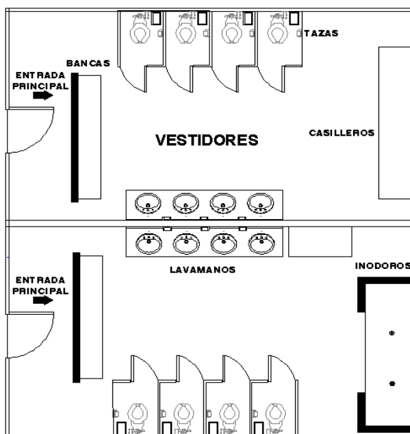
FIGURA 4.42. Alternativa 3-SLP del Área de vestidores.
