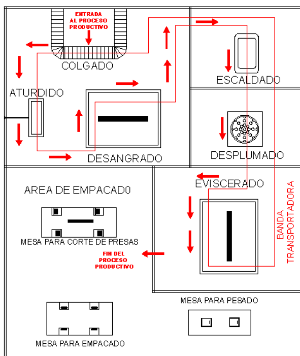
FIGURA 4.9. Alternativa 2- SLP del departamento de Producción.
