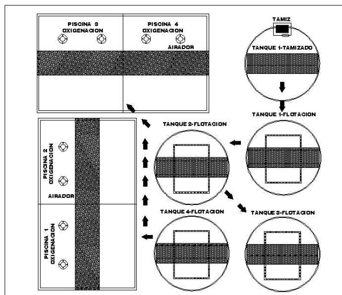
FIGURA 4.13. Alternativa 2- Área de tratamiento de aguas residuales.
