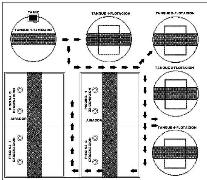
FIGURA 4.12. Alternativa 1- Área de tratamiento de aguas residuales.
