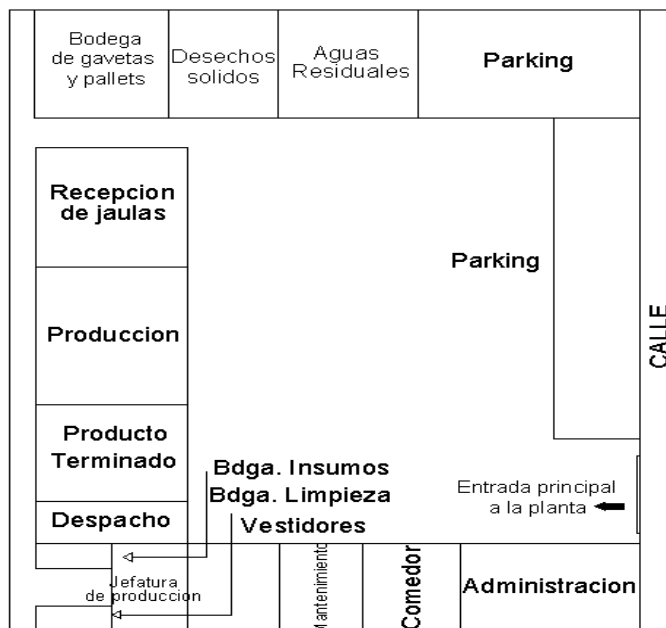
FIGURA 4.5. Alternativa 2 para la elección del Block Layout Final.
