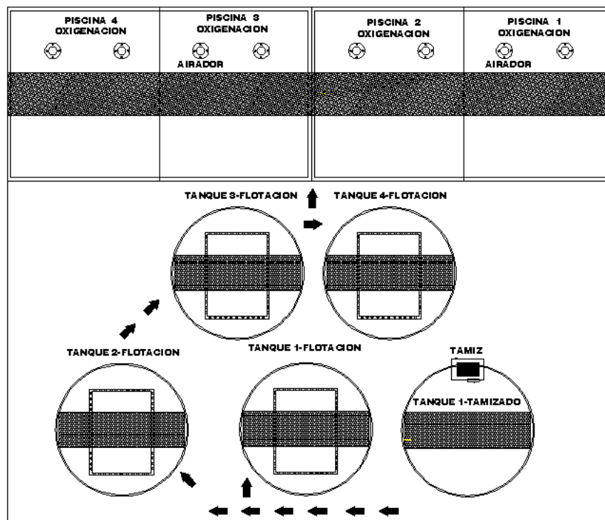
FIGURA 4.14. Alternativa 3- Área de tratamiento de aguas residuales.
