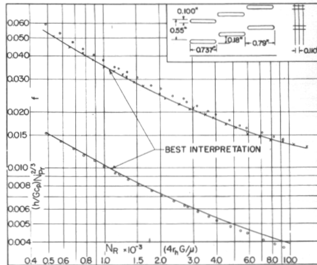
Figura 2.3. Coeficiente de transferencia y Factor de fricción
