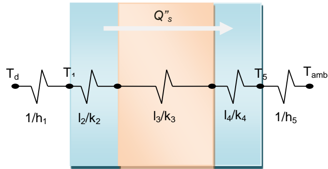
Figura D.1. Circuito Térmico del Flujo de Calor
