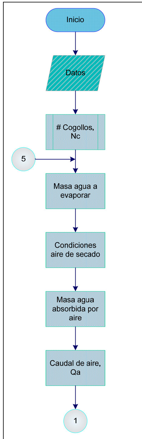
Figura 4.1. Flujograma del Diseño Térmico del Sistema
