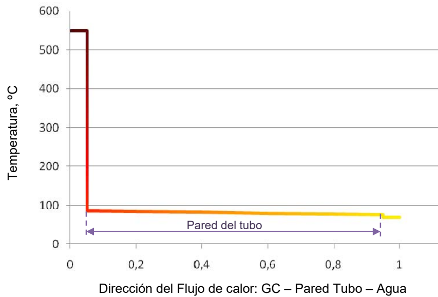
Figura 3.7. Flujo de Calor en Tubos del IC
