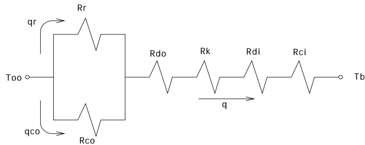
Figura 3.6. Circuito Térmico
