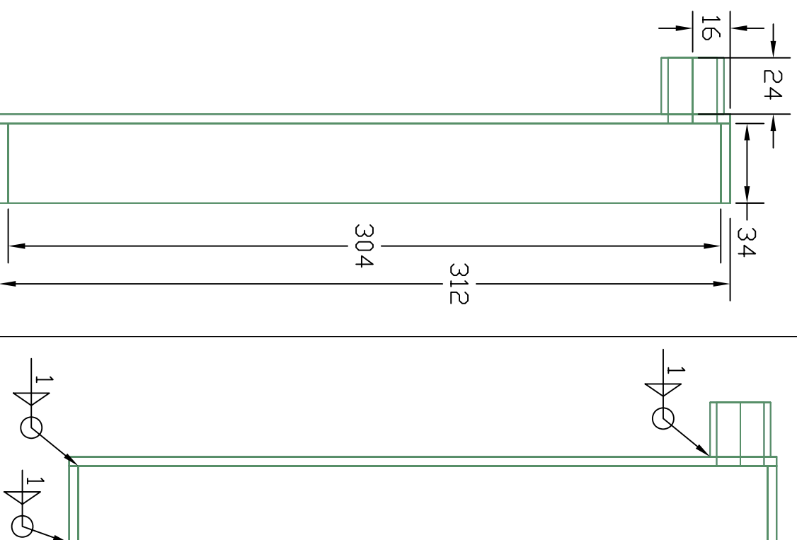
VISTA LATERAL DERECHA Tapa Espejo de Salida
