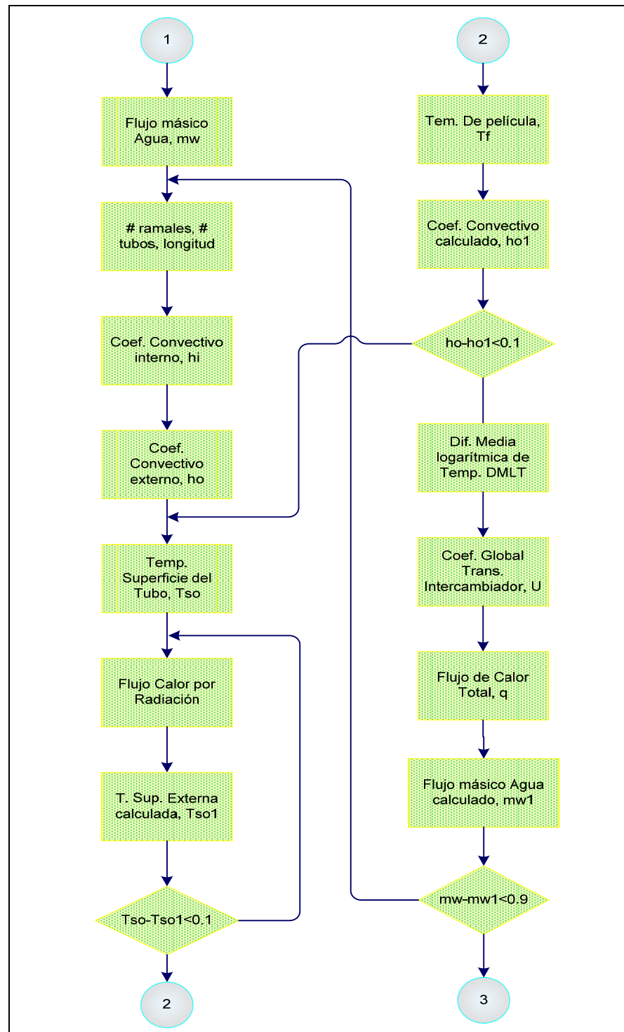
Figura 4.2. Flujograma del Diseño Térmico del Sistema
