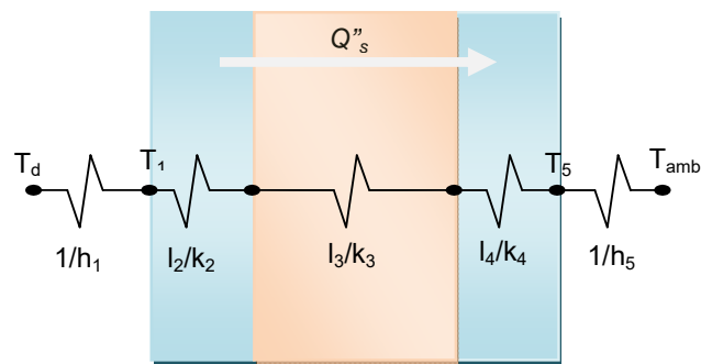
Figura 2.1. Circuito Térmico del Flujo de Calor
