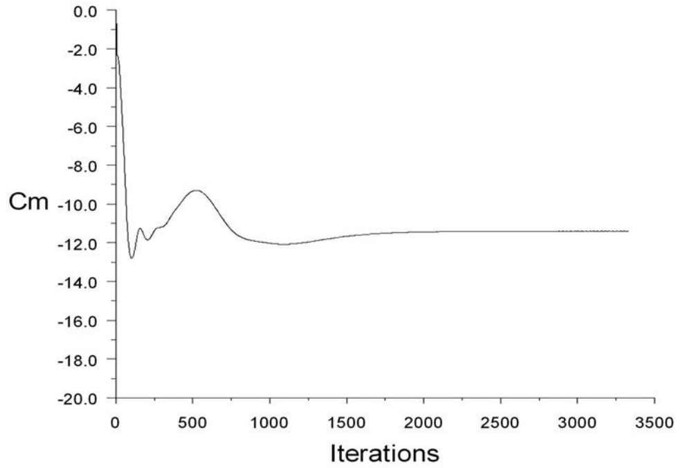
FIGURA 3.27 COEFICIENTE DE MOMENTO CASO 2
