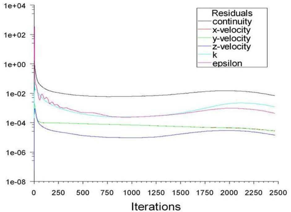
FIGURA 3.30 RESIDUOS CASO 4
