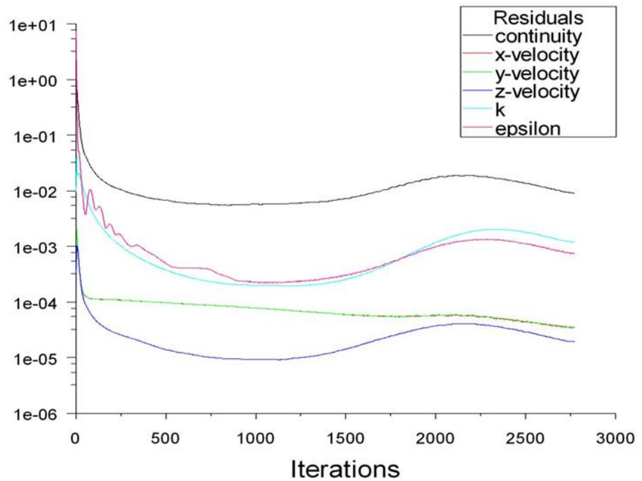
FIGURA 3.28 RESIDUOS CASO 3
