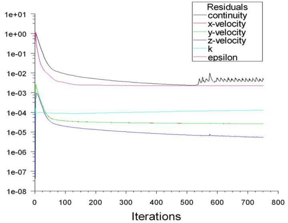
FIGURA 5.8 RESIDUOS CASO 1 MEJORADO
