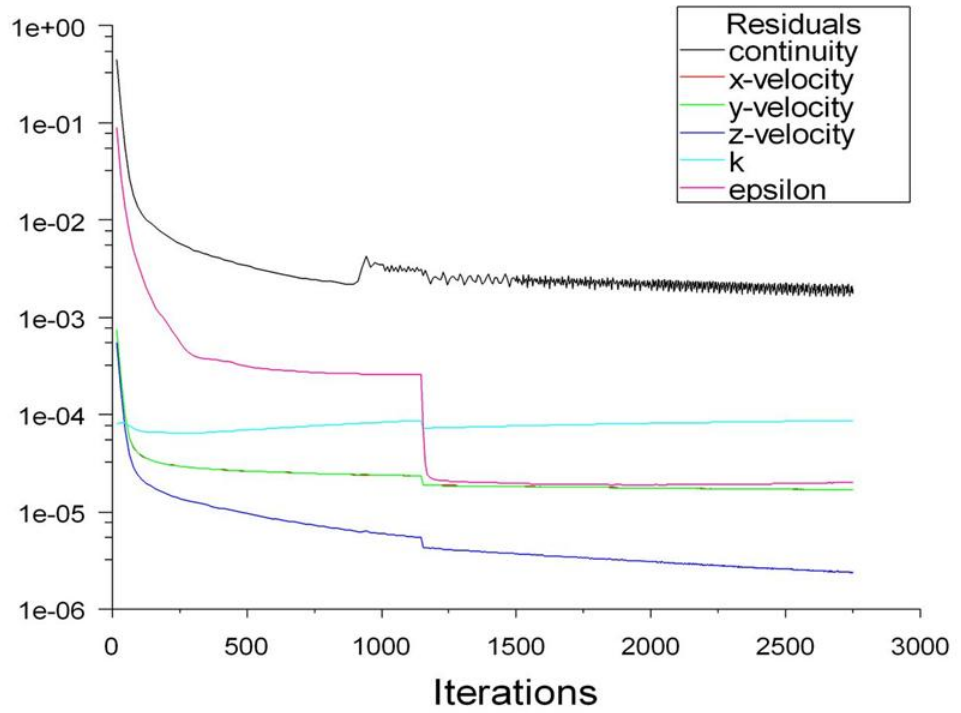
FIGURA 5.16 RESIDUOS CASO 5 MEJORADO
