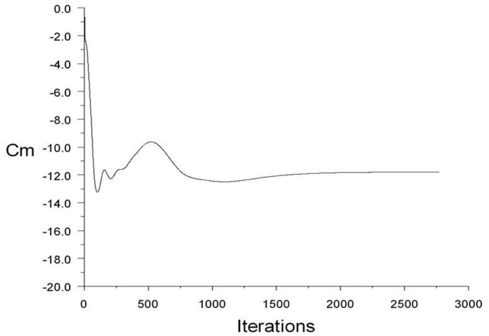
FIGURA 3.29 COEFICIENTE DE MOMENTO CASO 3
