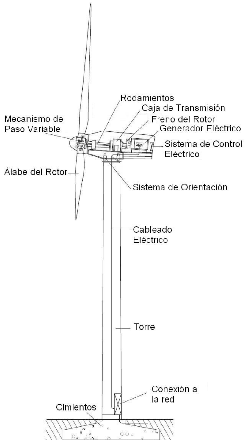
FIGURA 2.4 GENERADOR EÓLICO DE EJE HORIZONTAL
