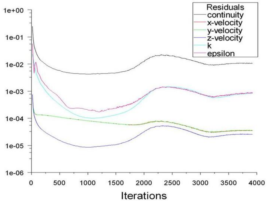
FIGURA 3.32 RESIDUOS CASO 5
