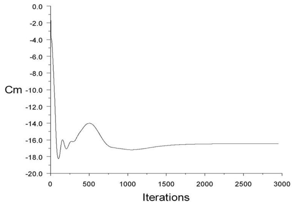
FIGURA 3.23 GRÁFICO DE COEFICIENTE DE MOMENTO
