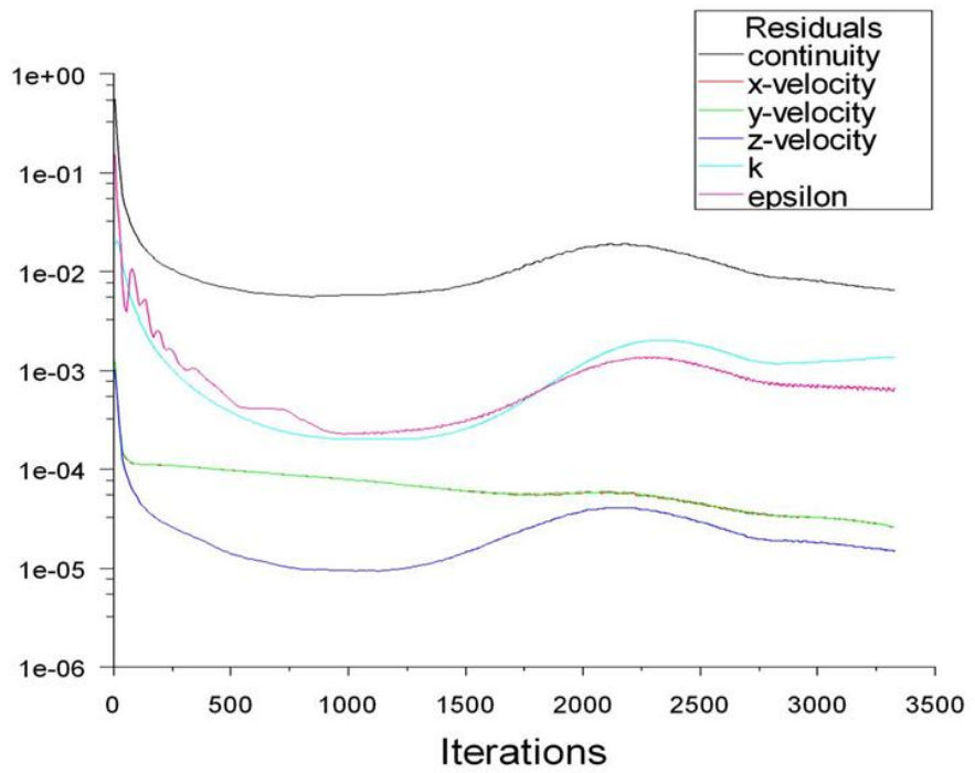
FIGURA 3.26 RESIDUOS CASO 2
