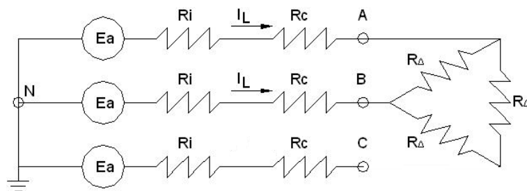
FIGURA 5.2 CIRCUITO ELECTRICO PARA LOS CASOS 5 Y 6
