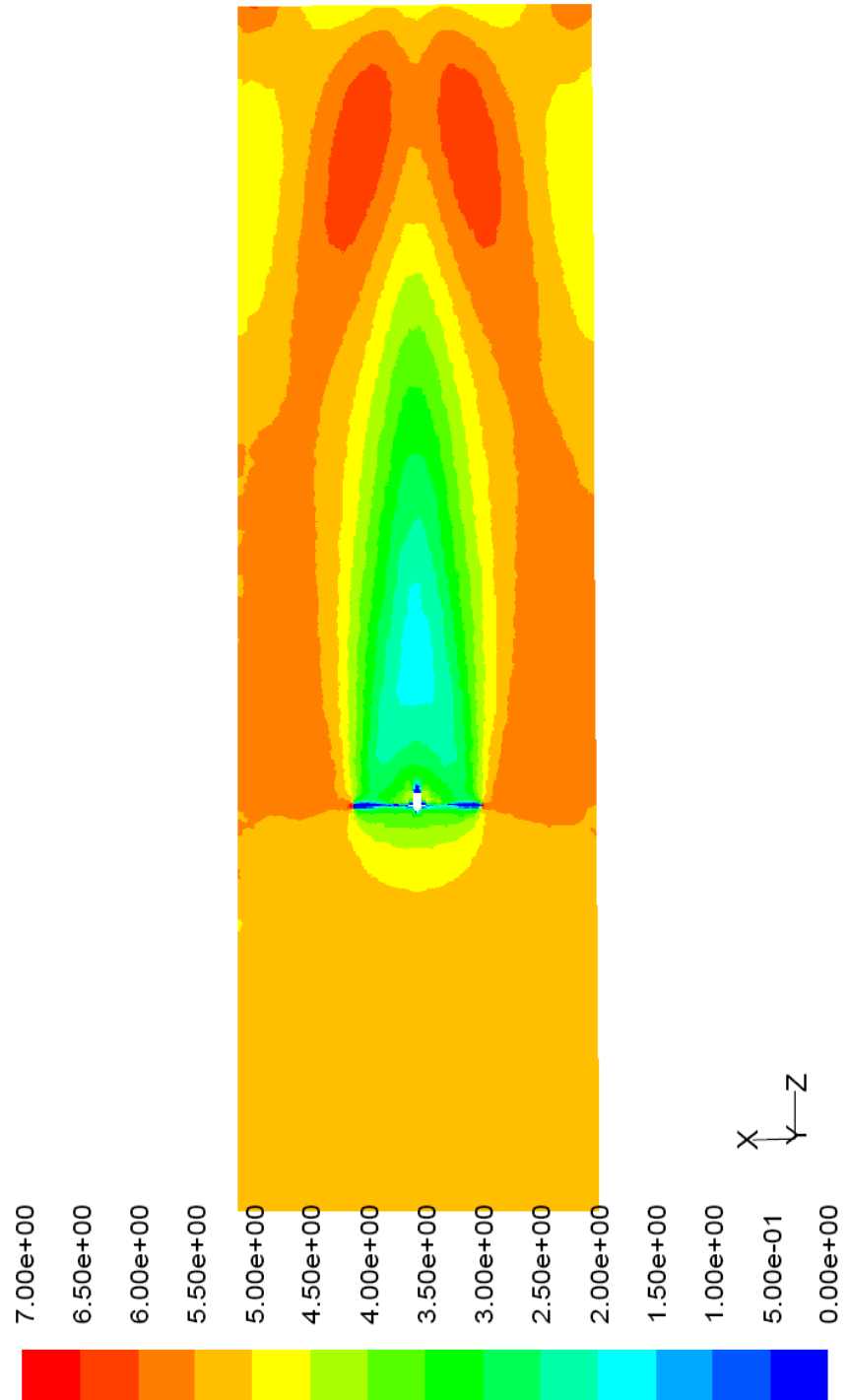
FIGURA 3.41 CONTORNO DE VELOCIDAD Z CASO 6
