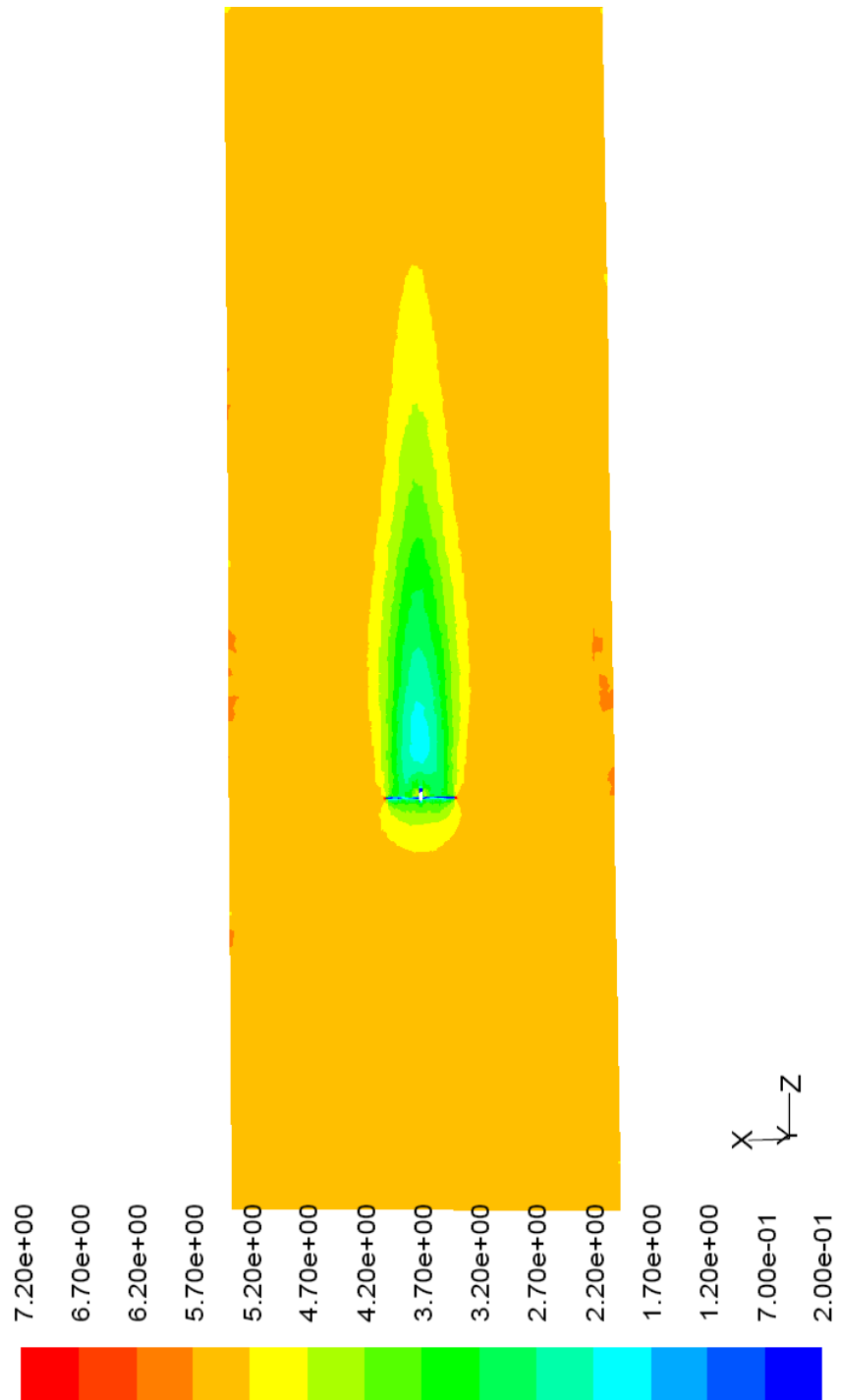
FIGURA 5.23 CONTORNO DE VELOCIDAD Z CASO 4 MEJORADO
