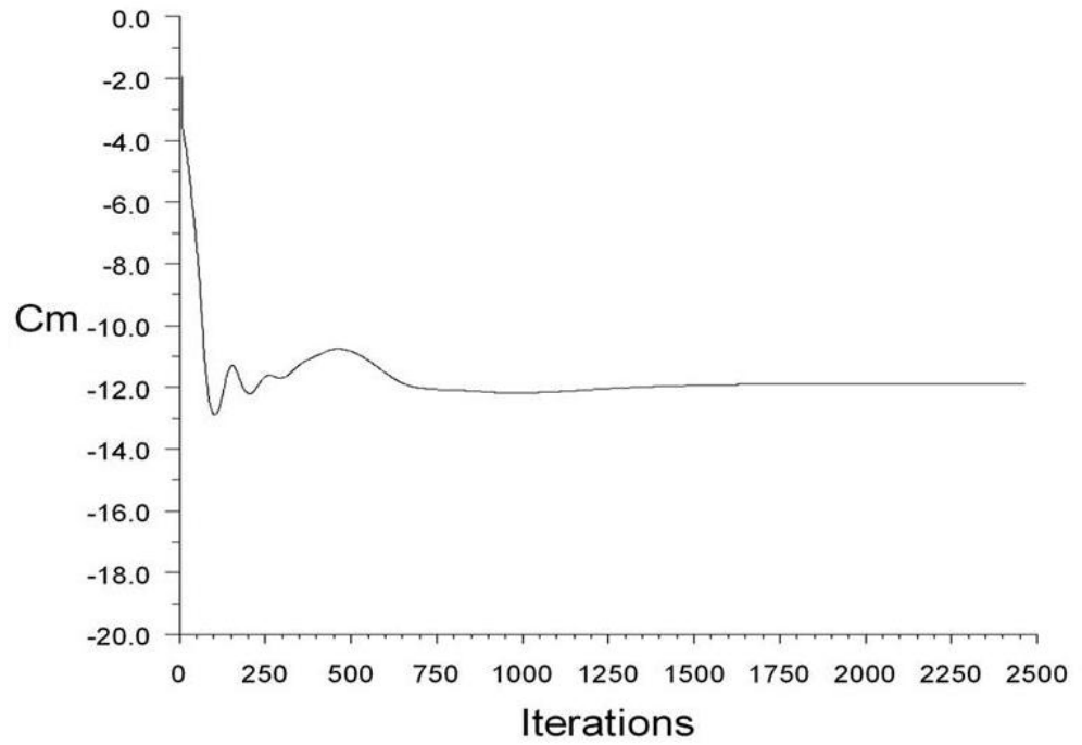
FIGURA 3.31 COEFICIENTE DE MOMENTO CASO 4
