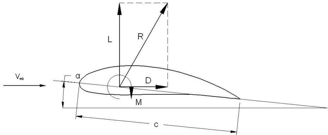
FIGURA 2.2 FUERZAS AERODINÁMICAS
