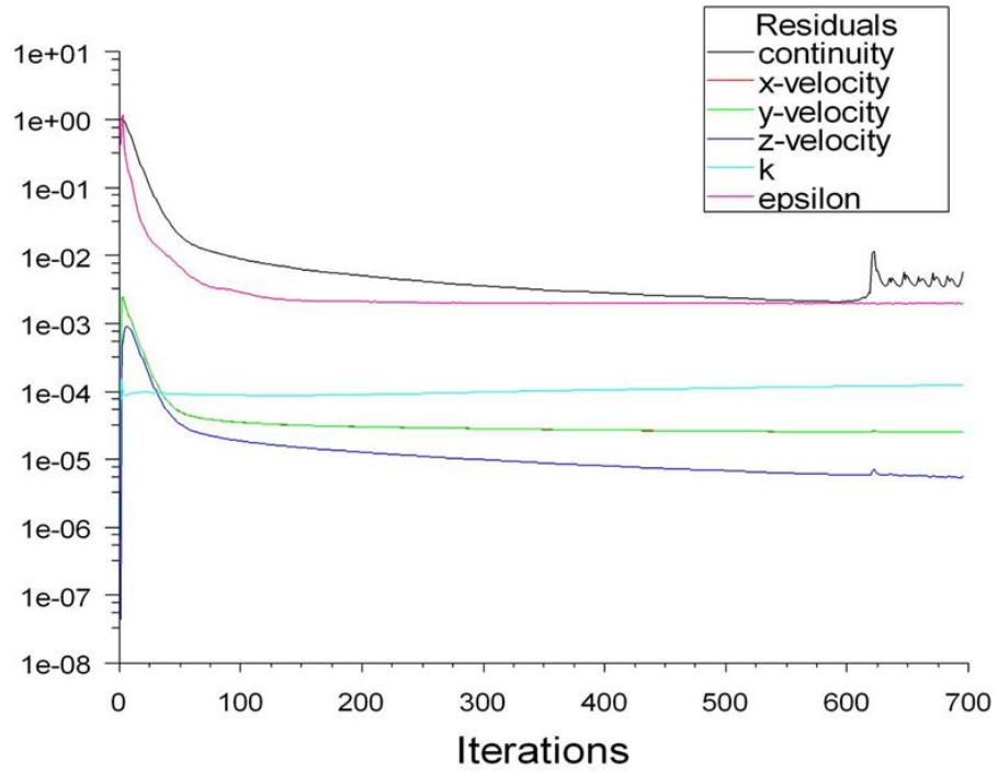
FIGURA 5.10 RESIDUOS CASO 2 MEJORADO
