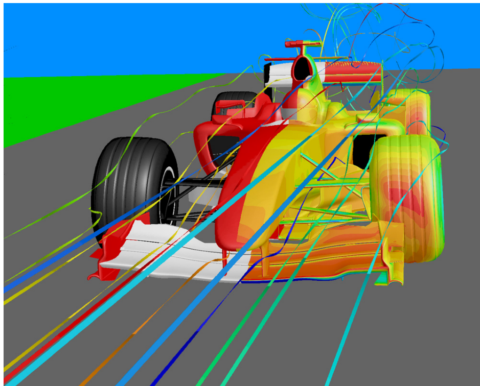
FIGURA 2.10 RESULTADO DE POST-PROCESAMIENTO DE UN PROGRAMA DE CFD COMERCIAL. Cortesía de Fluent Inc.
