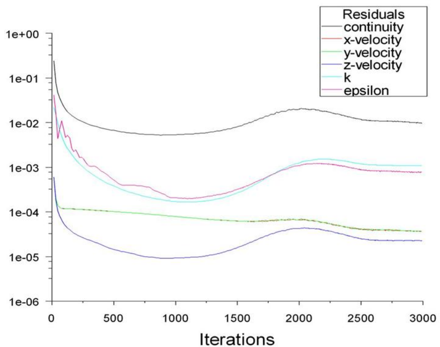
FIGURA 3.24 RESIDUOS CASO 1
