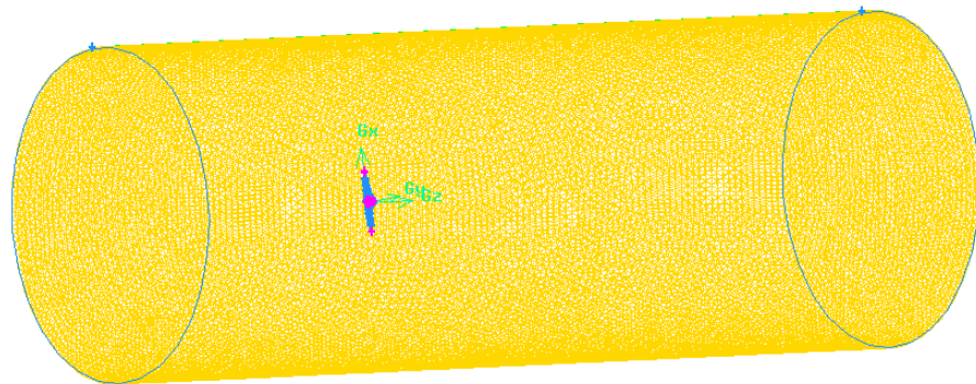
FIGURA 5.5 MALLADO TRIDIMENSIONAL DEL MODELO CFD MEJORADO
