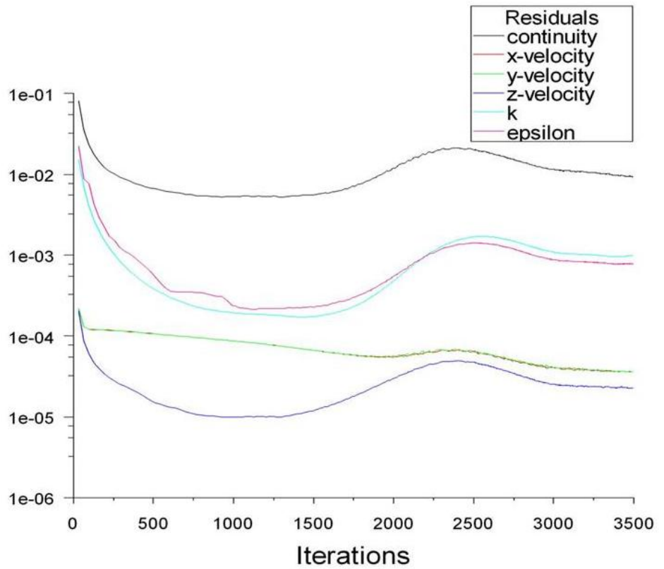
FIGURA 3.34 RESIDUOS CASO 6
