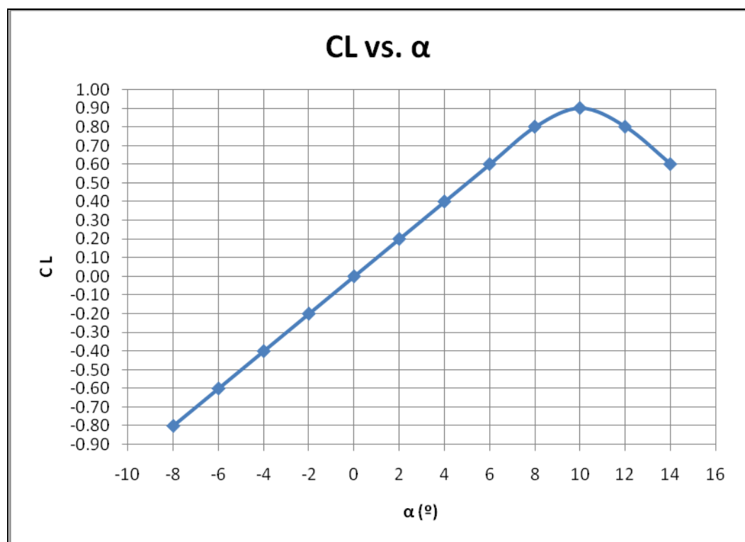
FIGURA 2.3 COEFICIENTE DE SUSTENTACIÓN VERSUS ÁNGULO DE ATAQUE PARA UN PERFIL NACA 0006 Y Re = 3.0 \times 10^6
