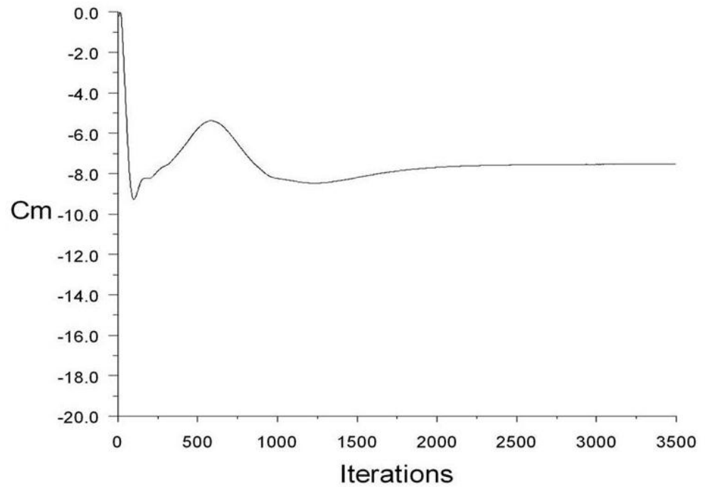
FIGURA 3.35 COEFICIENTE DE MOMENTO CASO 6
