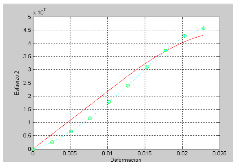
FIGURA 4.41 MODELAMIENTO A LOS 7 DÍAS/25% DE LIMOLITA
