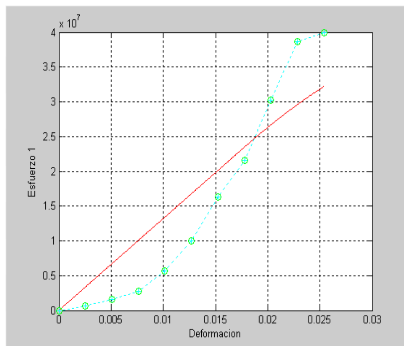
FIGURA 4.44 MODELAMIENTO A LOS 28 DÍAS/25% DE LIMOLITA
