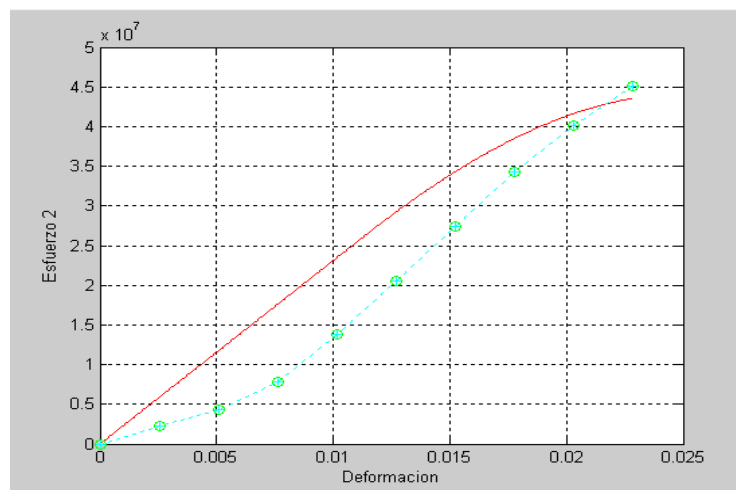
FIGURA 4.45 MODELAMIENTO A LOS 4 DÍAS/27.5%
