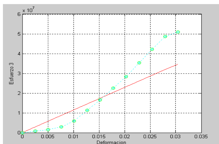
FIGURA 4.46 MODELAMIENTO A LOS 11 DÍAS/27.5%
