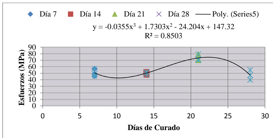
FIGURA 4.18. AJUSTE POLINOMIAL DE 3 º ORDEN DE RESISTENCIAS AL 25% DE LIMOLITA
