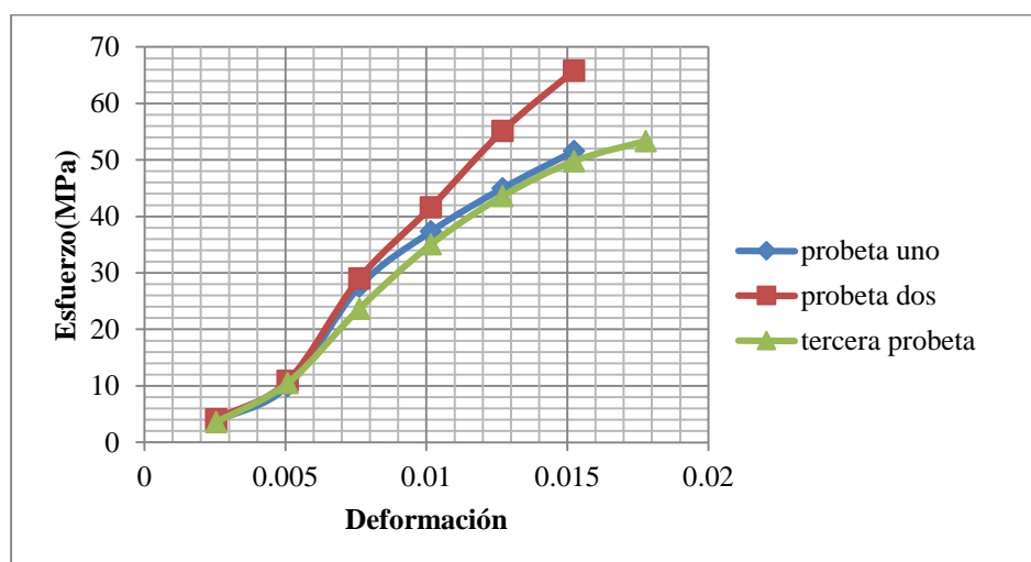
FIGURA 4.8. ESFUERZO VS DEFORMACIÓN/25 DÍAS
