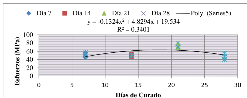
FIGURA 4.17. AJUSTE POLINOMIAL DE 2º ORDEN DE RESISTENCIAS AL 25% DE LIMOLITA
