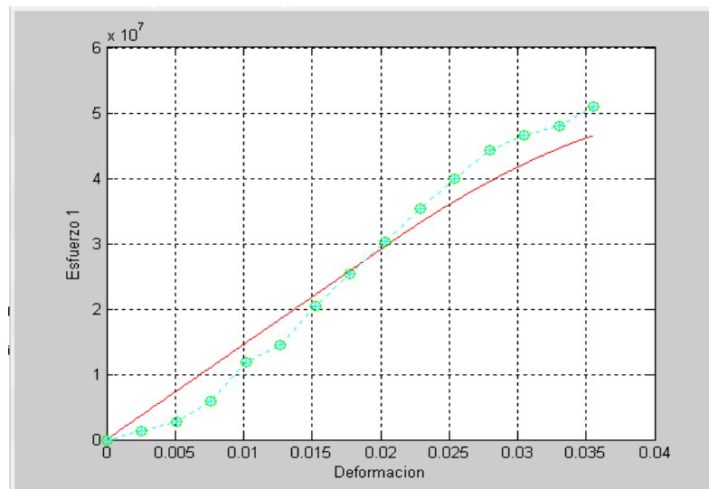
FIGURA 4.42 MODELAMIENTO A LOS 14 DÍAS/25% DE LIMOLITA
