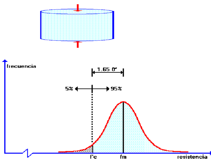
FIG3.15 DISTRIBUCION NORMALIZADA DE LOS ENSAYOS DE ROTURA
