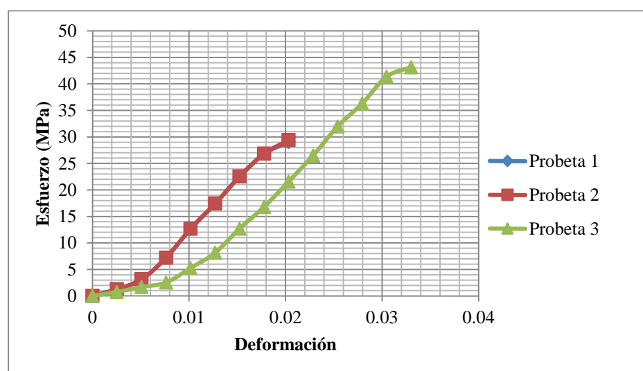
FIGURA 4.7. ESFUERZO VS DEFORMACIÓN/18 DÍAS
