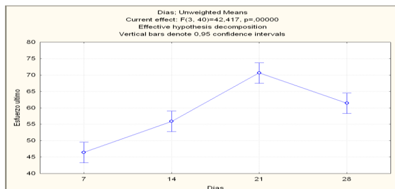
FIGURA 4.28. DÍAS VS ESFUERZOS DE RUPTURA (ANOVA)
