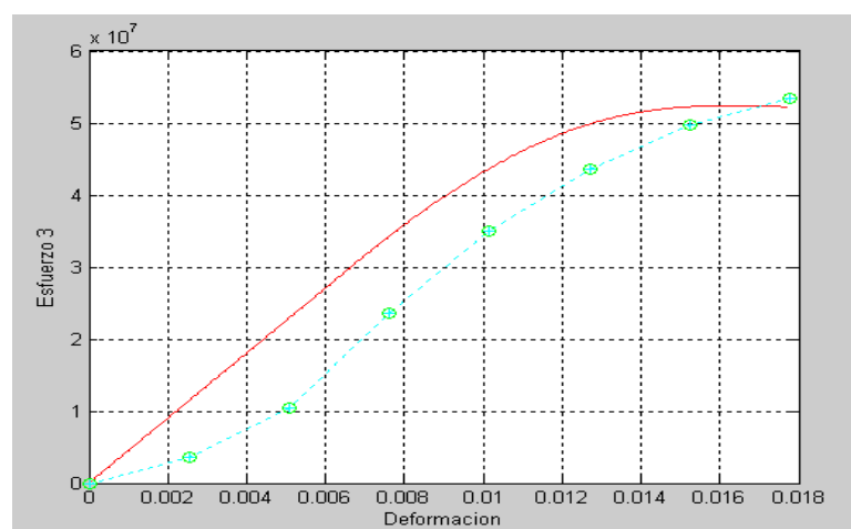
FIGURA 4.48 MODELAMIENTO A LOS 25 DÍAS/27.5%
