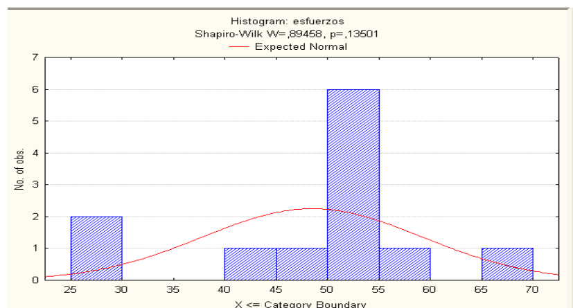
FIGURA 4.21. HISTOGRAMA DE ESFUERZOS AL 27.5% DE LIMOLITA
