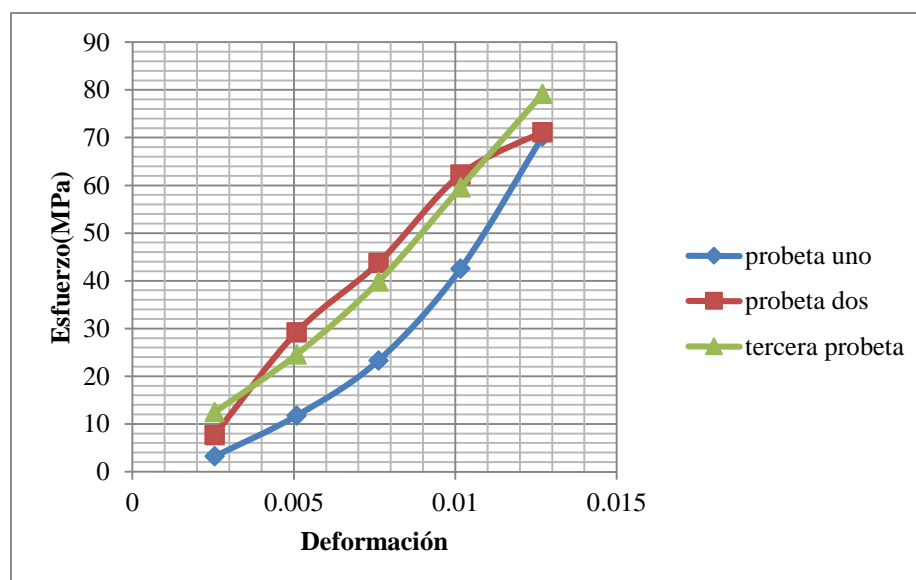
FIGURA 4.3. ESFUERZO VS DEFORMACIÓN/21DÍAS
