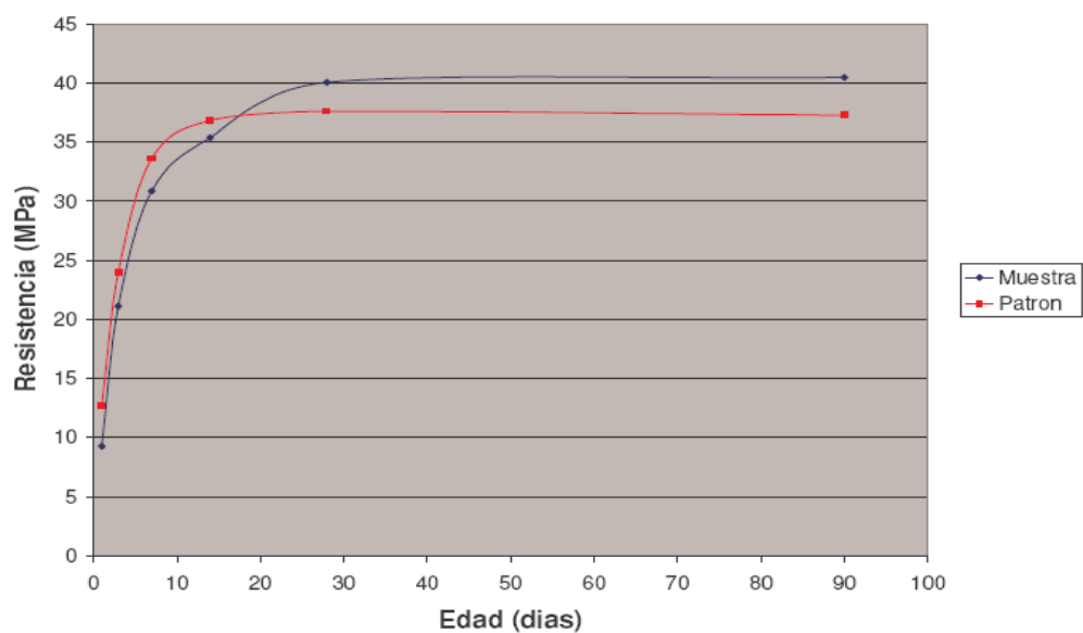
FIGURA 2.4. COMPARACION DE RESISTENCIAS MUESTRA/PATRON
