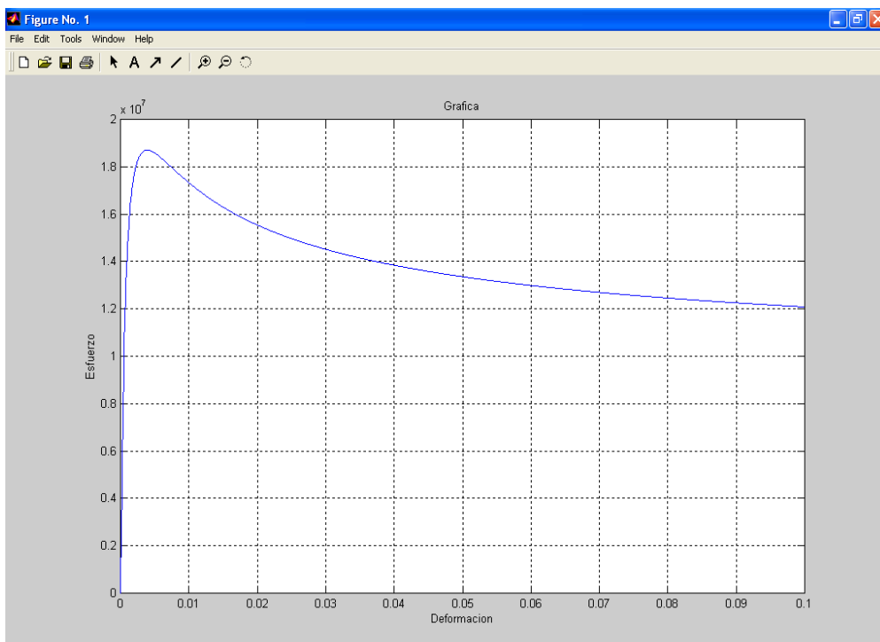
FIGURA 3.17. GRÁFICA ESFUERZO VS DEFORMACIÓN DEL MODELO
