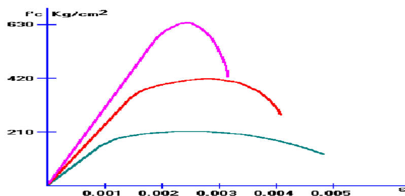
FIG 3.16 DISTRIBUCION DE LAS RESISTENCIAS
