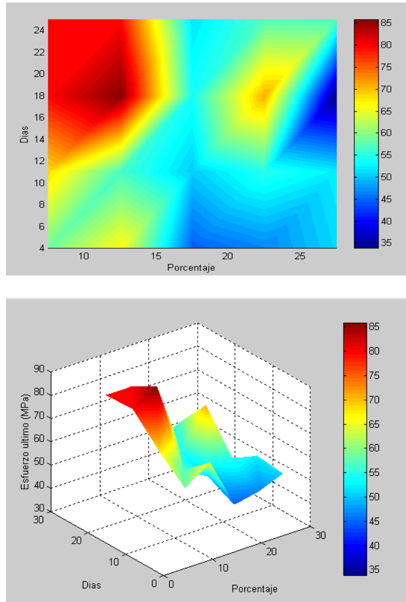
FIGURA 4.50 GRÁFICA GLOBAL DE LAS MEDIAS, ESFUERZOS ÚLTIMOS, DÍAS Y PORCENTAJES DE ADITIVOS (VALIDACIÓN)
