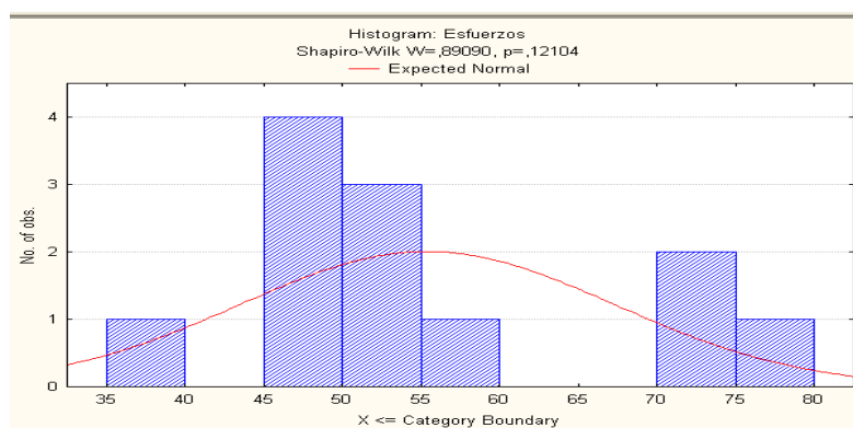
FIGURA 4.13. HISTOGRAMA DE ESFUERZOS AL 25% DE LIMOLITA
