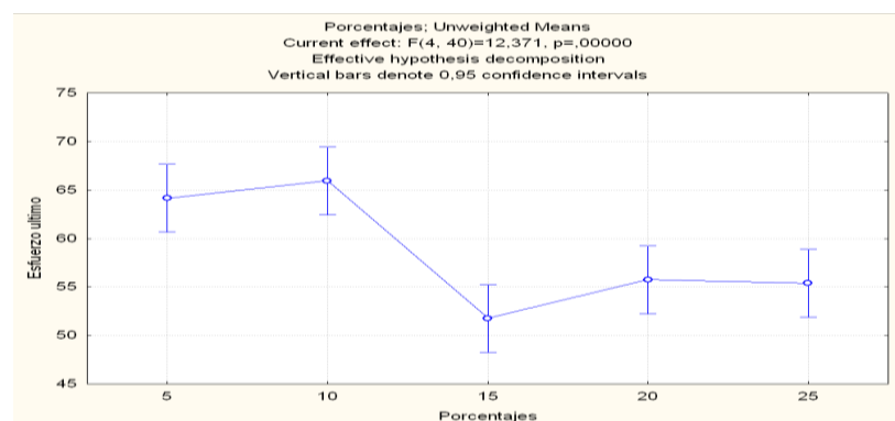
FIGURA 4.30. PORCENTAJES VS ESFUERZOS DE RUPTURA EN ANOVA
