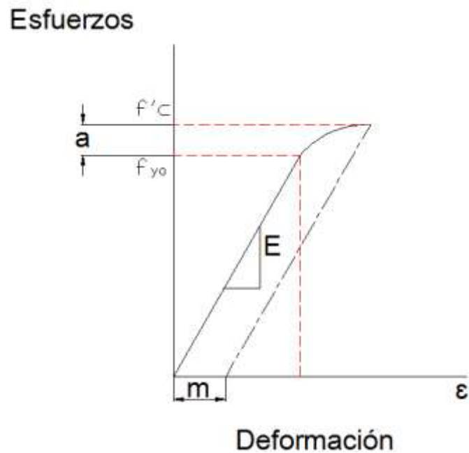
Figura 2.5. Esfuerzo-Deformación
