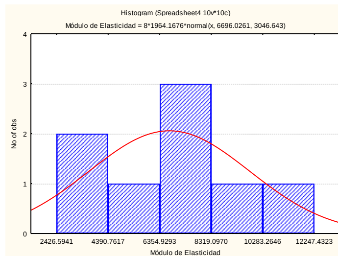
Figura 3.4 Histogramas de los módulos de elasticidad Adición: 15% Días de curado: 28
