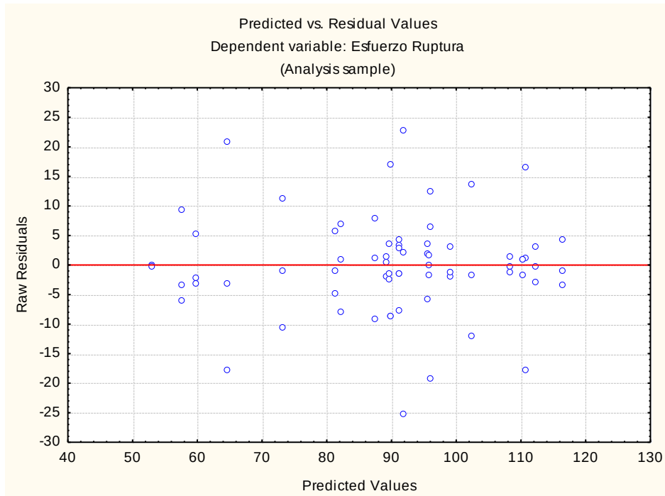
Figura 4.16. Valores predictivos y residuales
