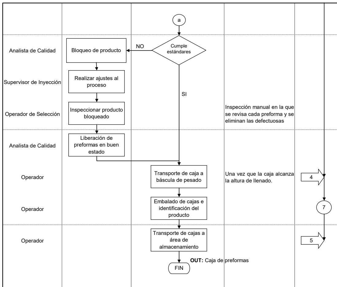
FIGURA 1.5 DIAGRAMA DE FLUJO DEL PROCESO DE ELABORACIÓN DE PREFORMAS
