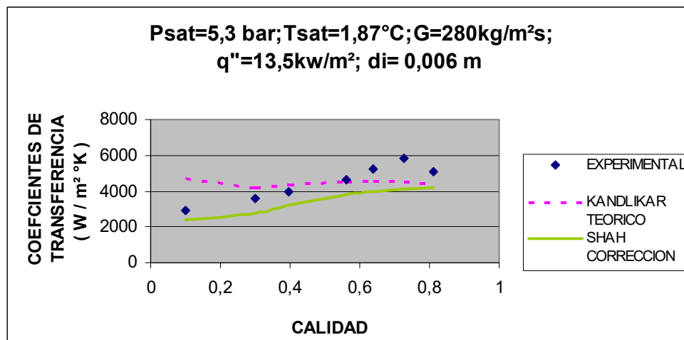
FIGURA 2.29 EVALUACION DE MODELOS CORREGIDOS DE SHAH Y KANDLIKAR A T_{sat} = 1.87^{\circ}\text{C} PARA R22
