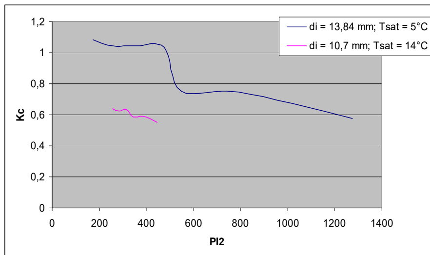
FIGURA 2.42 VALORES DE PI_2 Y K_c PARA CORRELACIÓN DE KANDLIKAR A di = 13.84\text{mm} ; T_{sat} = 5^\circ\text{C} Y di = 10.7\text{mm} ; T_{sat} = 14^\circ\text{C}
