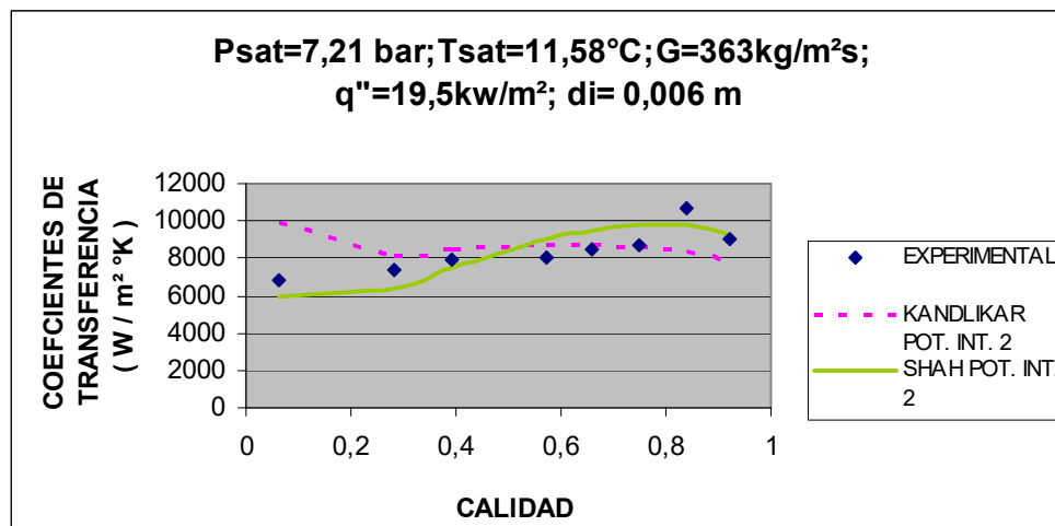
FIGURA 2.31 EVALUACION DE MODELOS CORREGIDOS DE SHAH Y KANDLIKAR A T_{sat} = 11.58^{\circ}\text{C} PARA R22
