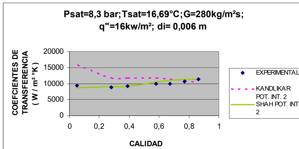
FIGURA 2.33 EVALUACION DE MODELOS CORREGIDOS DE SHAH Y KANDLIKAR A T_{sat} = 16.69^{\circ}\text{C} PARA R22
