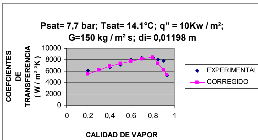
FIGURA 2.52 EVALUACION DE MODELO CORREGIDO DE WOLVERINE A G = 150 \text{ Kg} / \text{m}^2 \text{ s} PARA R22
