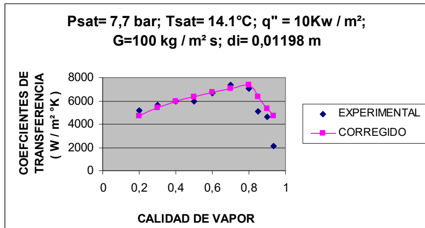
FIGURA 2.51 EVALUACION DE MODELO CORREGIDO DE WOLVERINE A G = 100 \text{ Kg} / \text{m}^2 \text{ s} PARA R22
