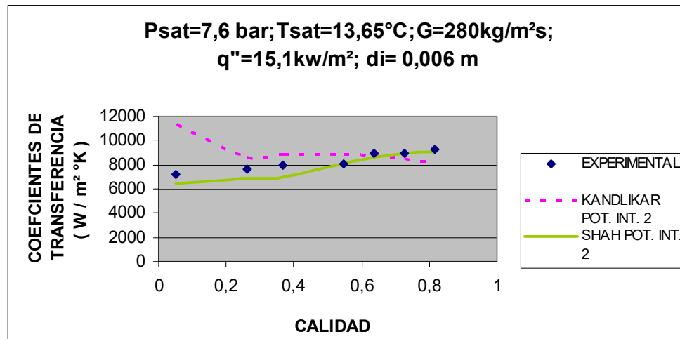
FIGURA 2.32 EVALUACION DE MODELOS CORREGIDOS DE SHAH Y KANDLIKAR A T_{sat} = 13.65^{\circ}\text{C} PARA R22
