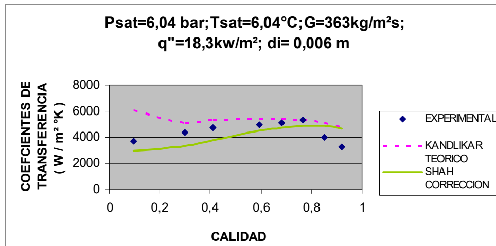
FIGURA 2.30 EVALUACION DE MODELOS CORREGIDOS DE SHAH Y KANDLIKAR A T_{sat} = 6.04^{\circ}\text{C} PARA R22
