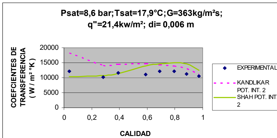
FIGURA 2.34 EVALUACION DE MODELOS CORREGIDOS DE SHAH Y KANDLIKAR A T_{sat} = 17.9^{\circ}\text{C} PARA R22
