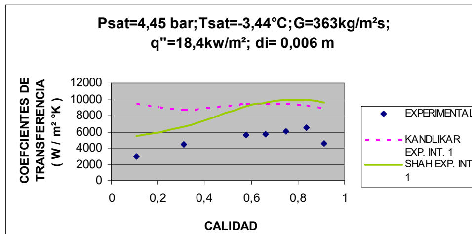
FIGURA 2.27 EVALUACION DE MODELOS CORREGIDOS DE SHAH Y KANDLIKAR A T_{sat} = -3.44^{\circ}\text{C} PARA R22
