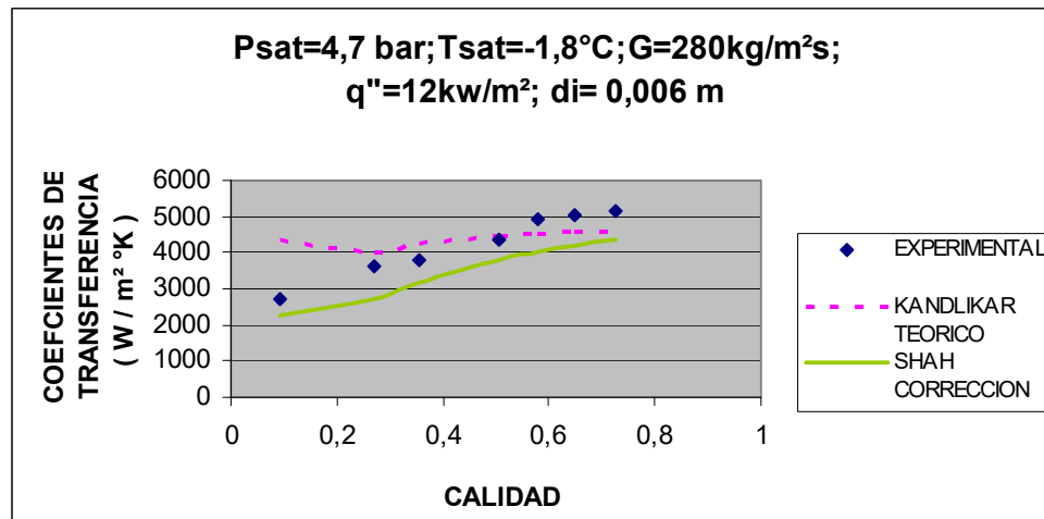
FIGURA 2.28 EVALUACION DE MODELOS CORREGIDOS DE SHAH Y KANDLIKAR A T_{sat} = -1.8^{\circ}\text{C} PARA R22
