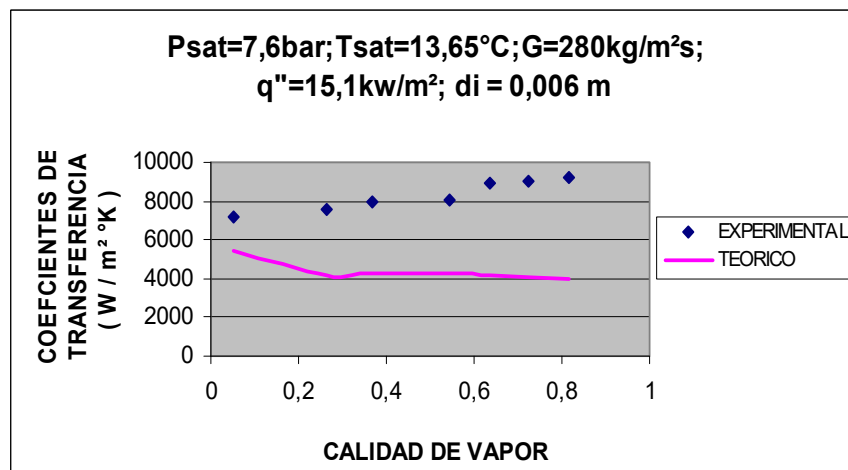
FIGURA 2.2.22 EVALUACION DE CORRELACION DE KANDLIKAR A
