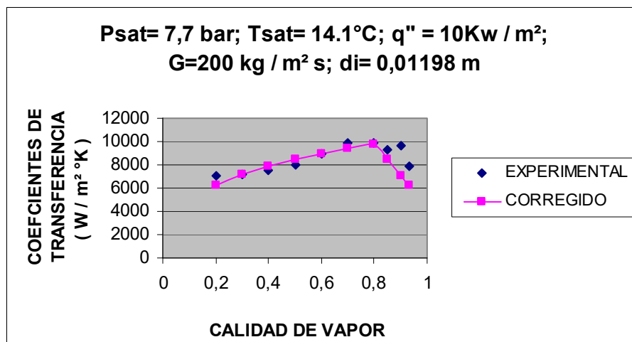
FIGURA 2.53 EVALUACION DE MODELO CORREGIDO DE WOLVERINE A G = 200 \text{ Kg} / \text{m}^2 \text{ s} PARA R22
