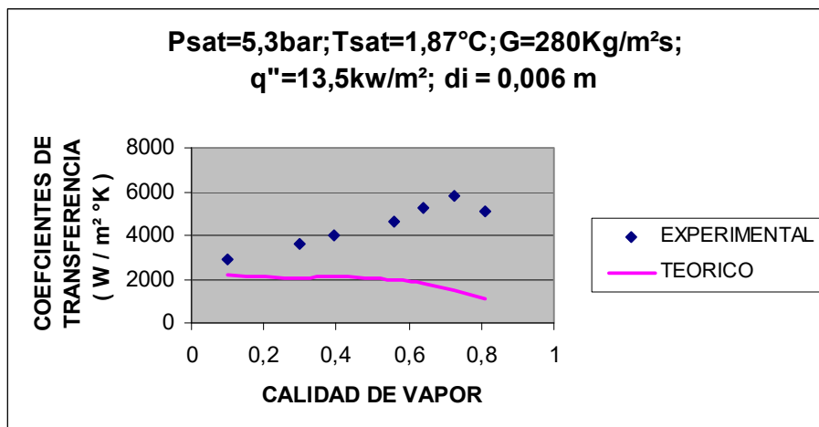
FIGURA 2.8 EVALUACION DE CORRELACION DE SHAH A T_{sat} = 1.87\text{ }^{\circ}\text{C} PARA R22
