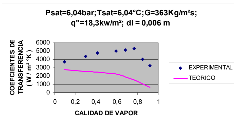
FIGURA 2.9 EVALUACION DE CORRELACION DE SHAH A T_{sat} = 6.04\text{ }^{\circ}\text{C} PARA R22
