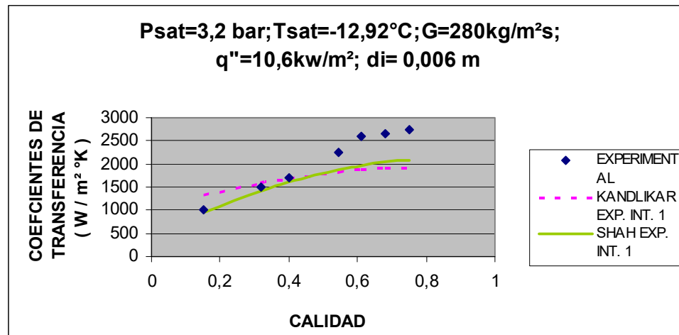
FIGURA 2.26 EVALUACION DE MODELOS CORREGIDOS DE SHAH Y KANDLIKAR A T_{sat} = -12.92^{\circ}\text{C} PARA R22
