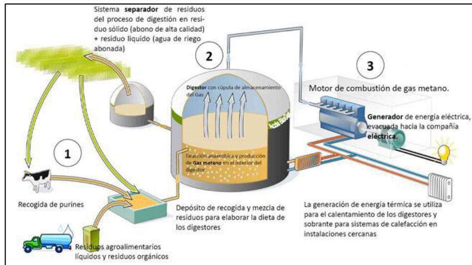
Figura 30. Esquema de una planta de aprovechamiento de biogás (Ecoespacios, 2012).
