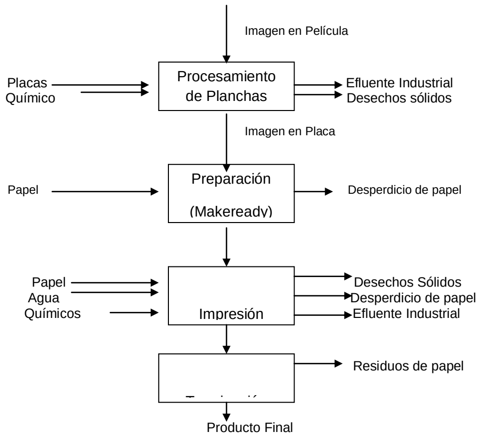
FIGURA 3.1 DIAGRAMA DEL PROCESO OFFSET
